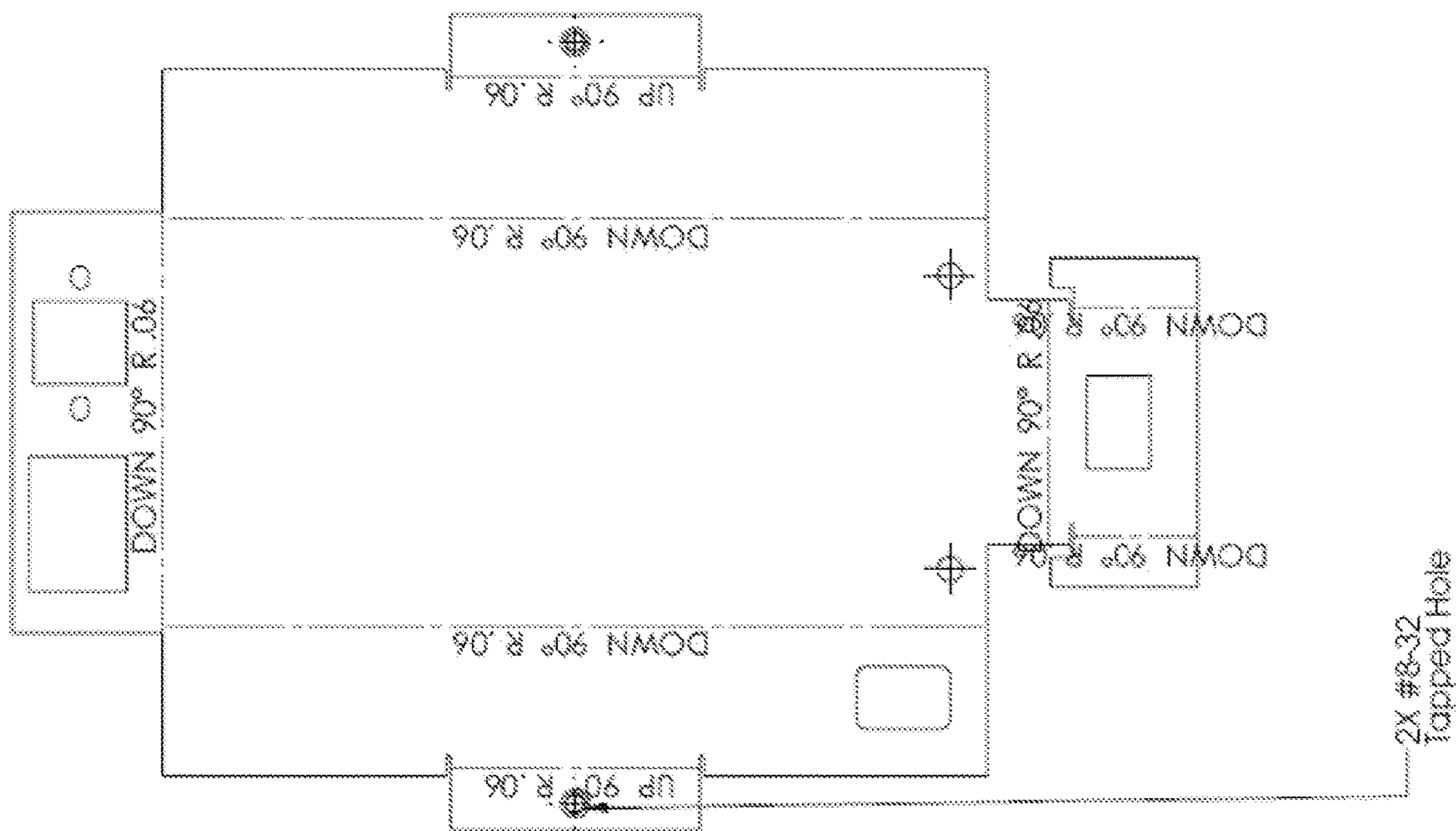
FIG. 15B
