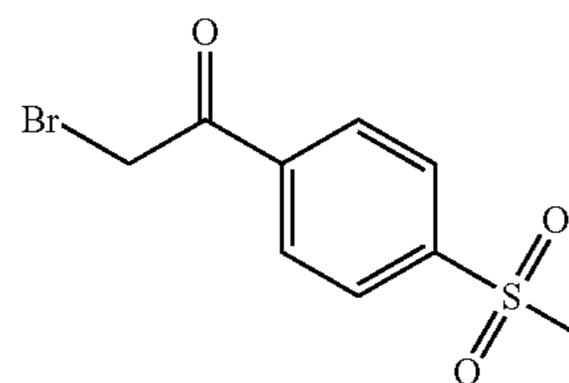
2-Bromo-1-[4-(methylsulfonyl)phenyl]-1-ethanone
