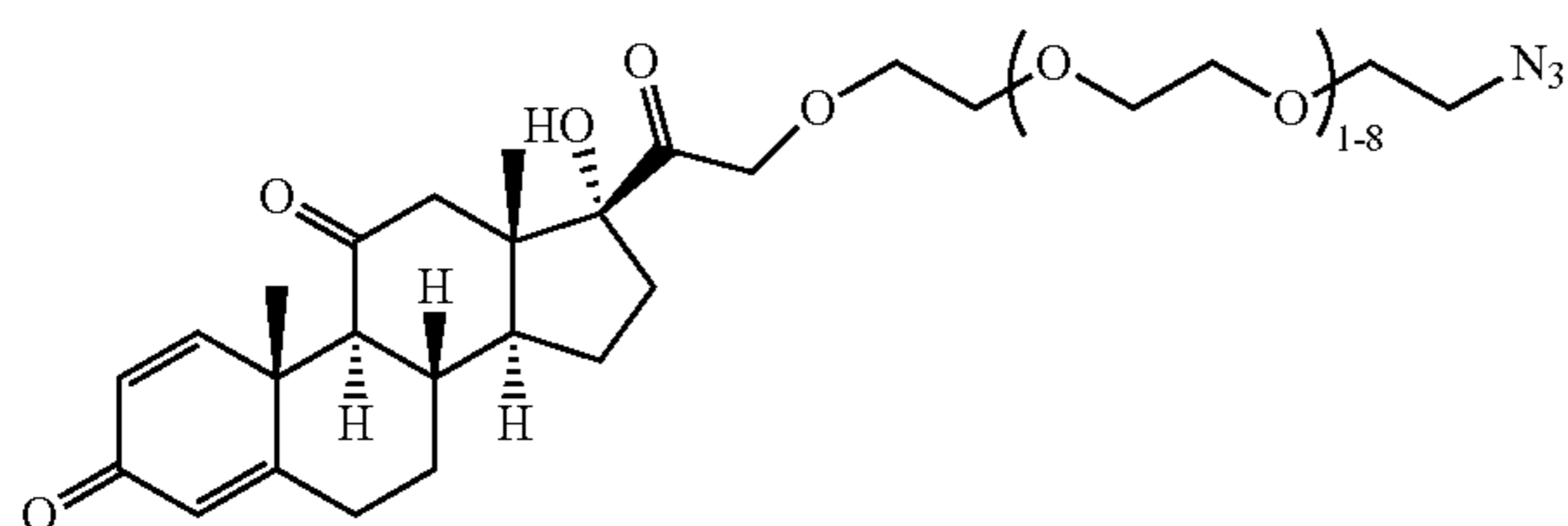
Prednisolone analogue
