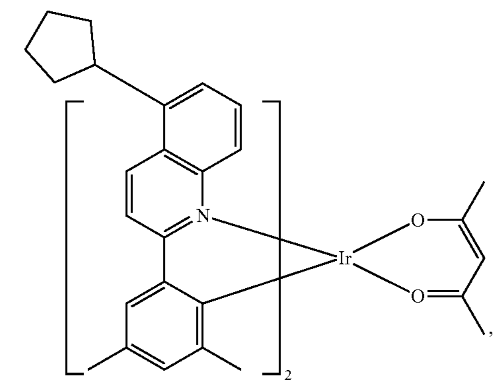
Compound E17
