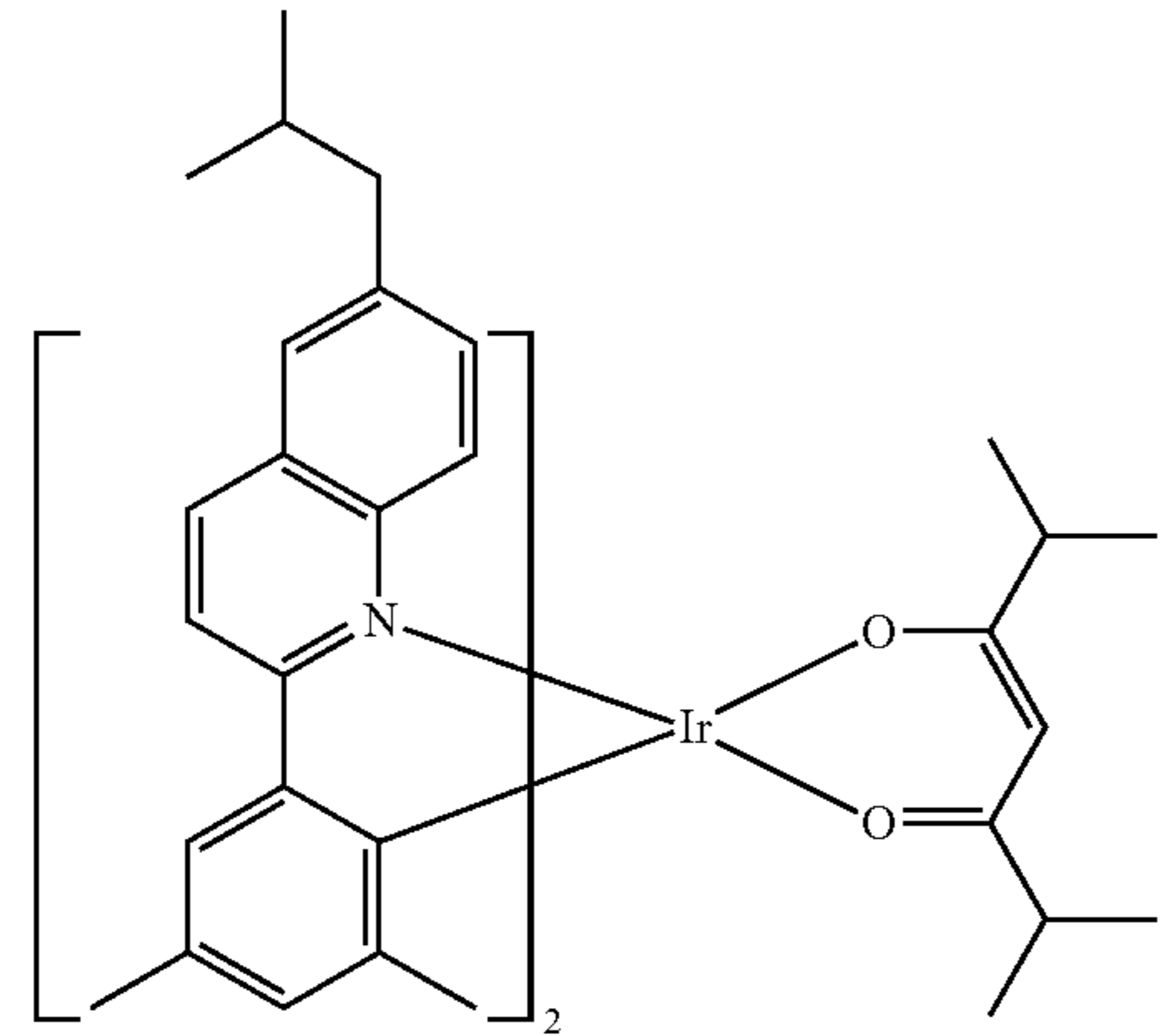
Compound E15
