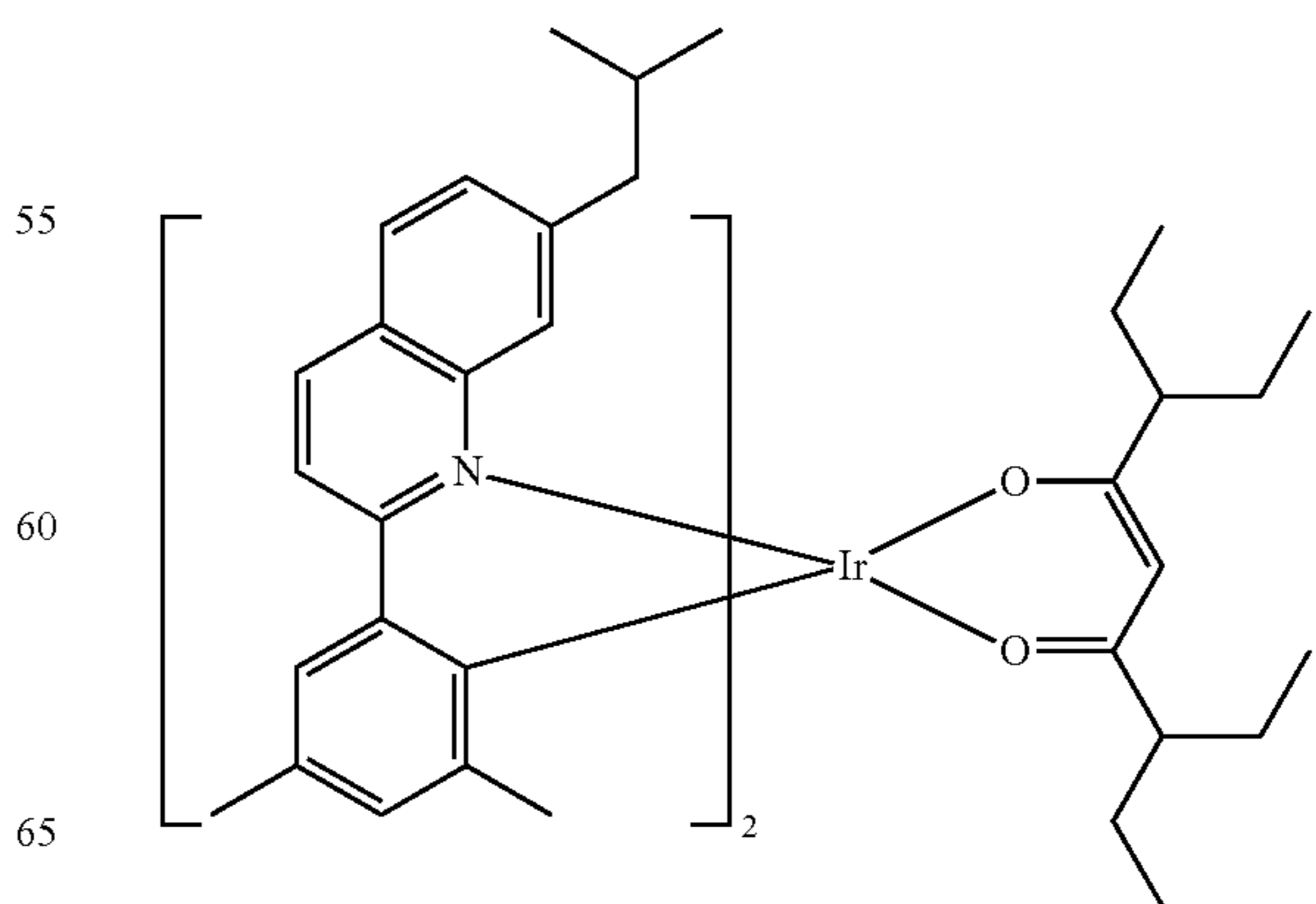
Compound E10
