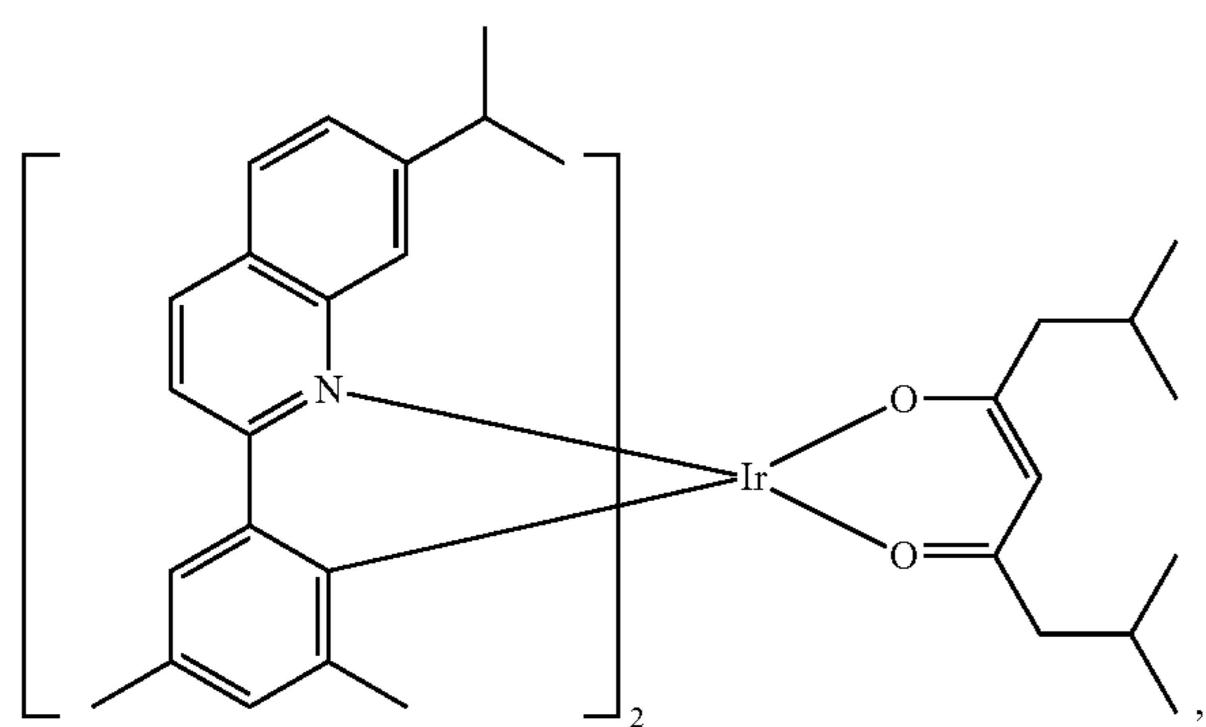
Compound E36
