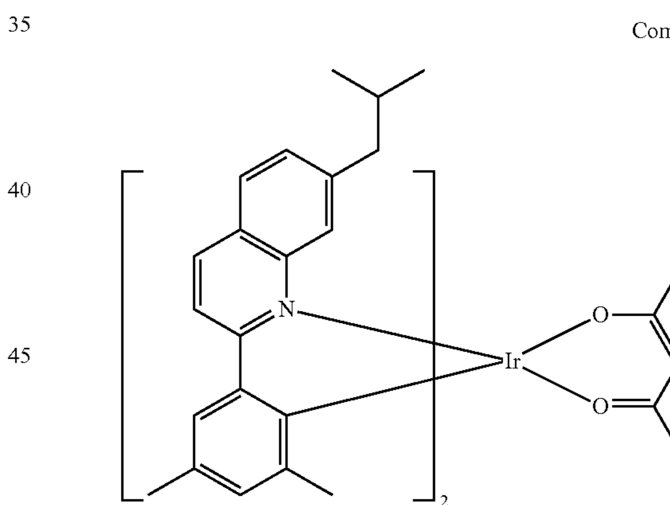
Compound E10
