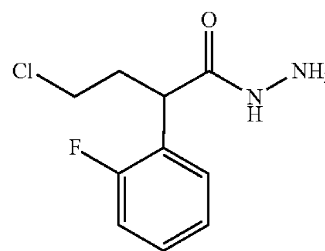
Step 4: 4-chloro-2-(2-fluorophenyl)butanehydrazide
