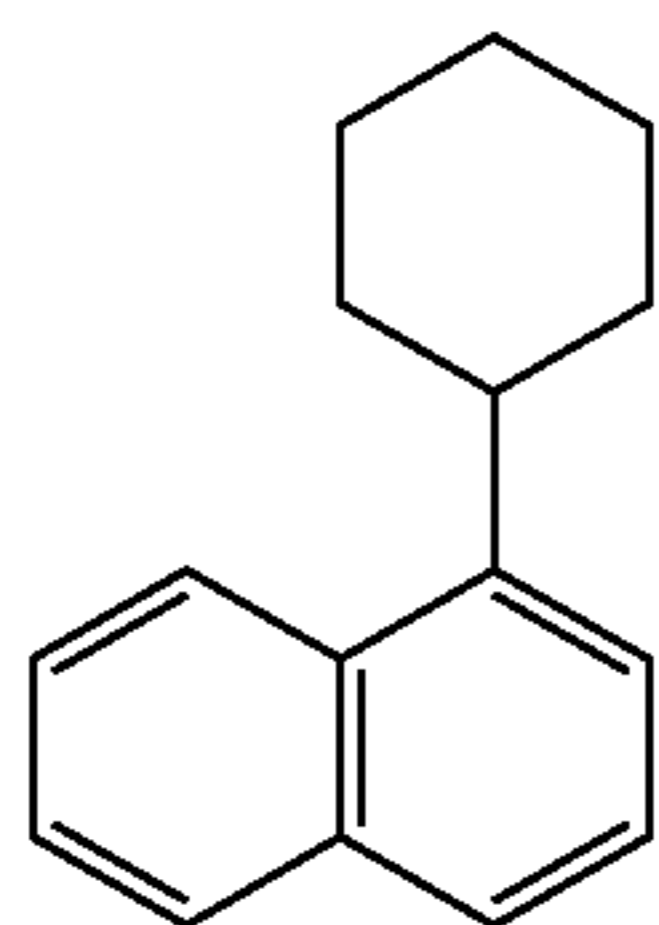
CAS 3042-69-1 Cyclohexylnaphthalene
