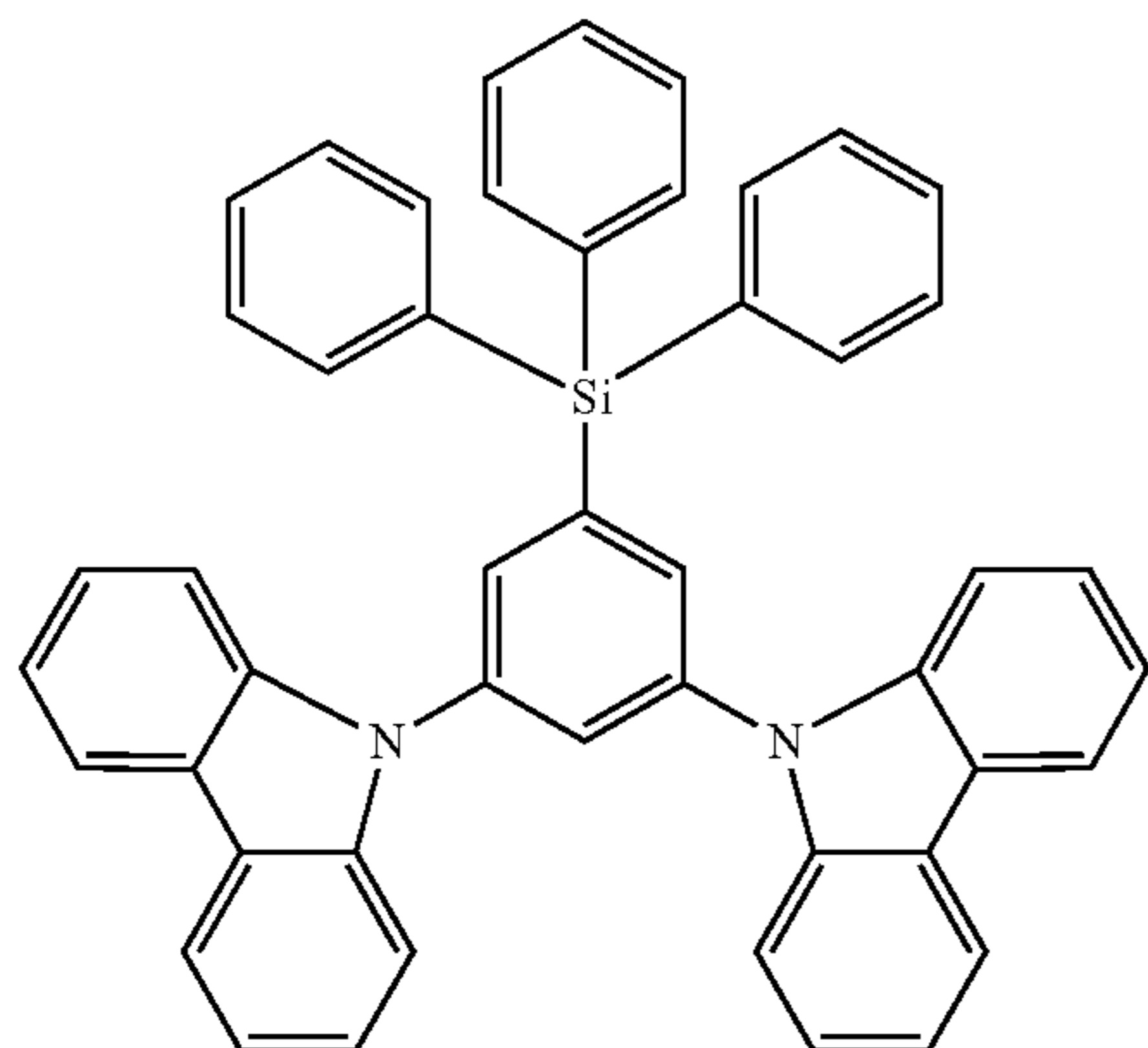
SimCP
