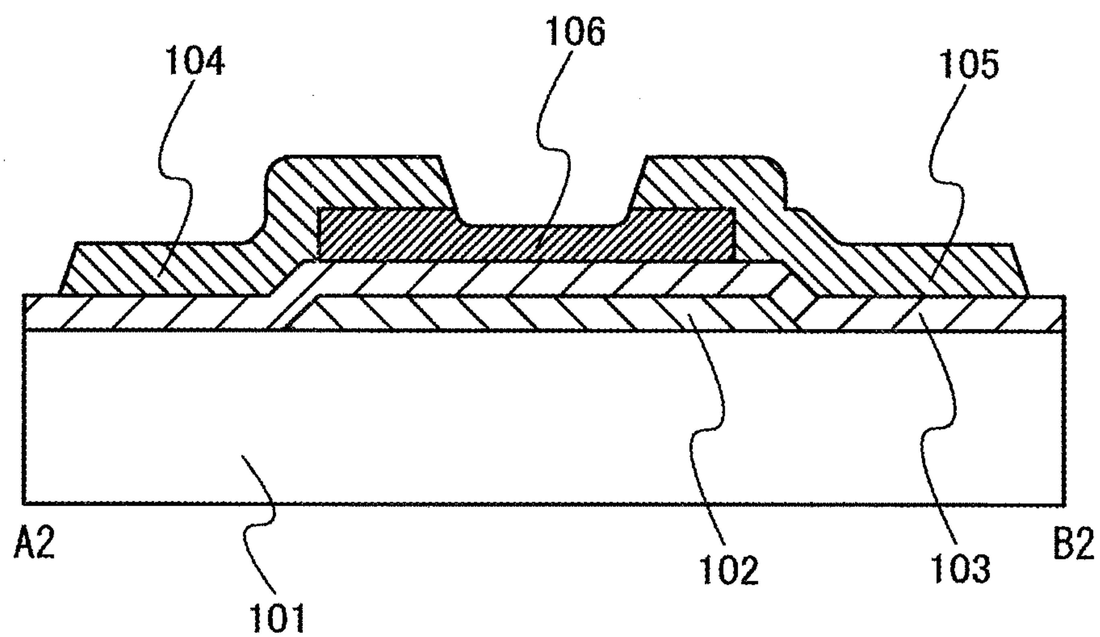
FIG. 2B
