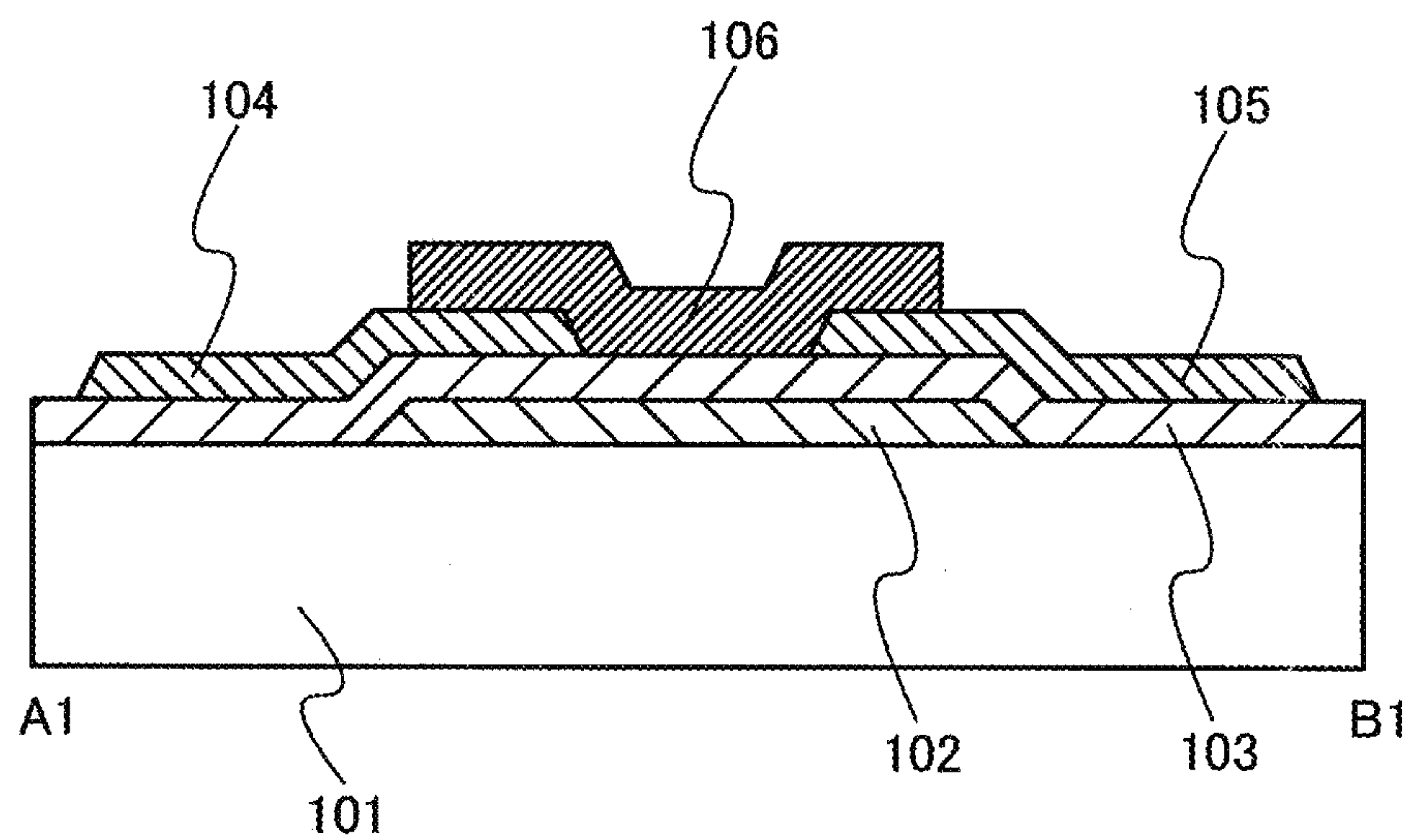
FIG. 1B
