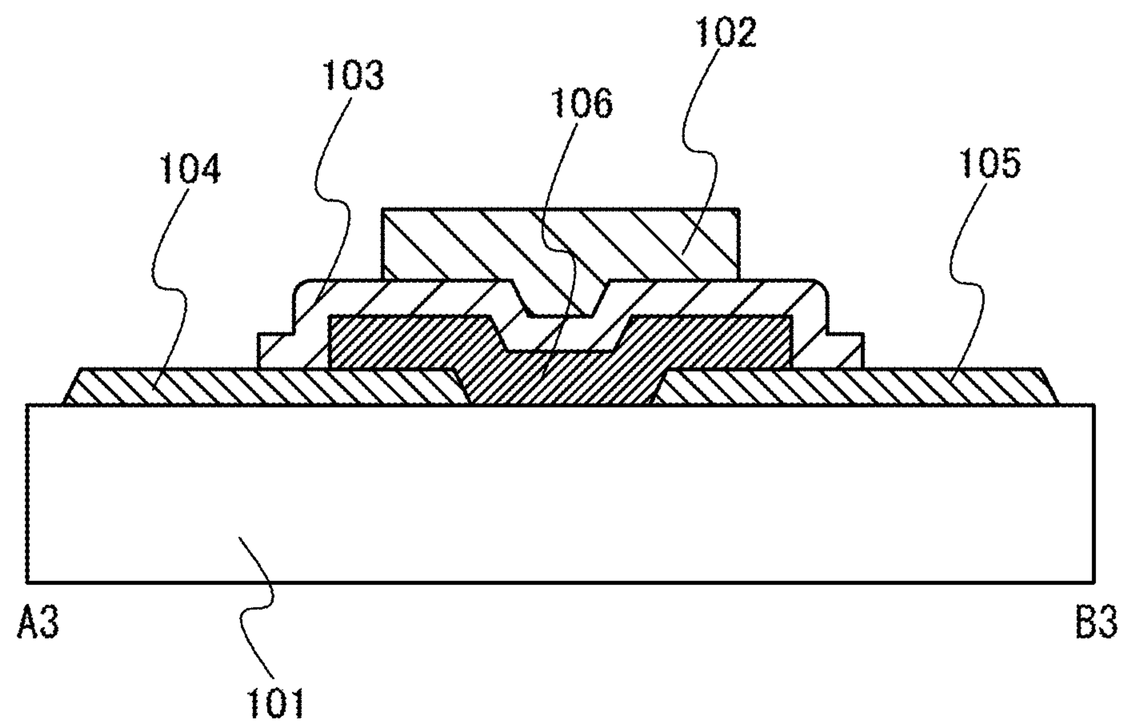
FIG. 3B
