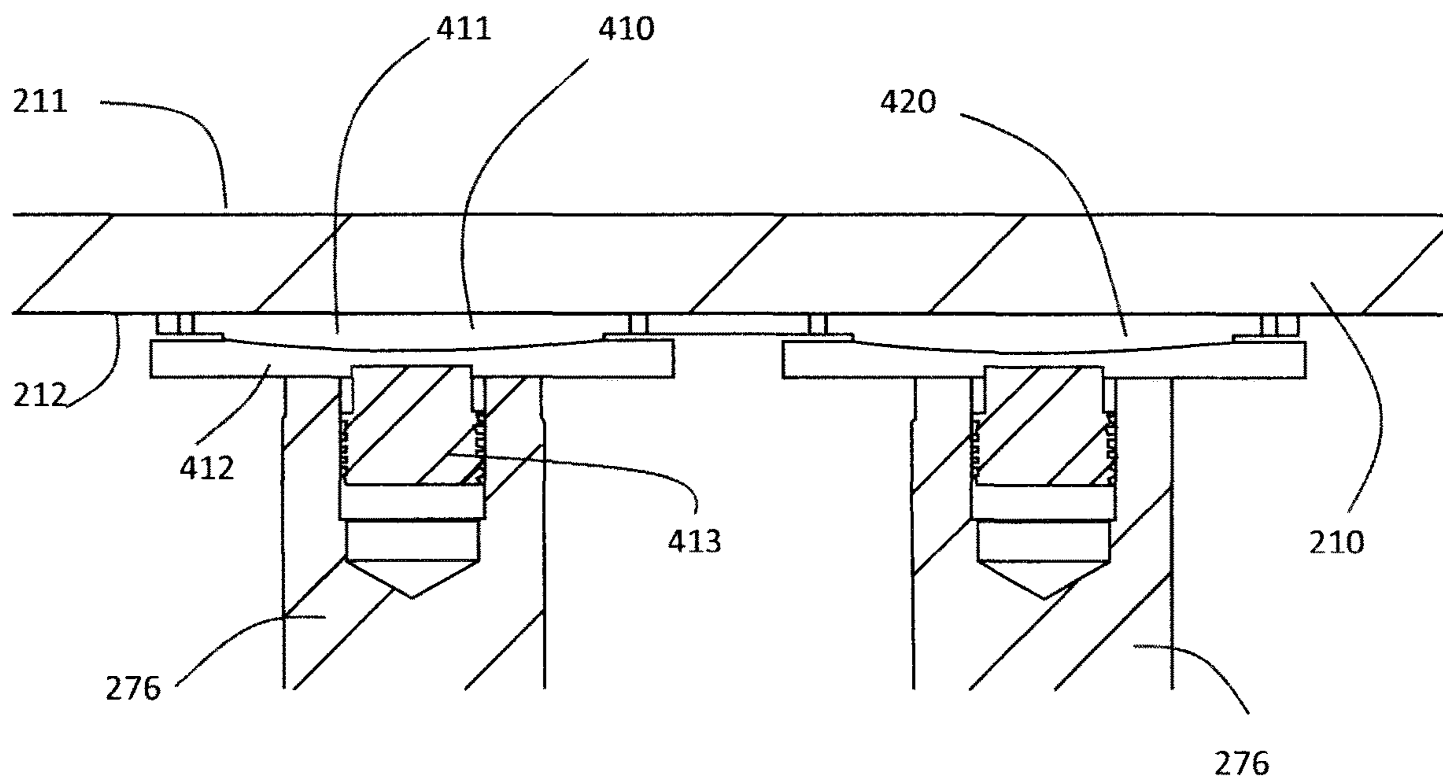
SECTION A-A
