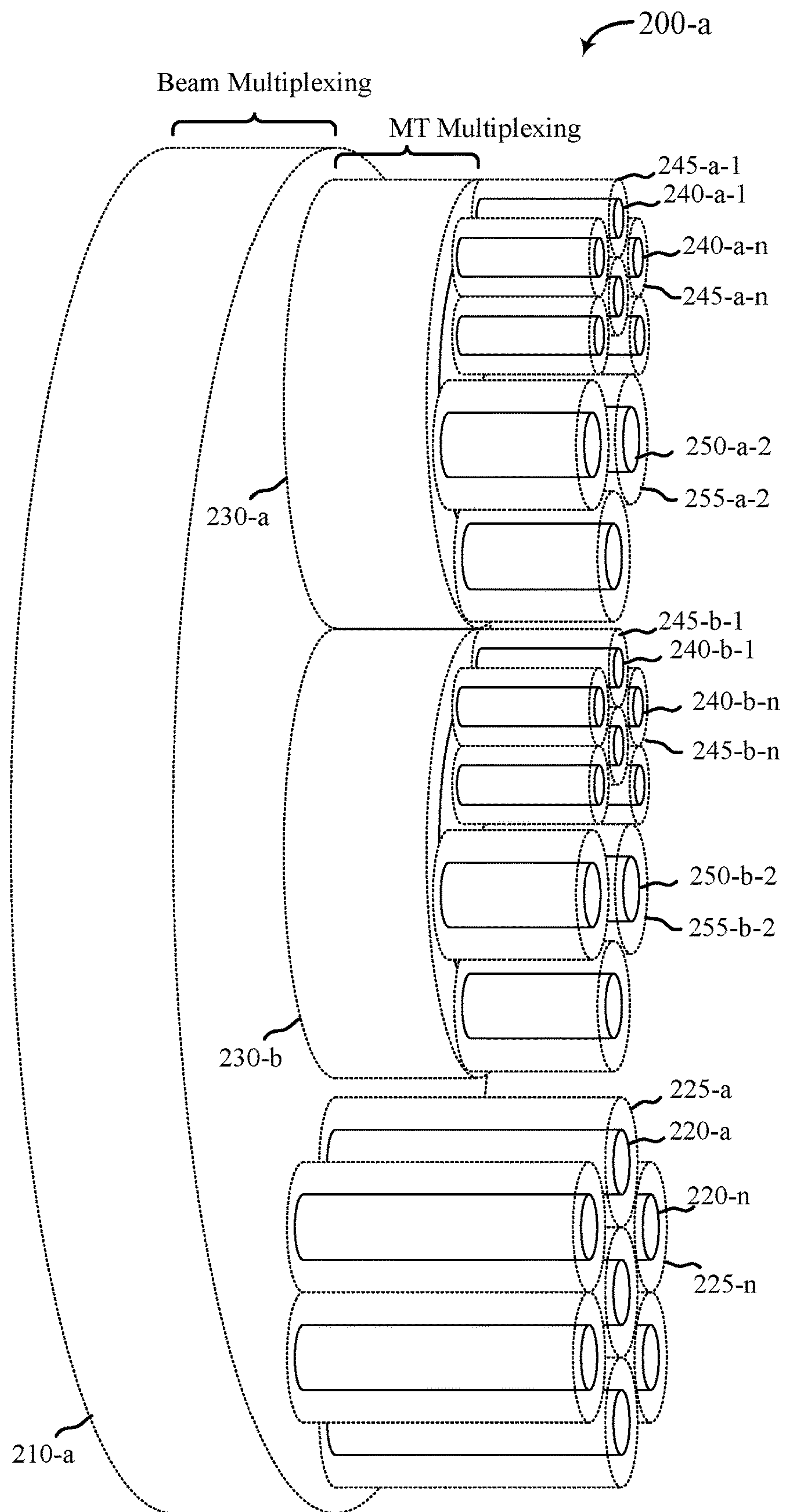
FIG. 2A
