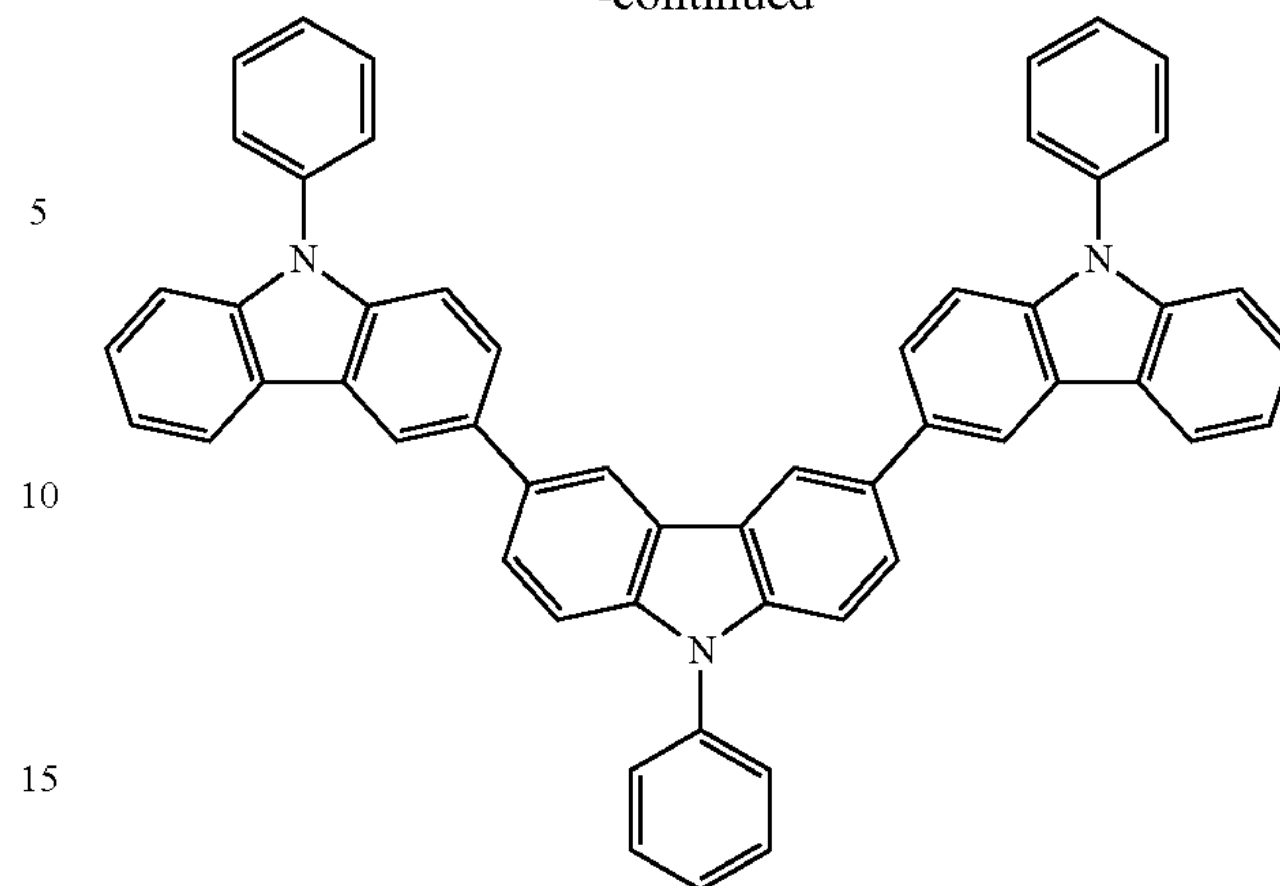
Tris-PCz
