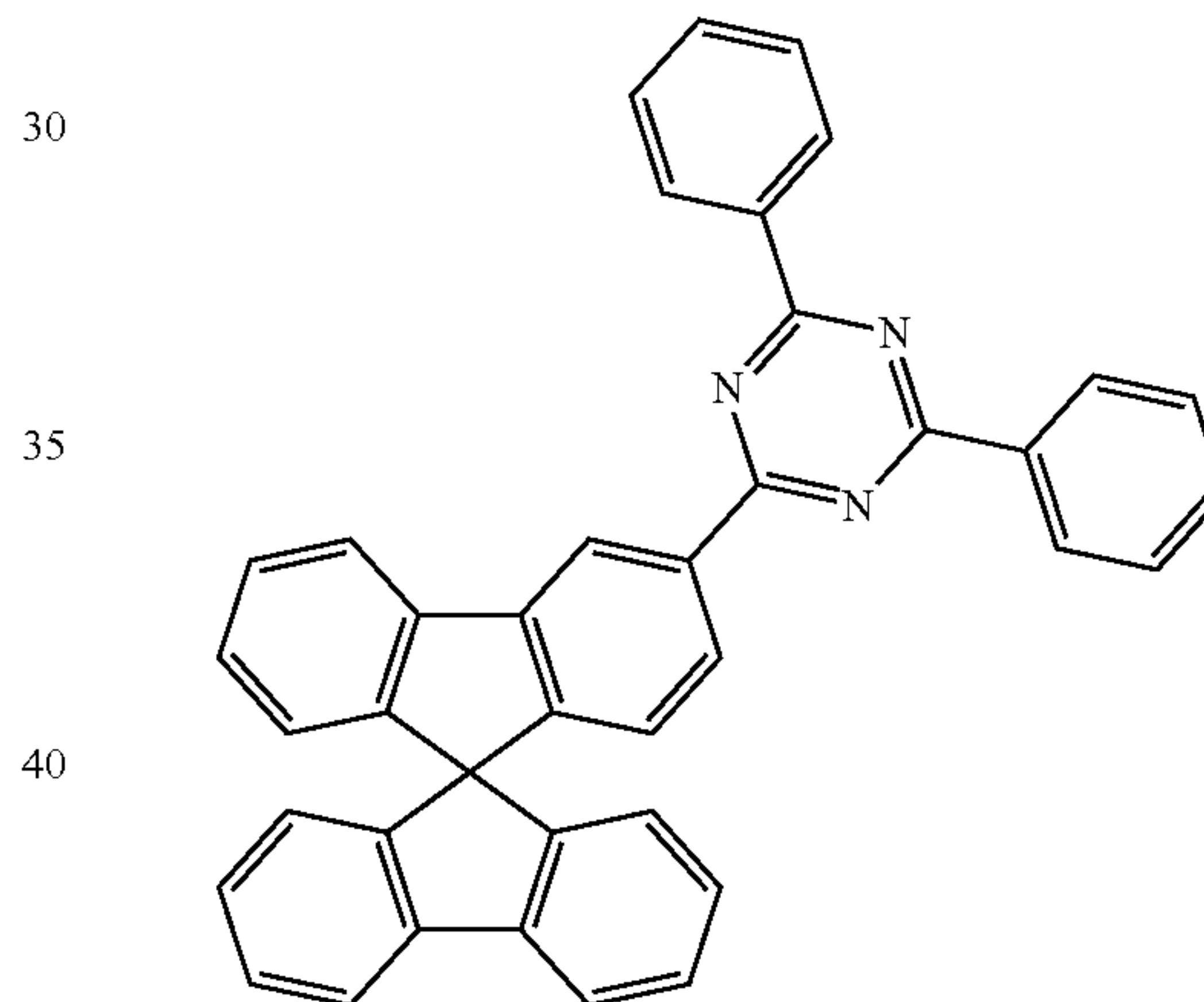
SF3-TRZ
