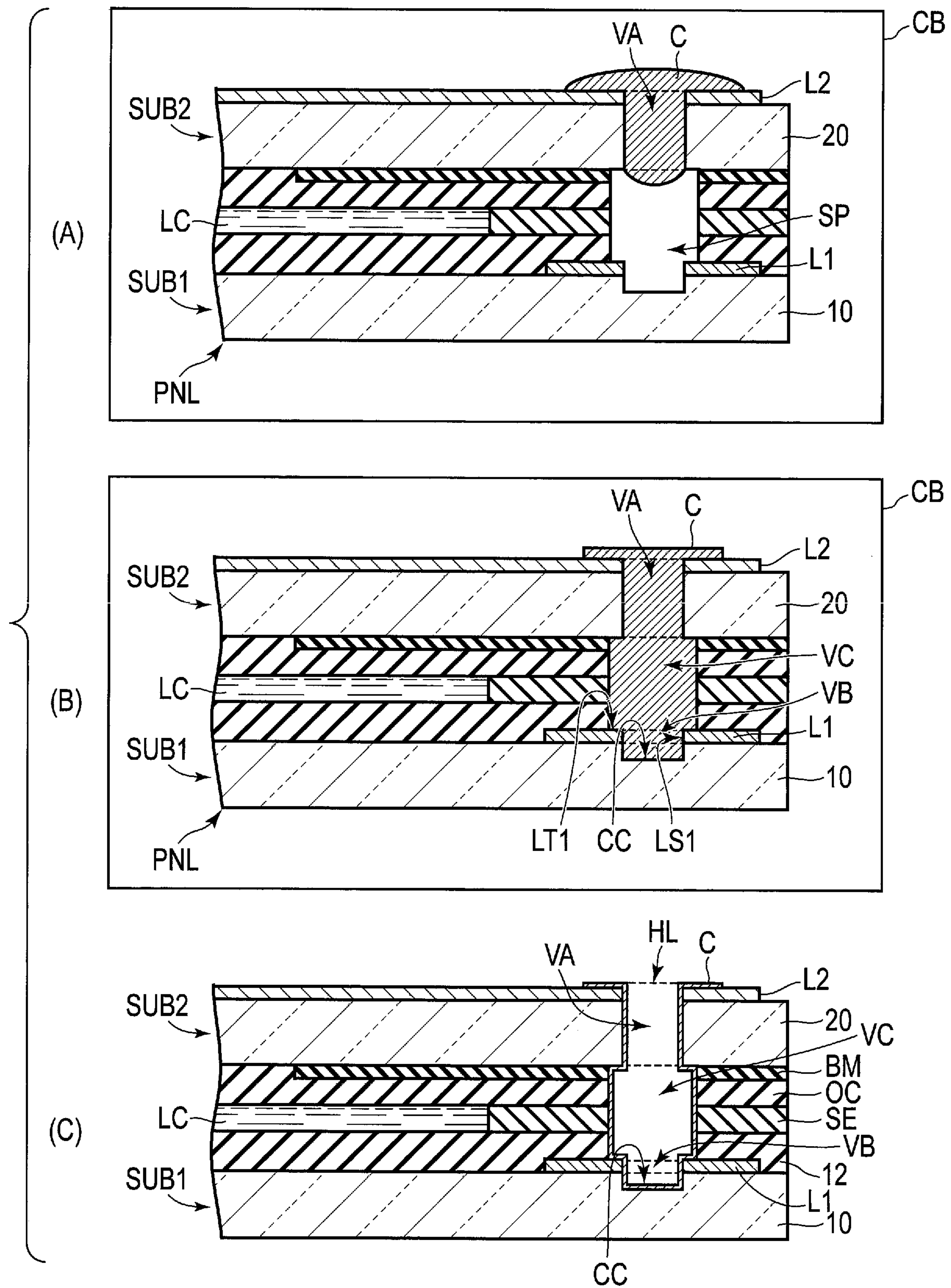
FIG. 18
