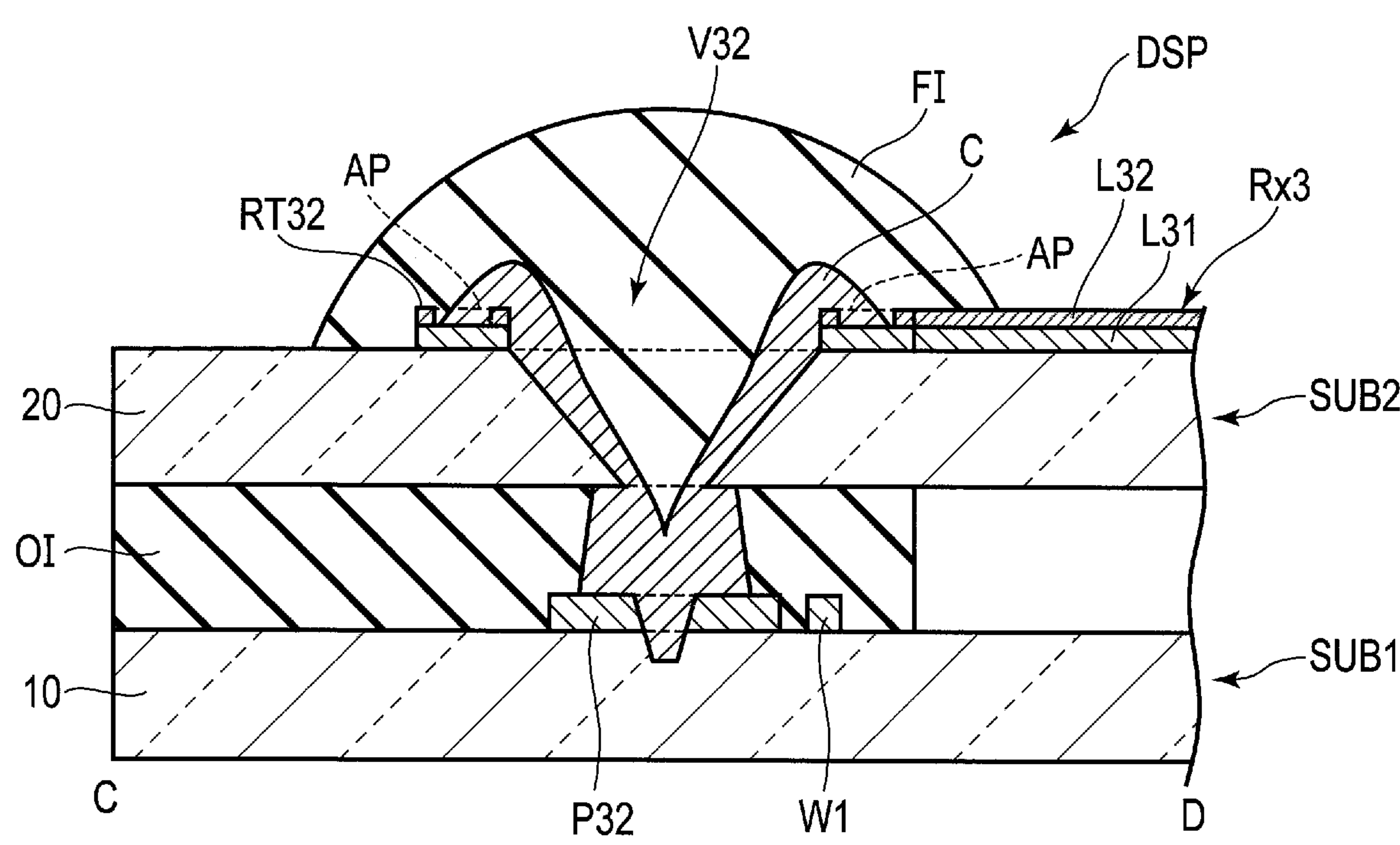
FIG. 23
