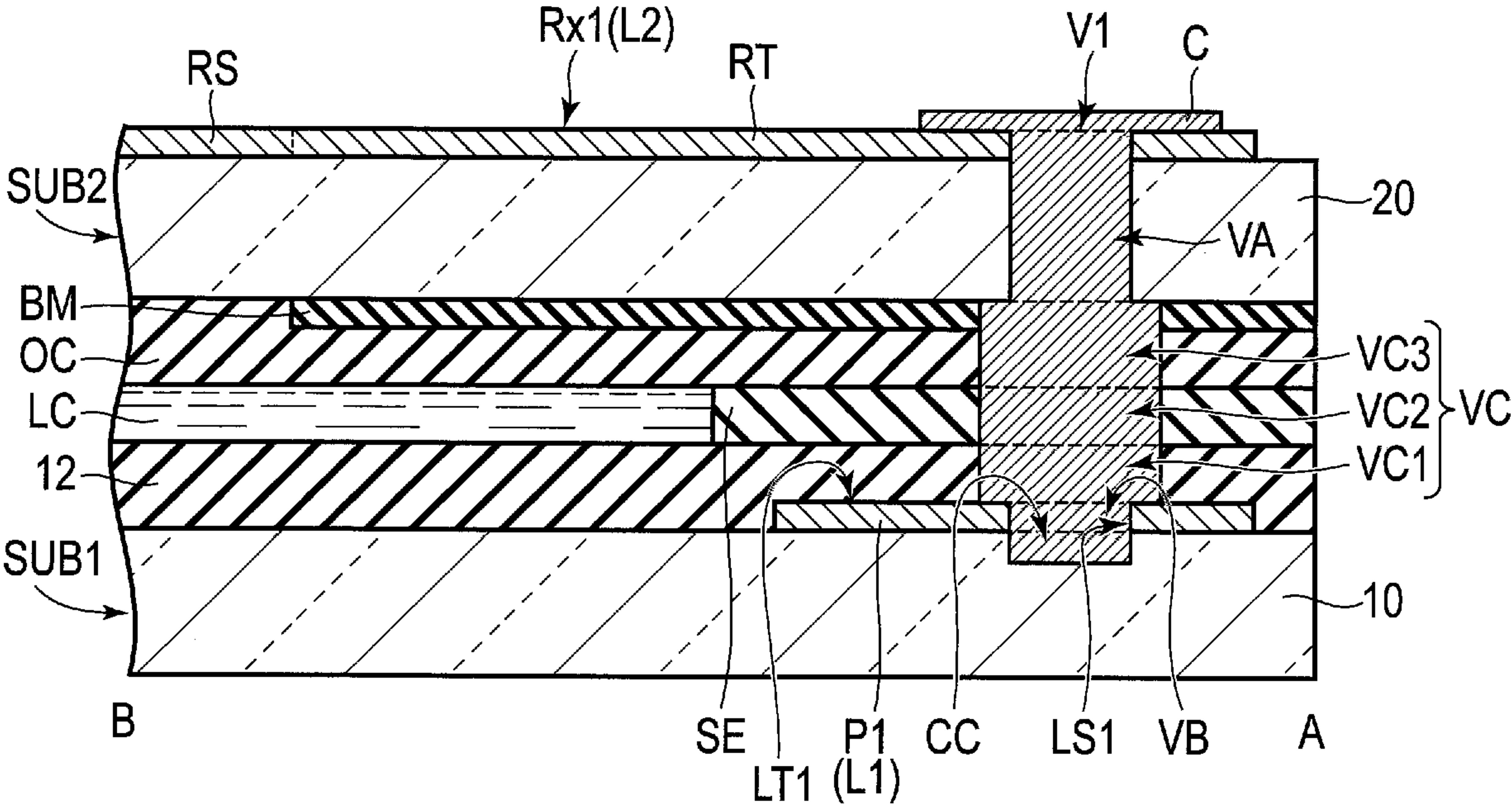
FIG. 16A
