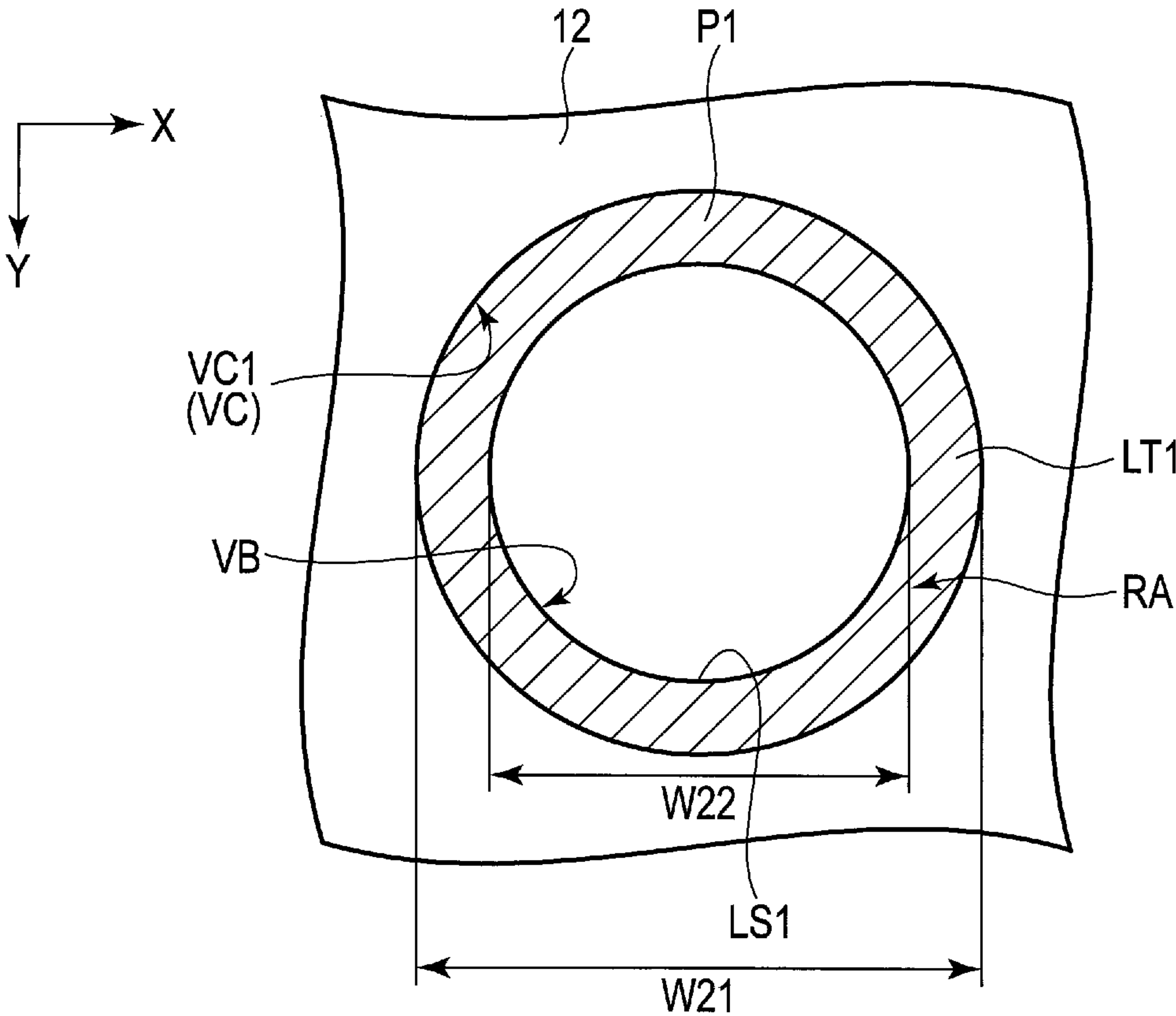
FIG. 16B
