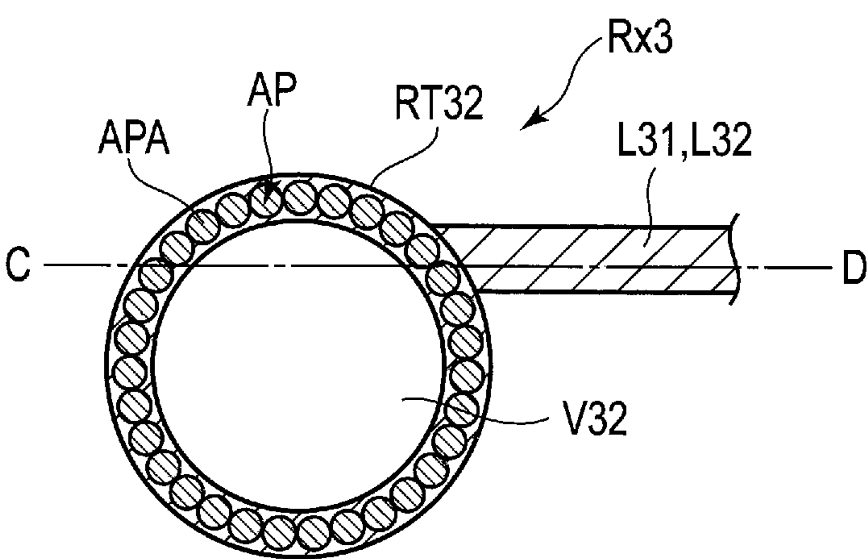
FIG. 22
