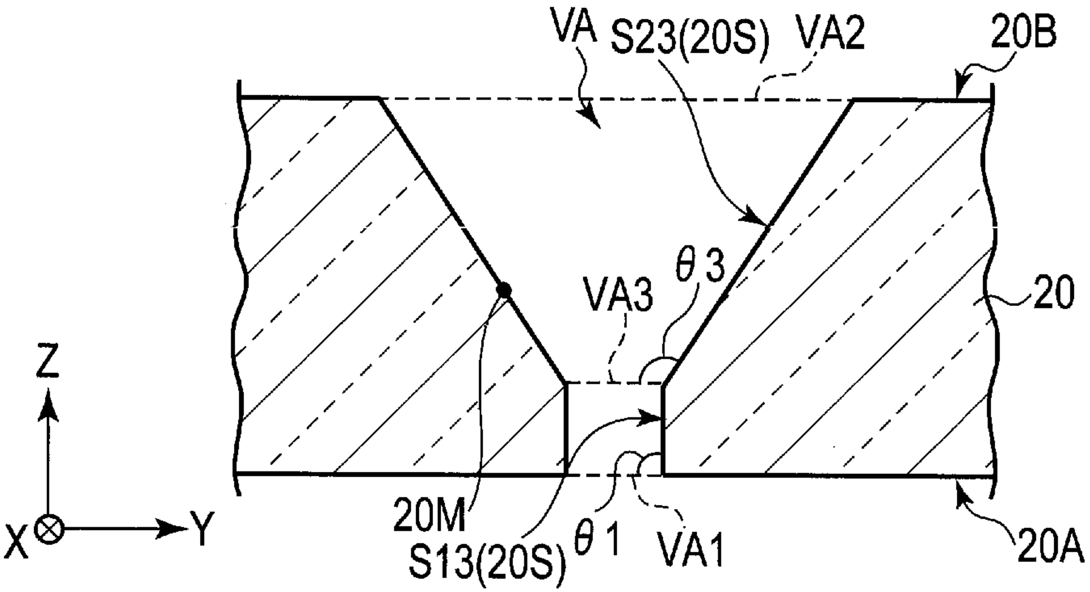
FIG. 29B
