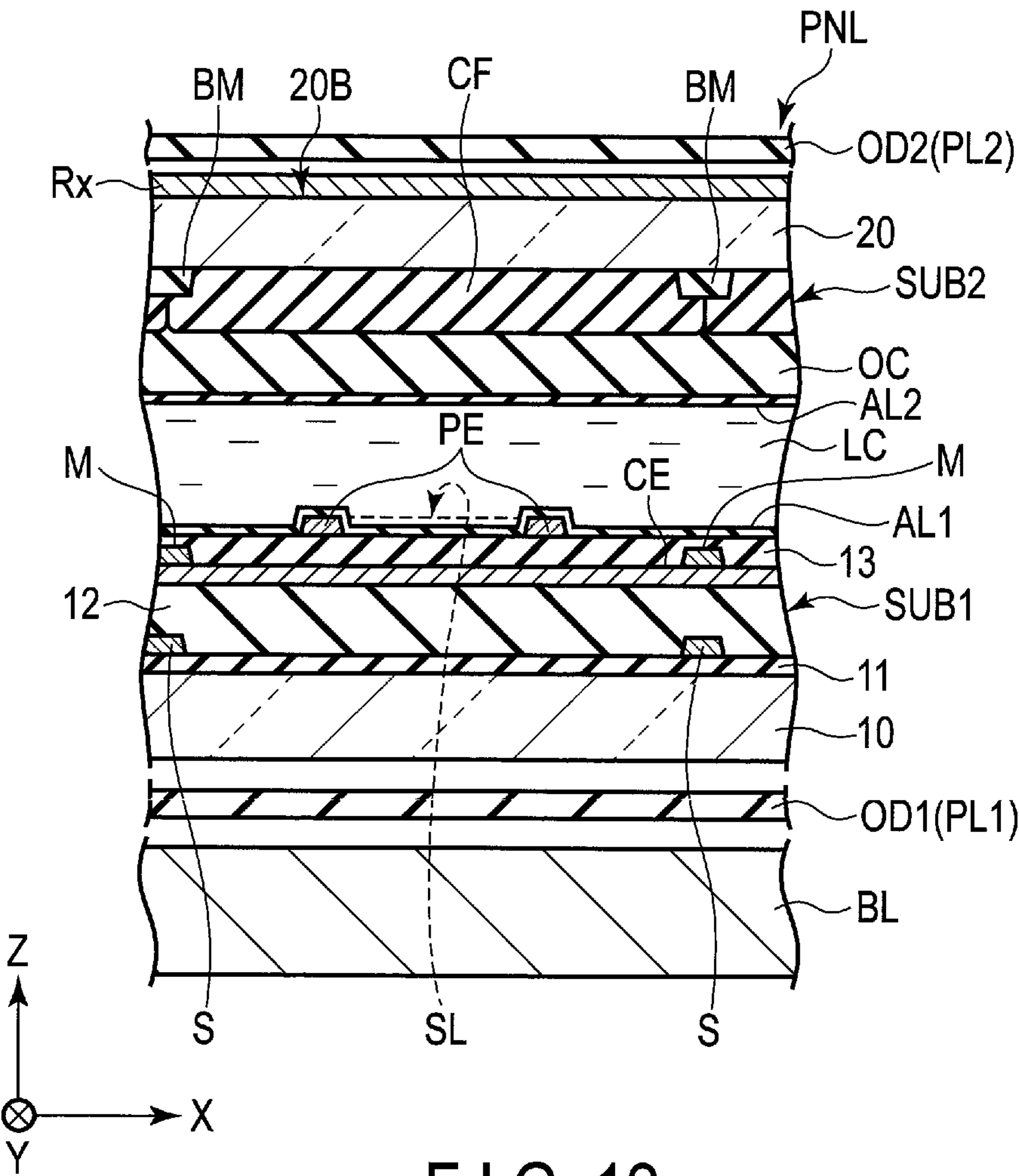
FIG. 12
