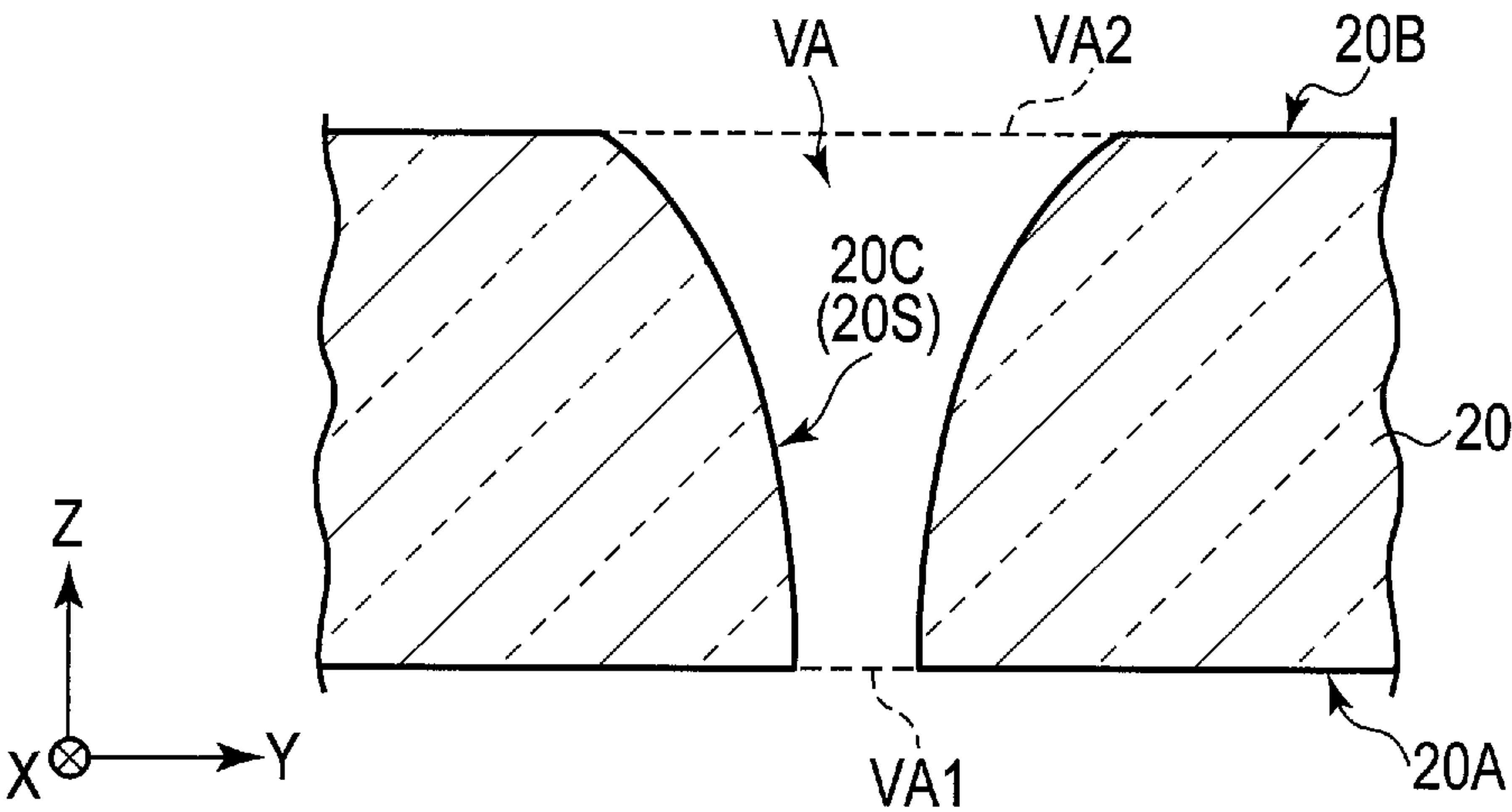
FIG. 28A
