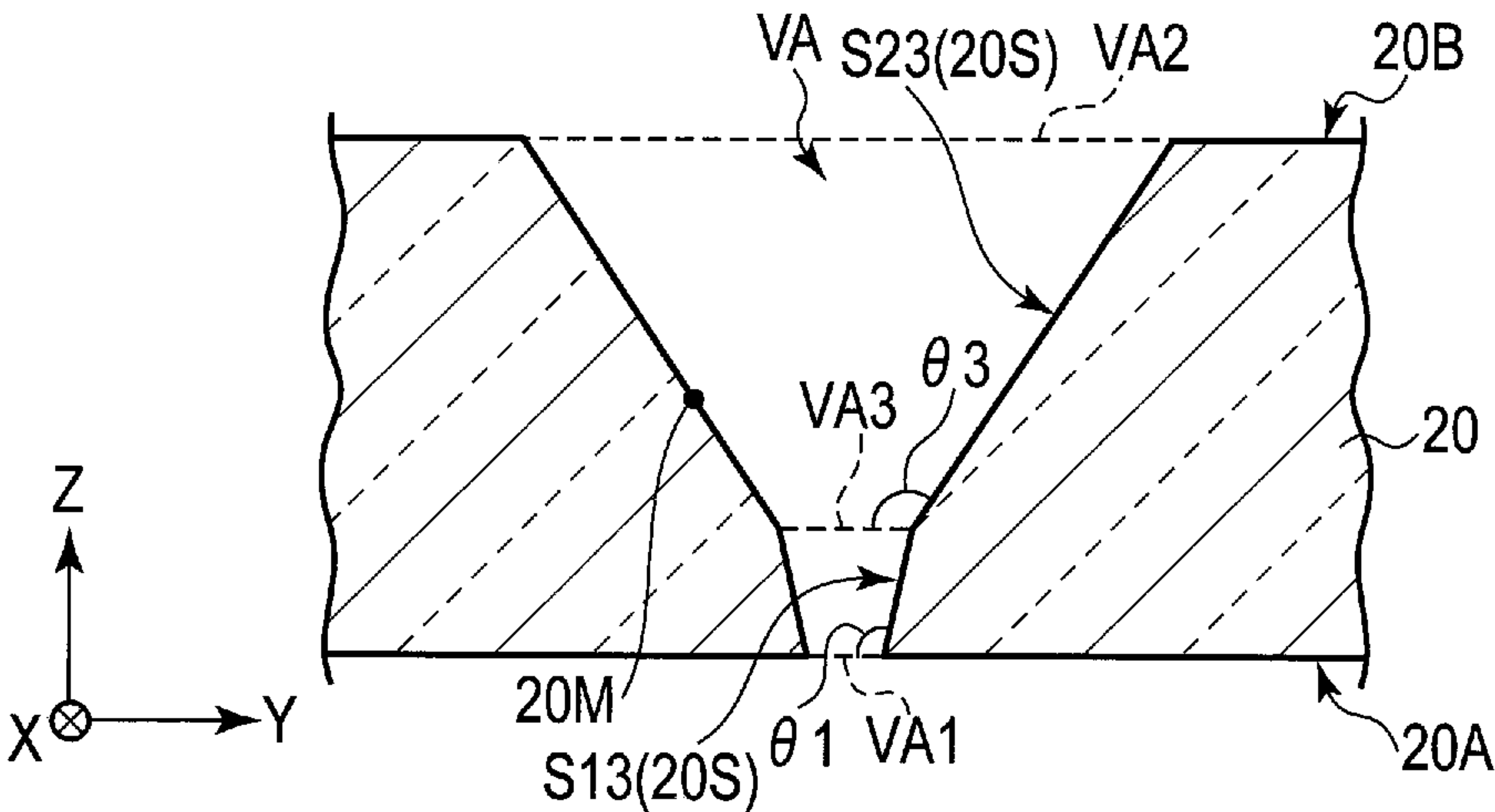
FIG. 29A
