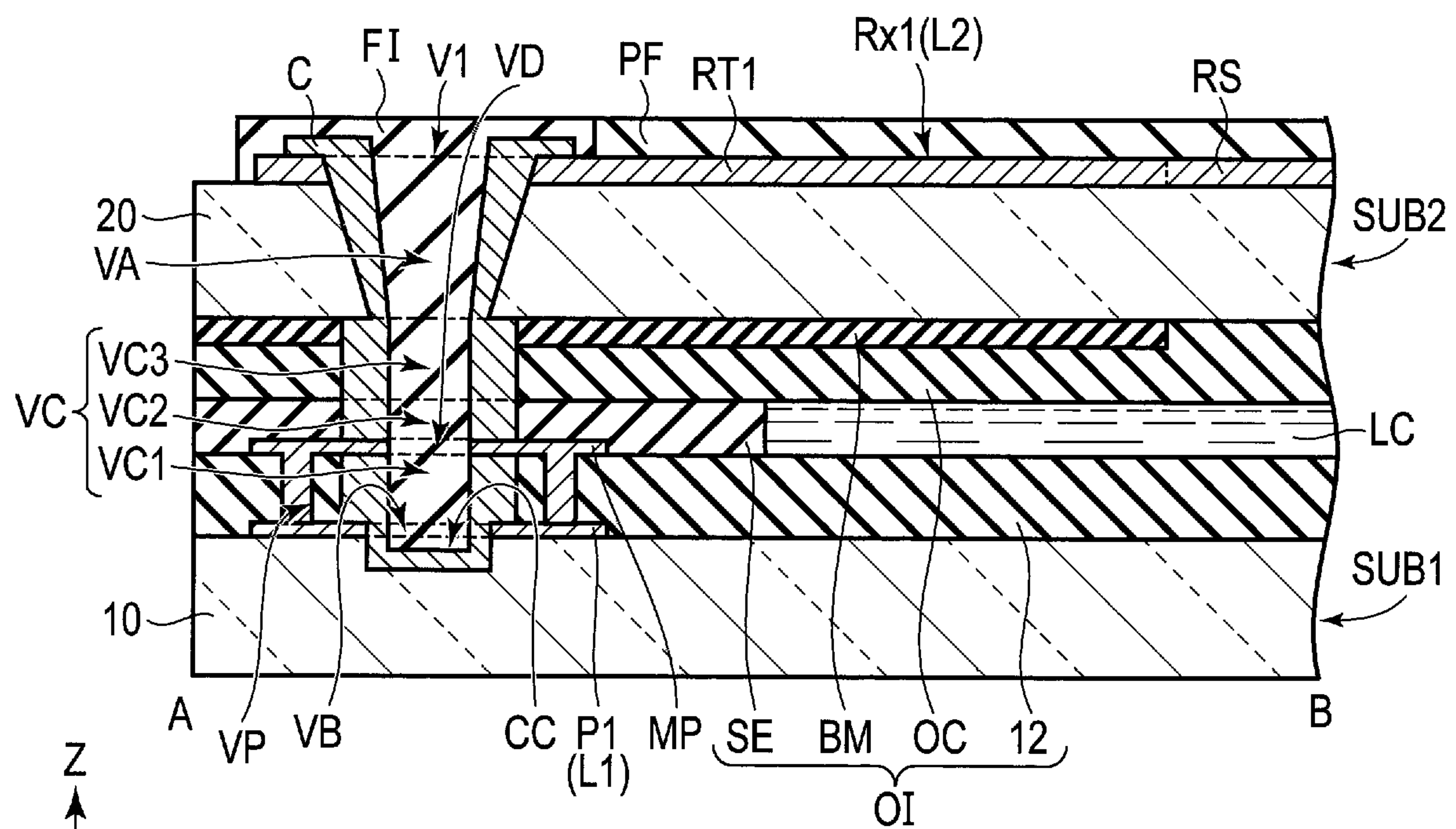
FIG. 33
