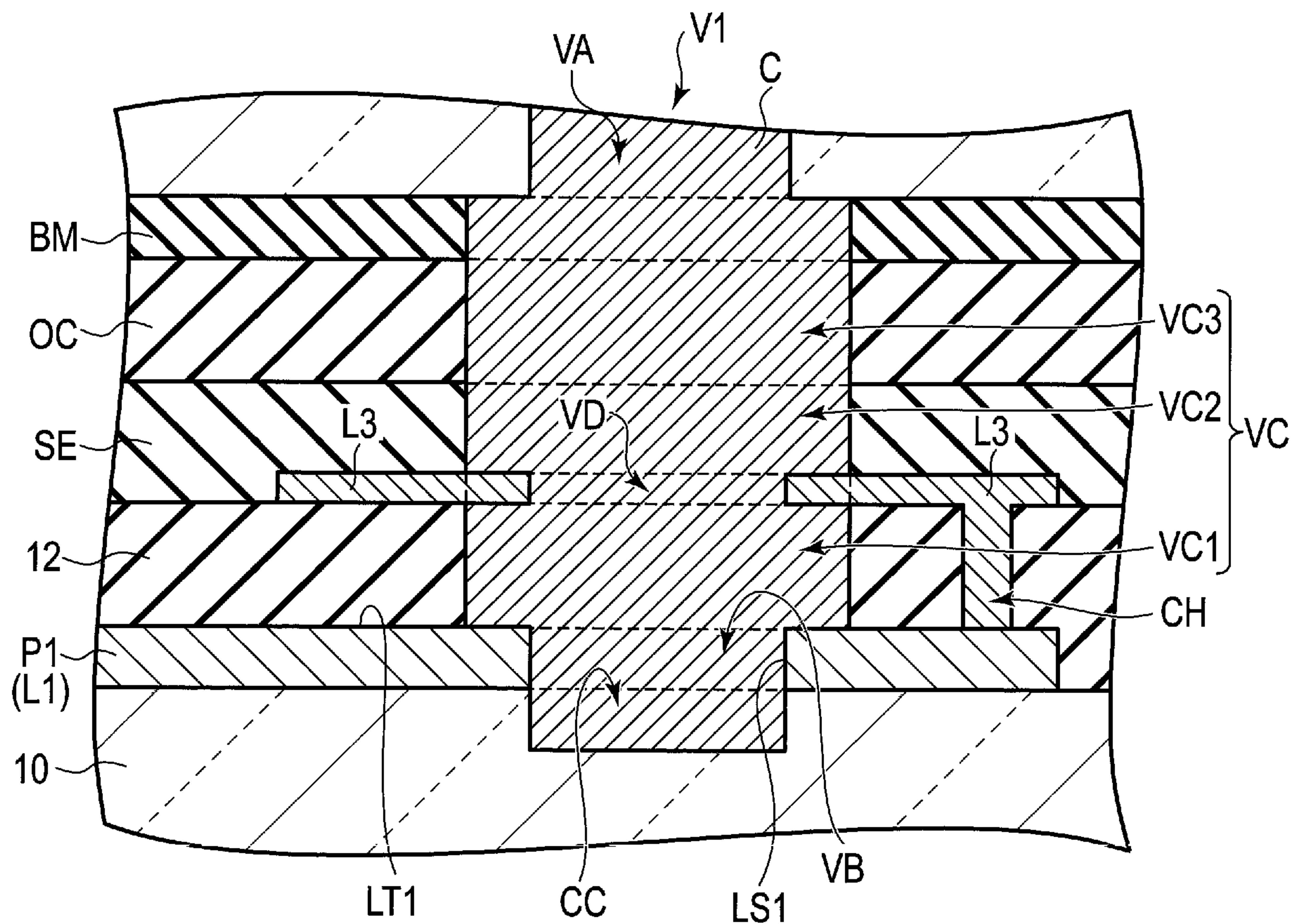
FIG. 24
