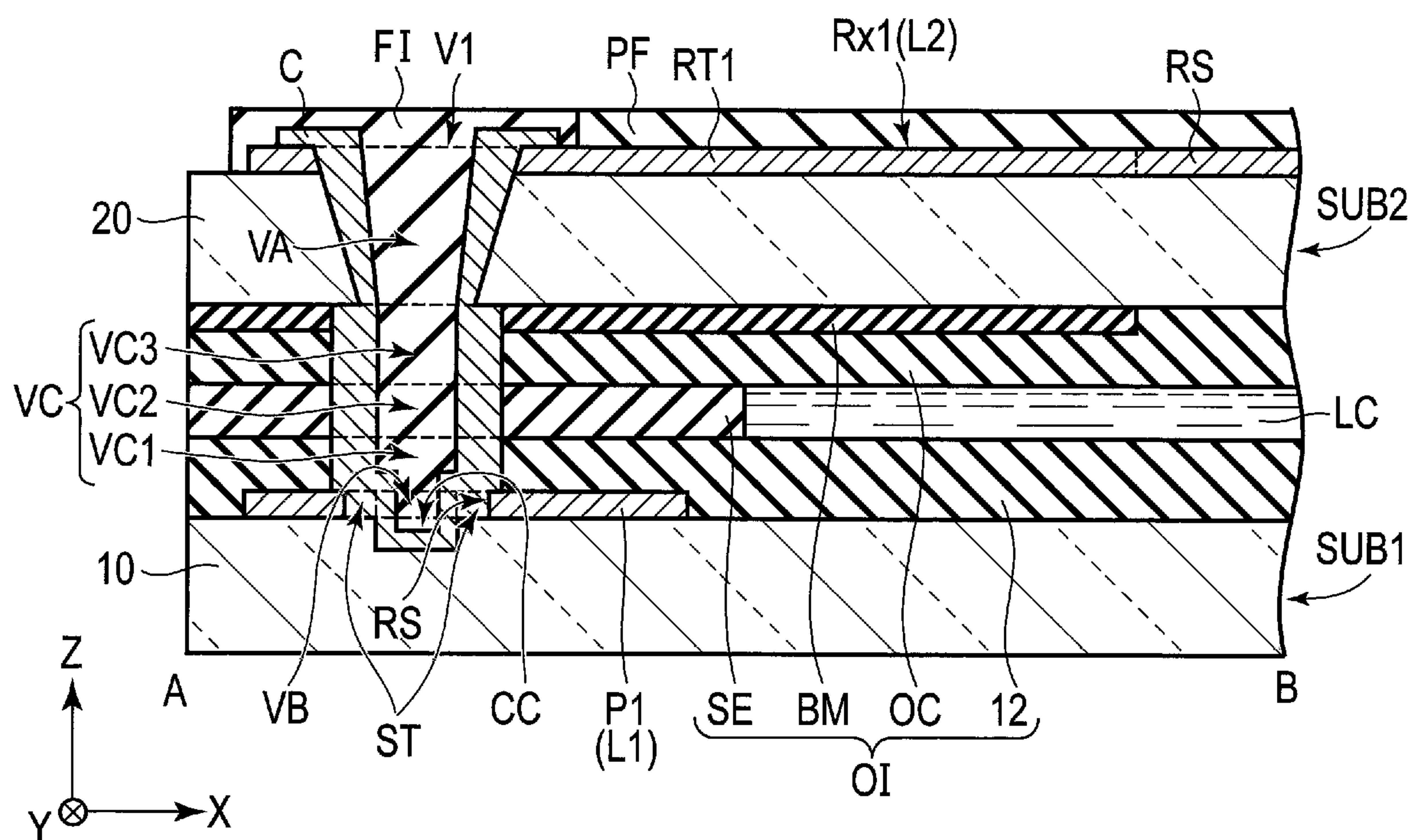
FIG. 31
