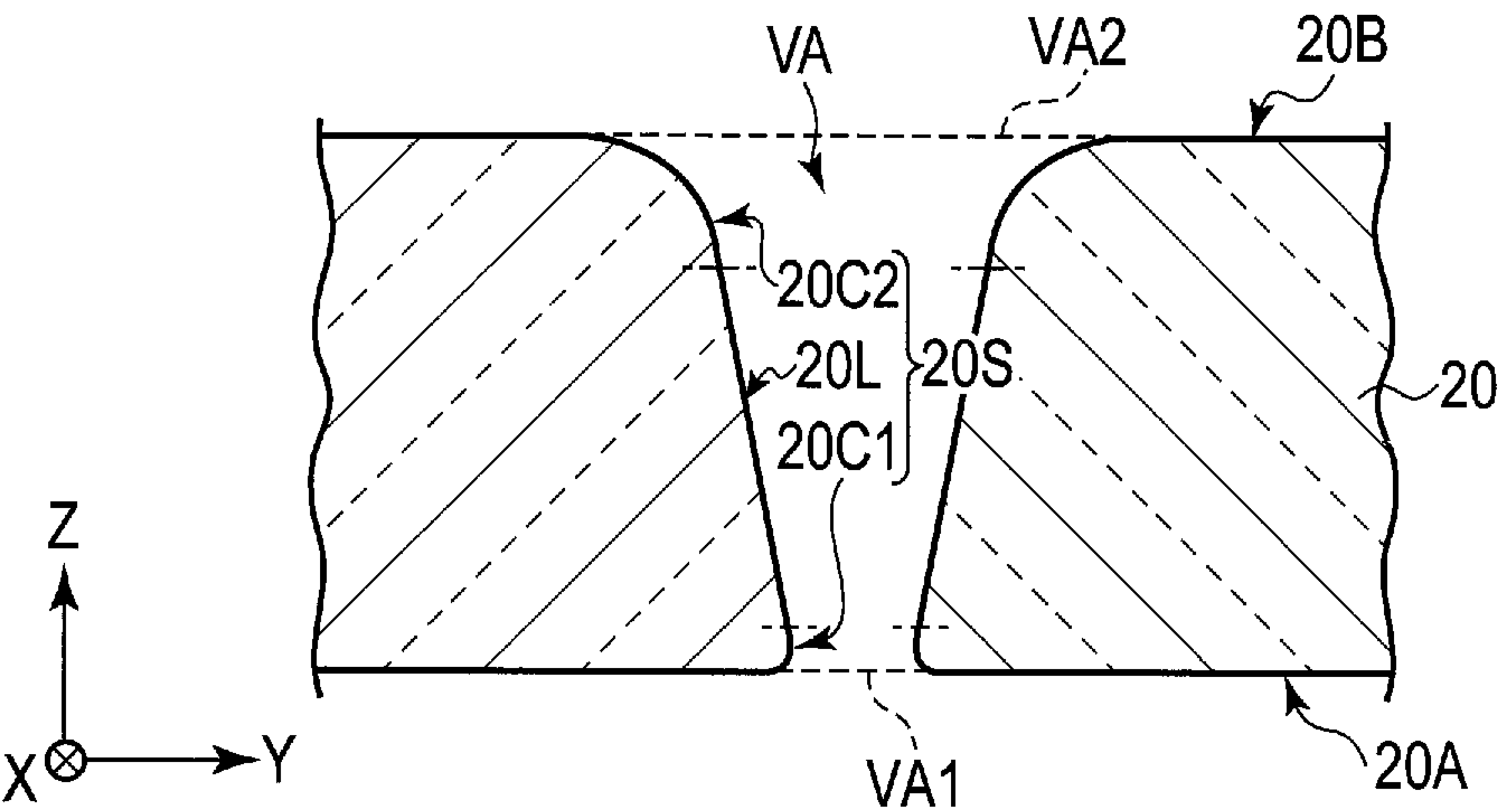
FIG. 28C
