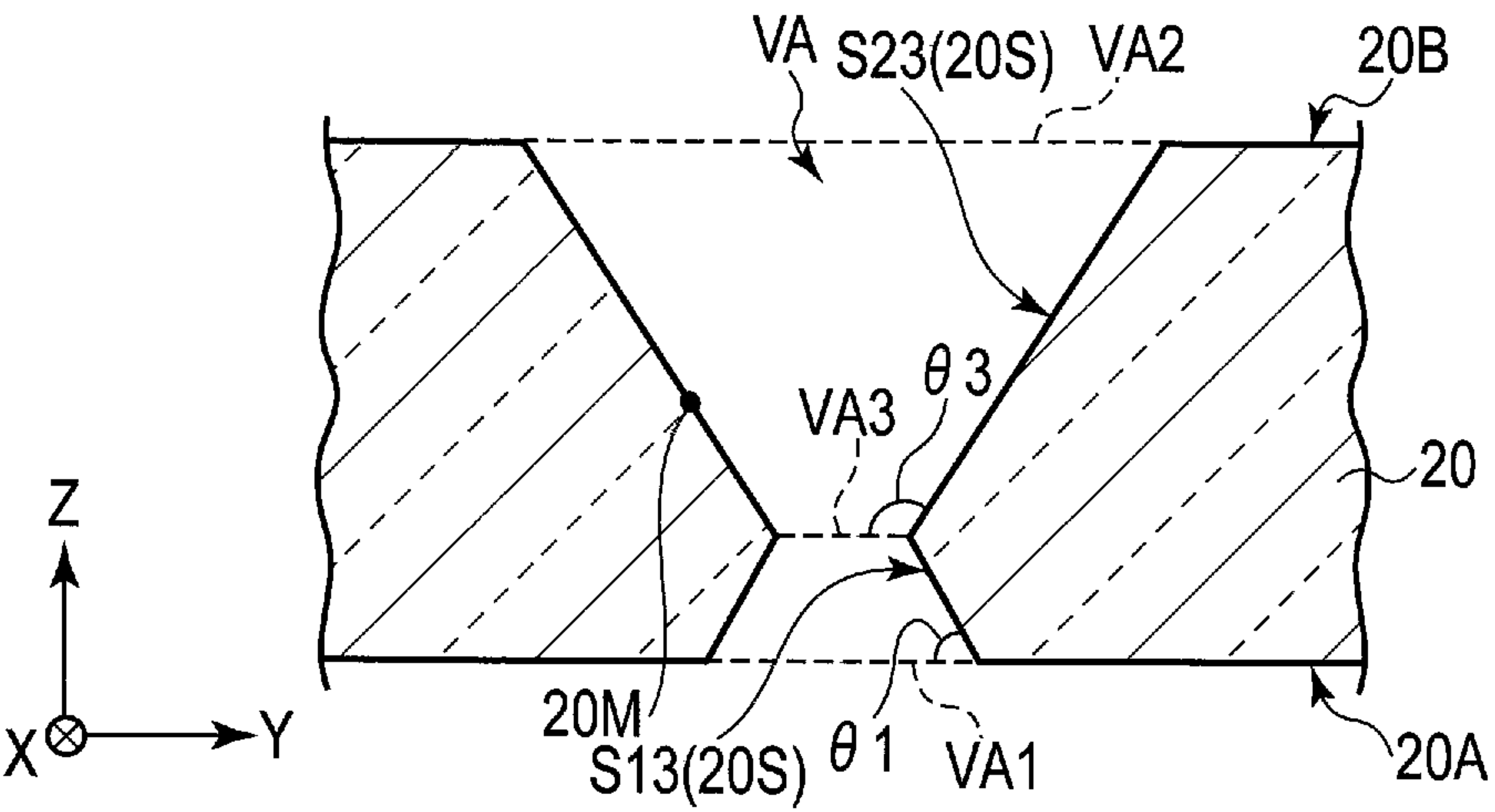
FIG. 29C
