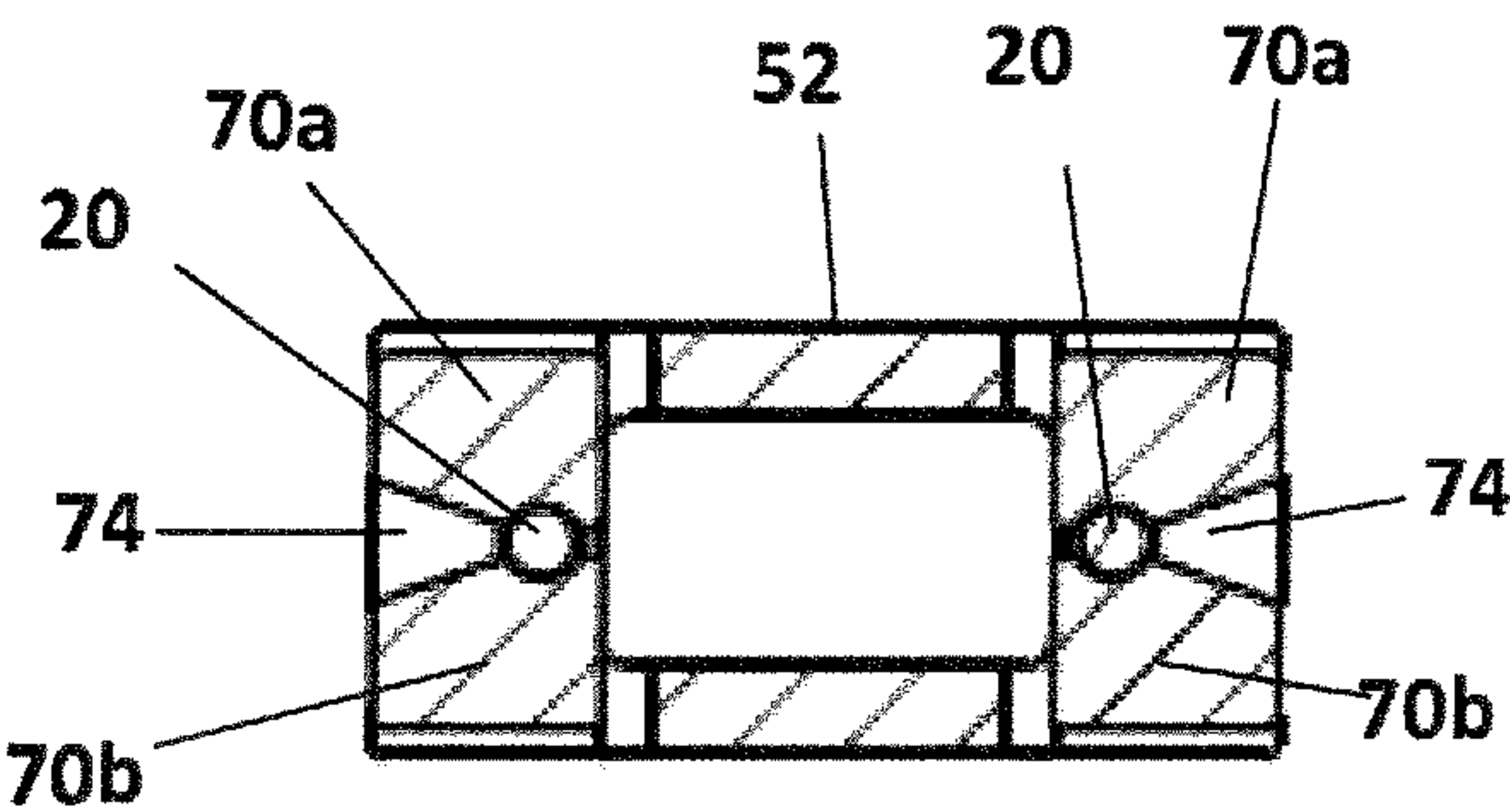
SECTION D-D
