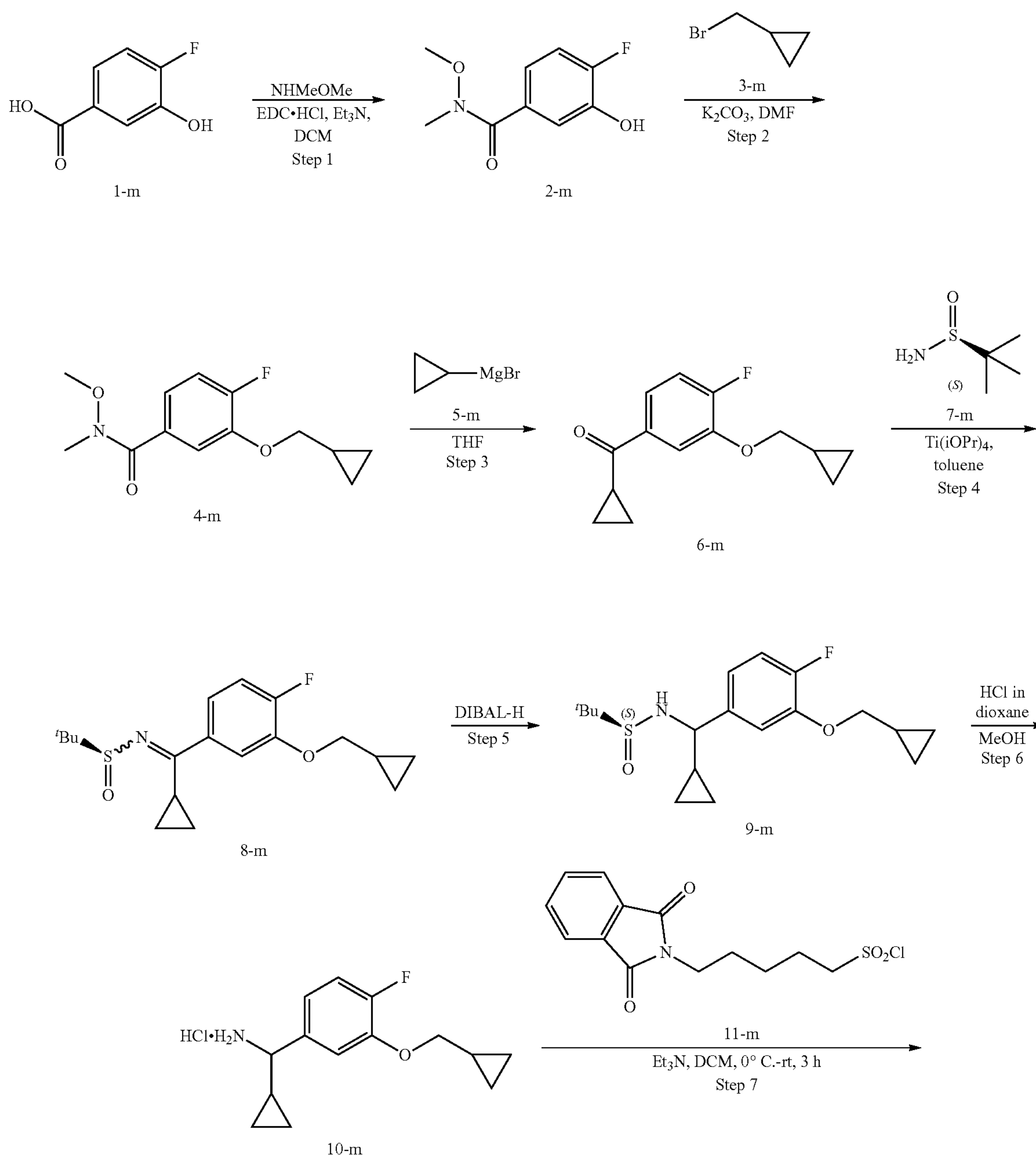
Scheme 14.
