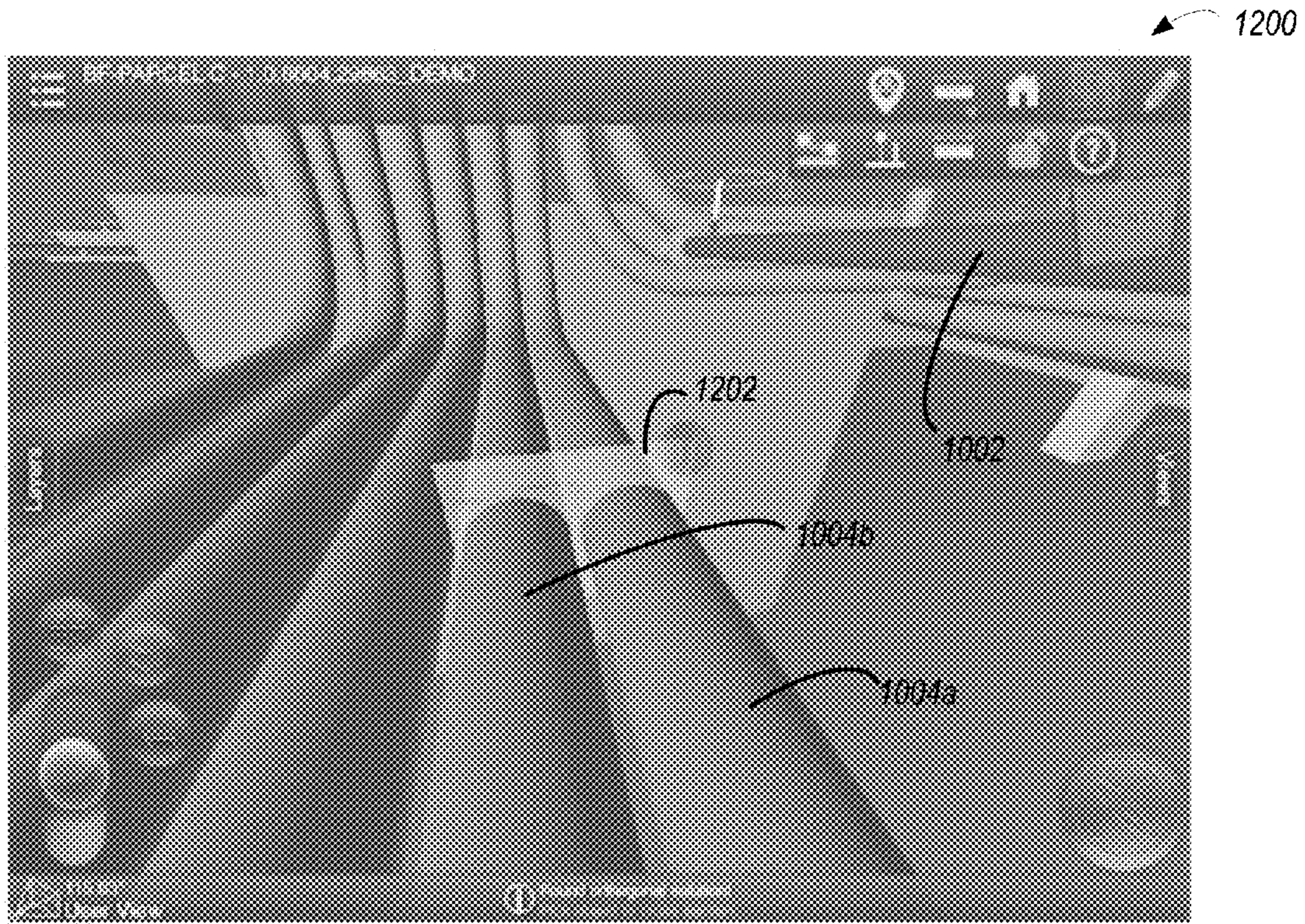
Fig. 12A
