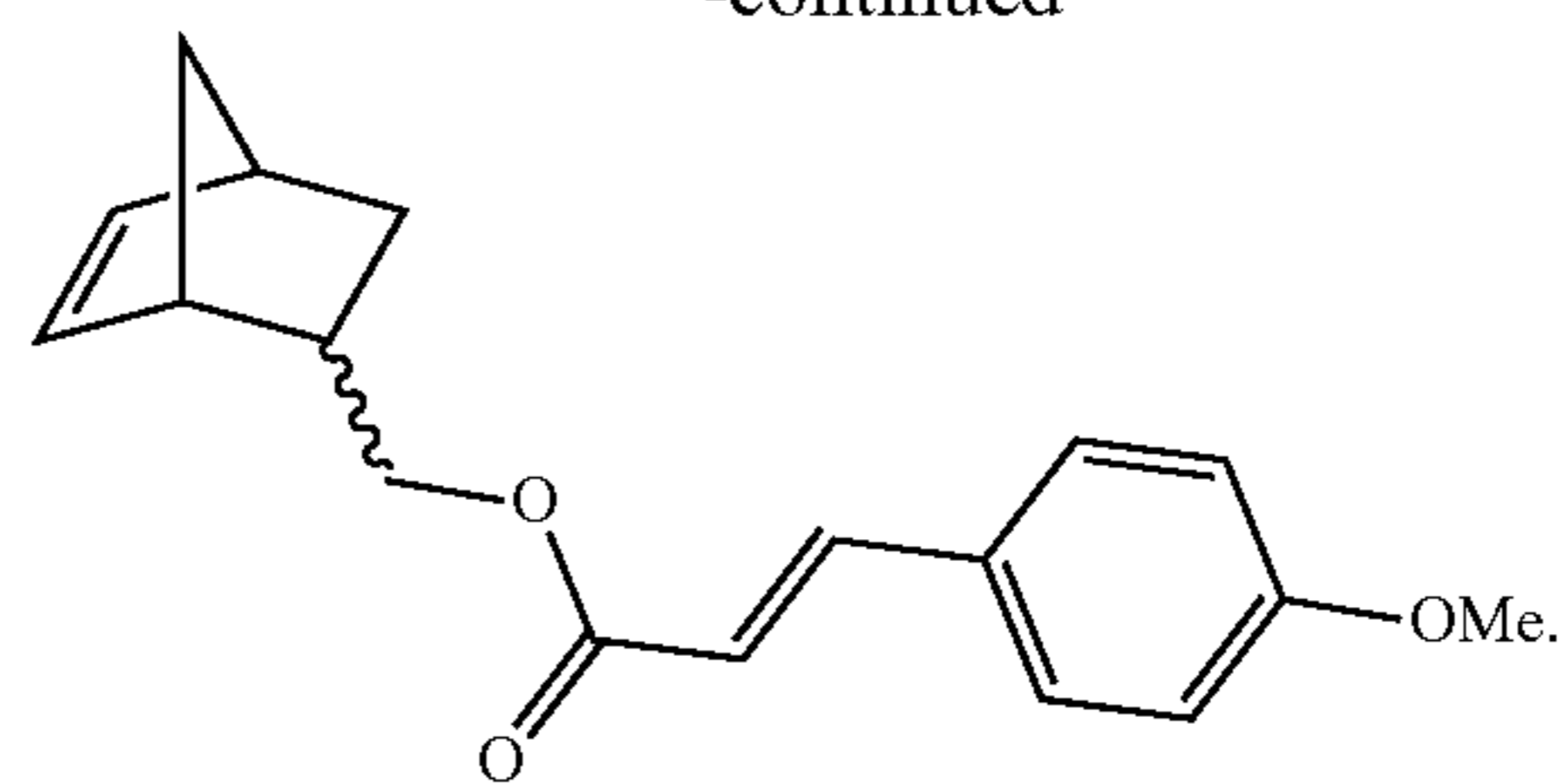
(bicyclo[2.2.1]hept-5-en-2-yl)methyl 3-(4-methoxyphenyl)acrylate (NBMeOCinnamate)
