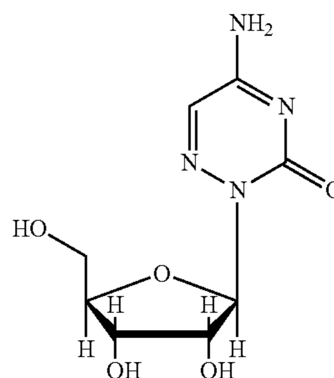
6-Azacytidine
