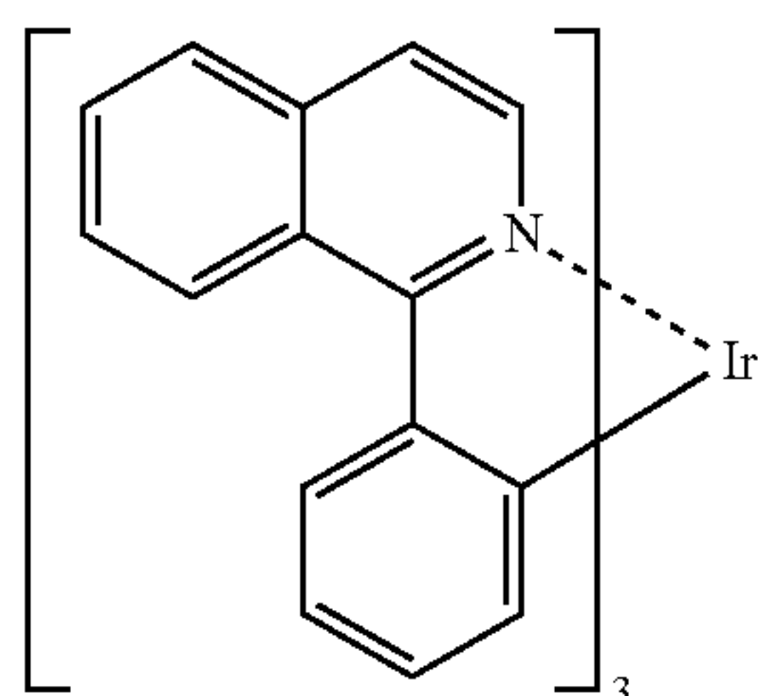
Ir(piq) 3
