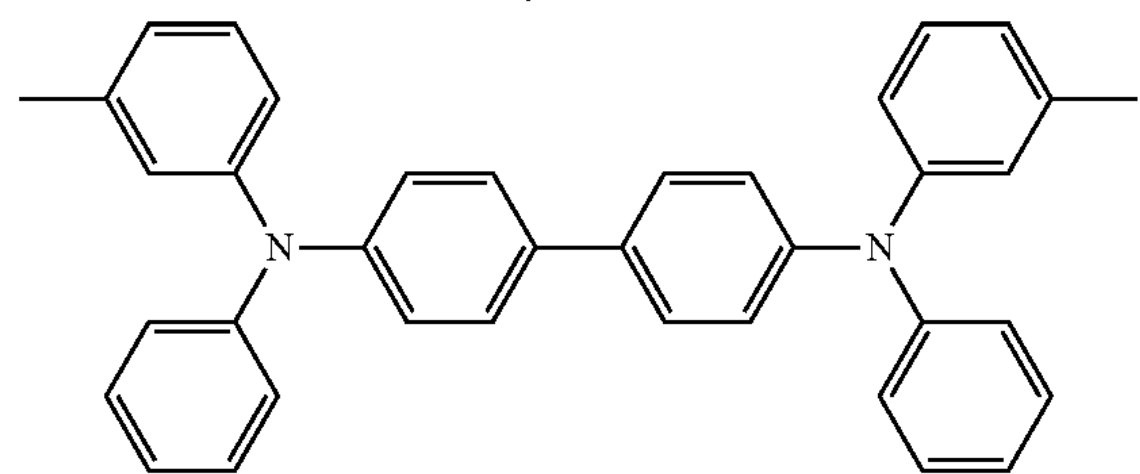
TPD
