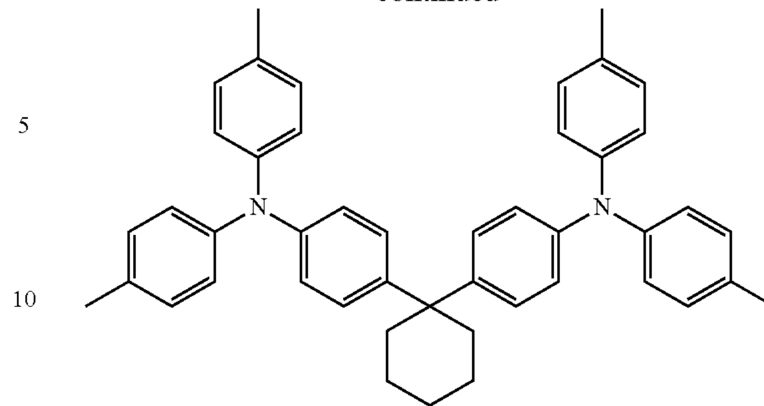
TAPC
