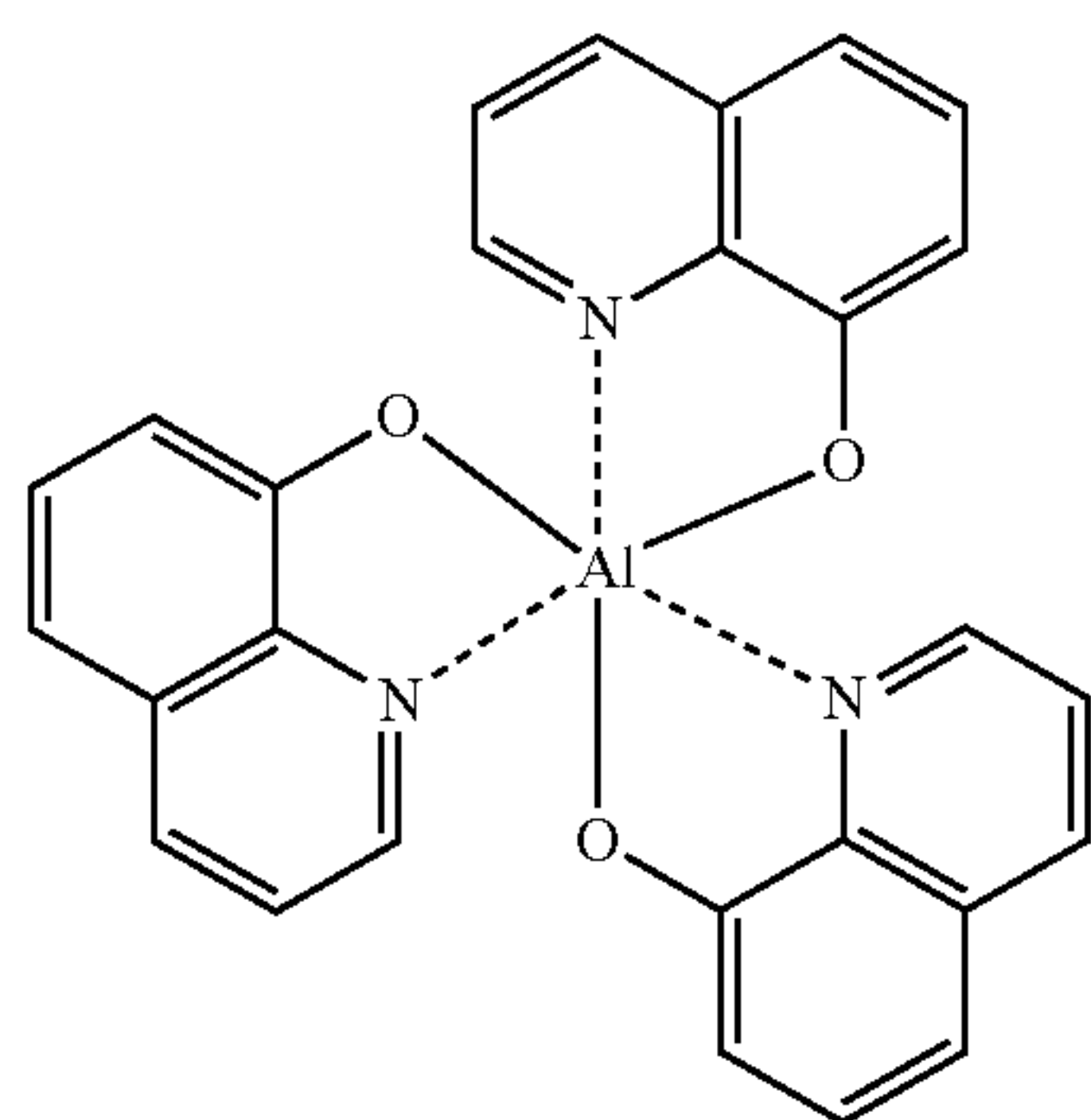
Alq 3
