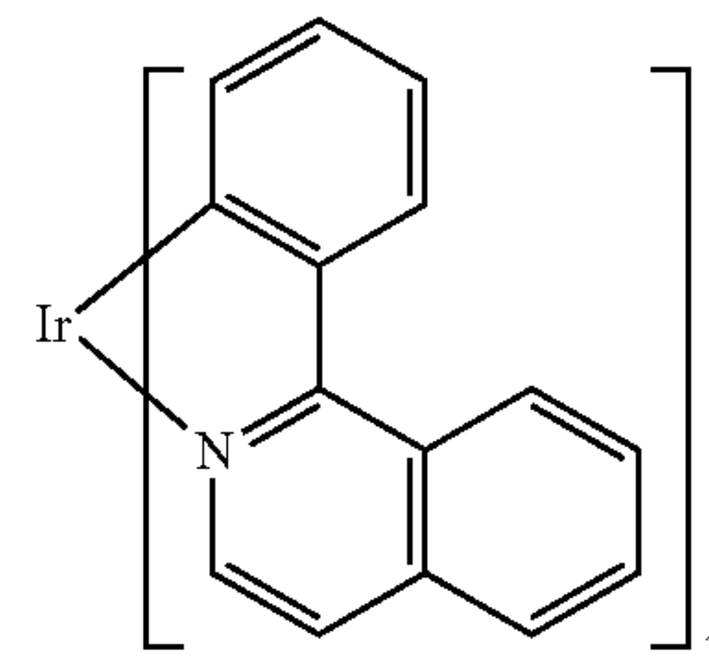
Ir(piq) 3
