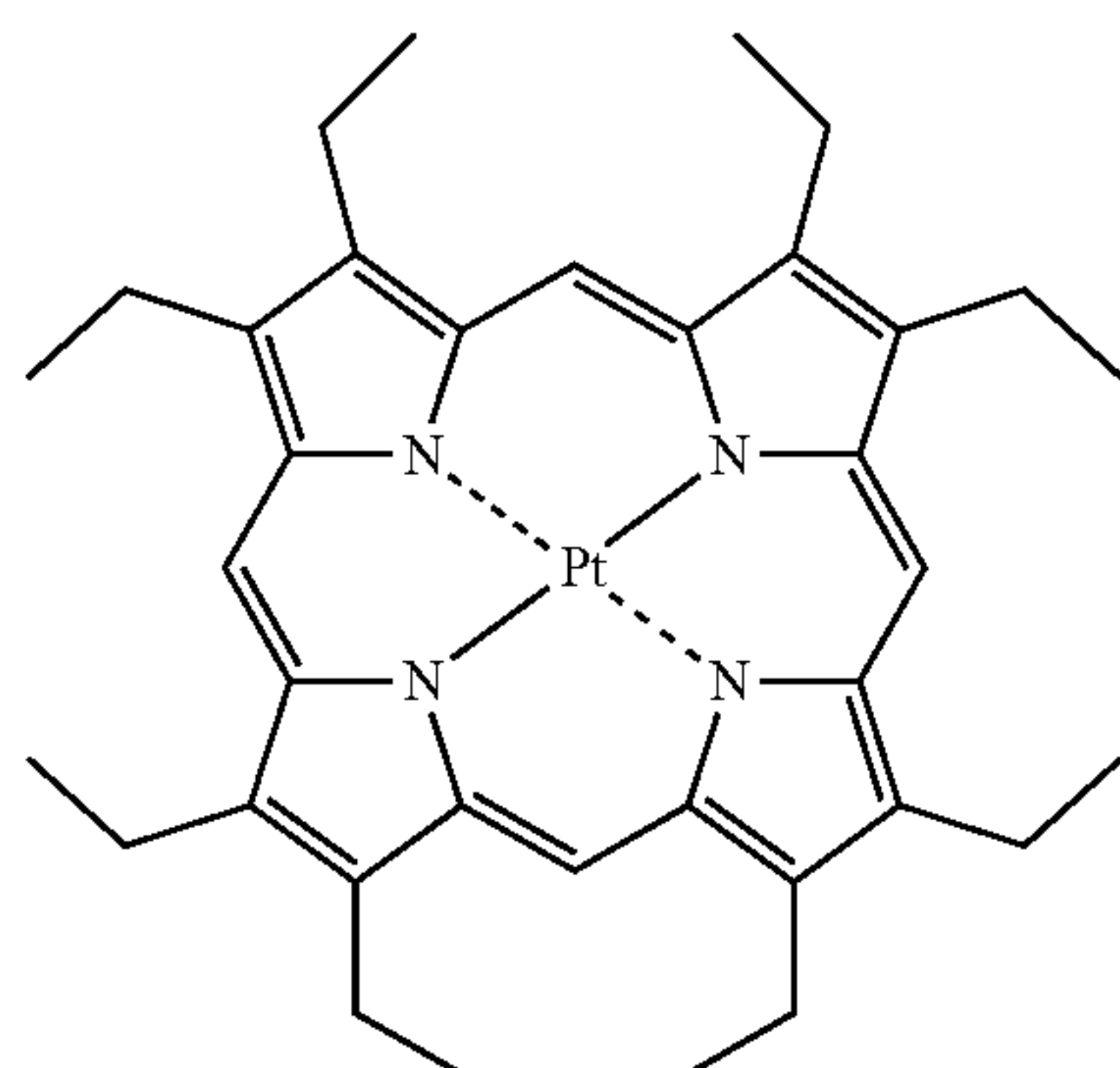
PtOEP
