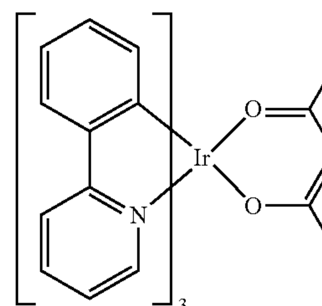
Ir(ppy) 2 (acac)
