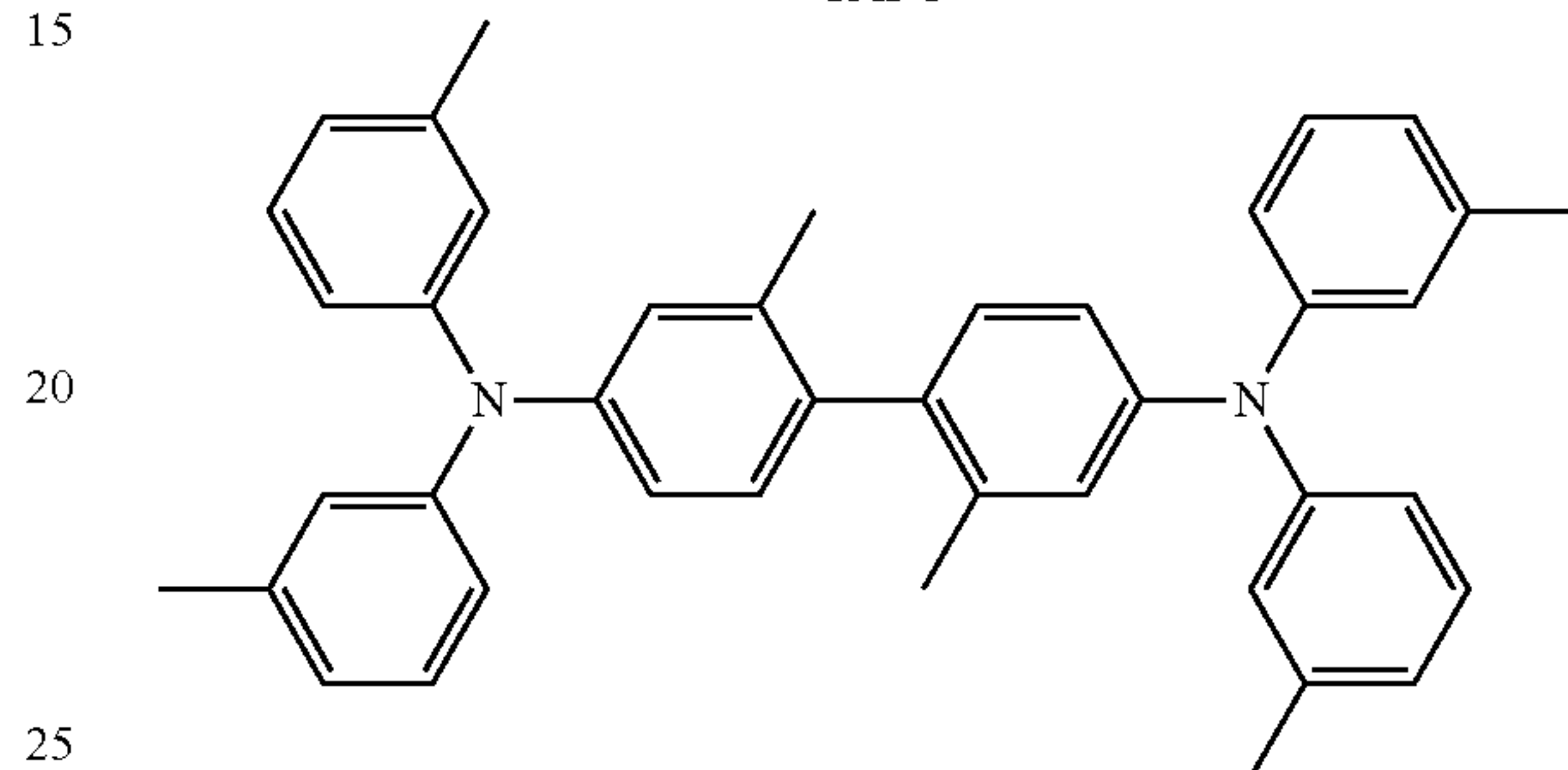
HMTPD
