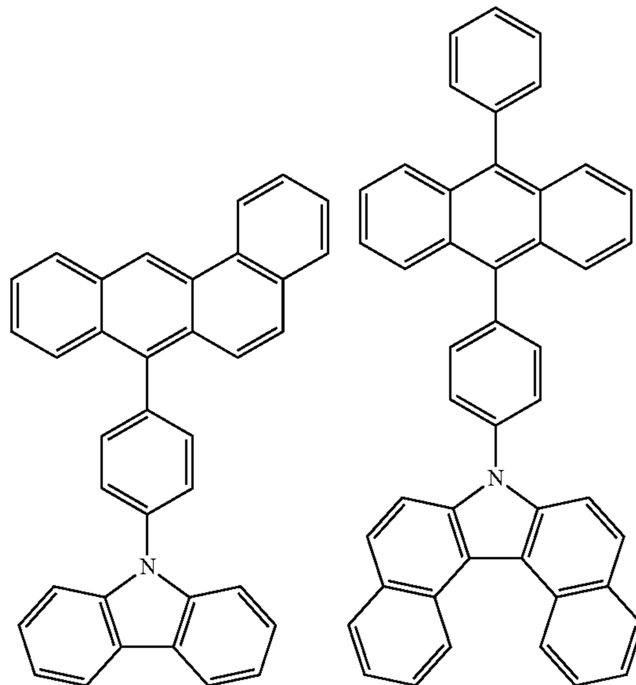
7CzPaBA
