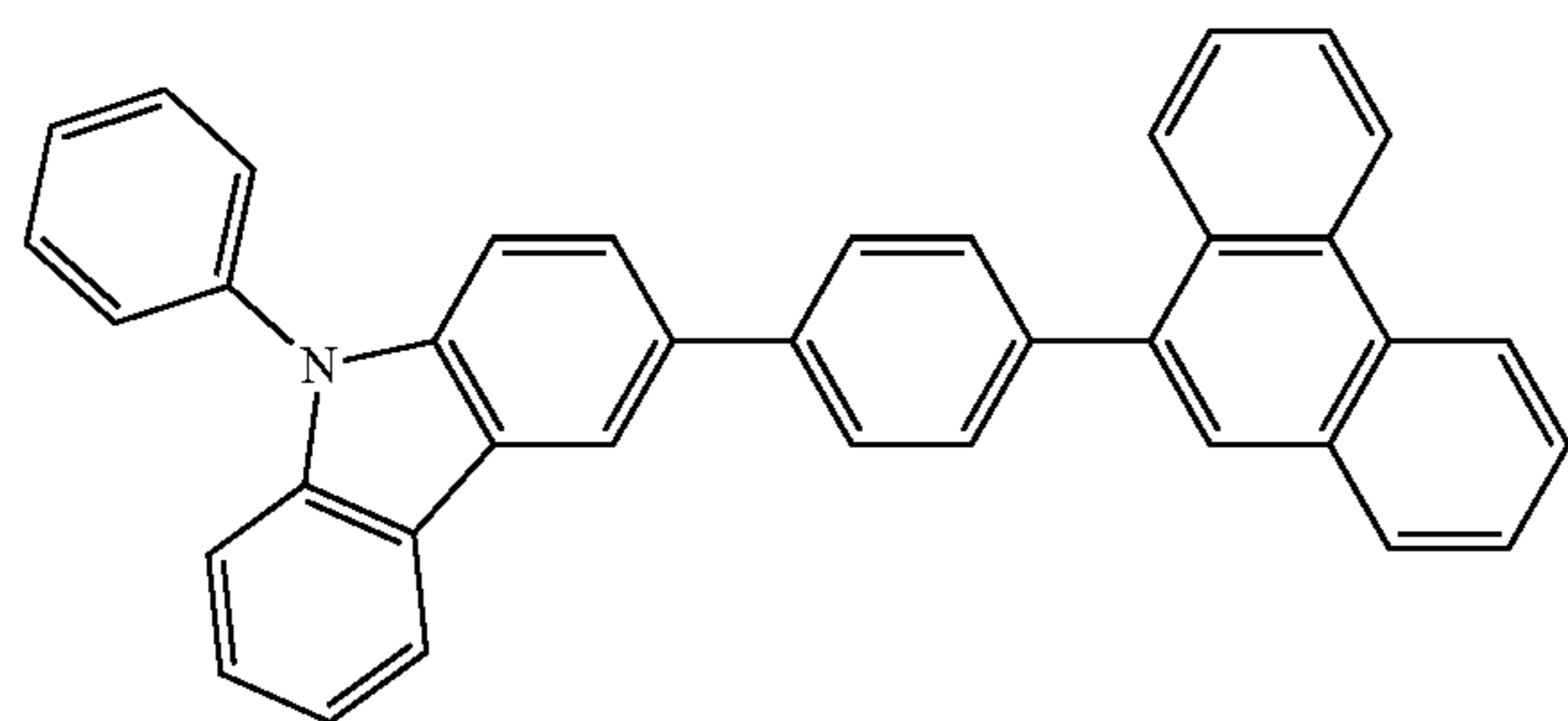
PCPPn
