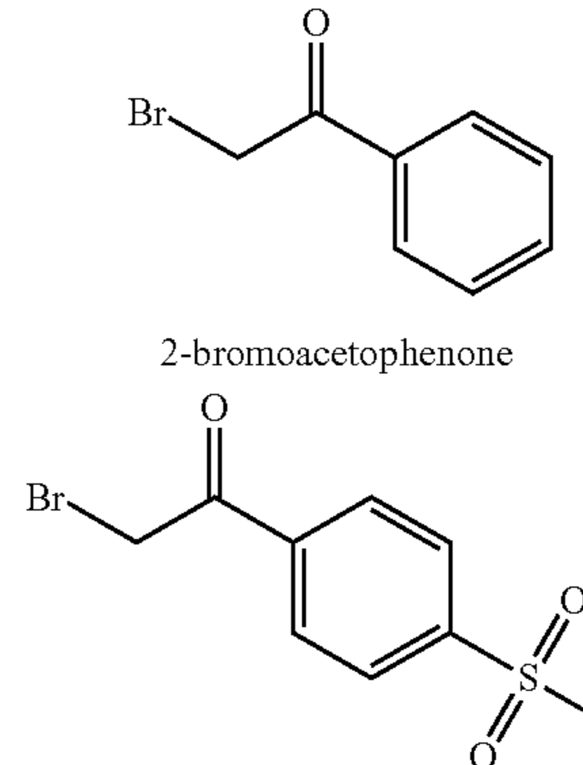
2-Bromo-1-[4-(methylsulfonyl)phenyl]-1-ethanone
