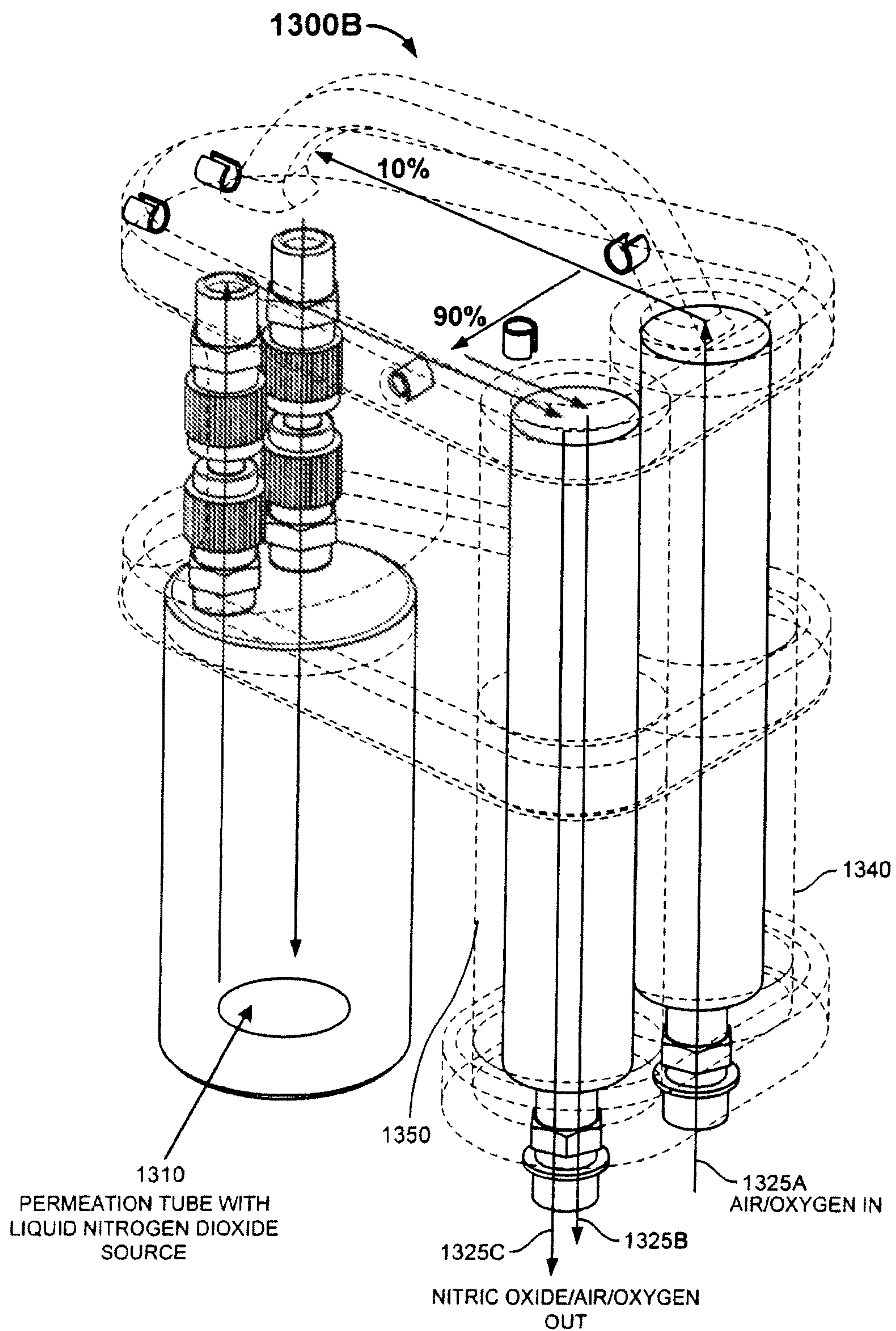
FIG. 13B
