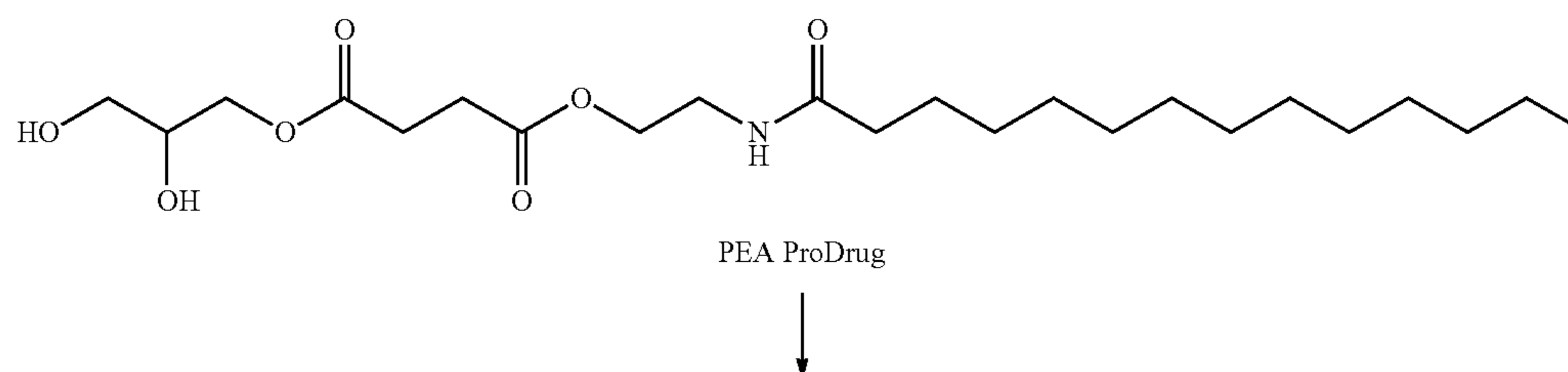
Scheme 20.
