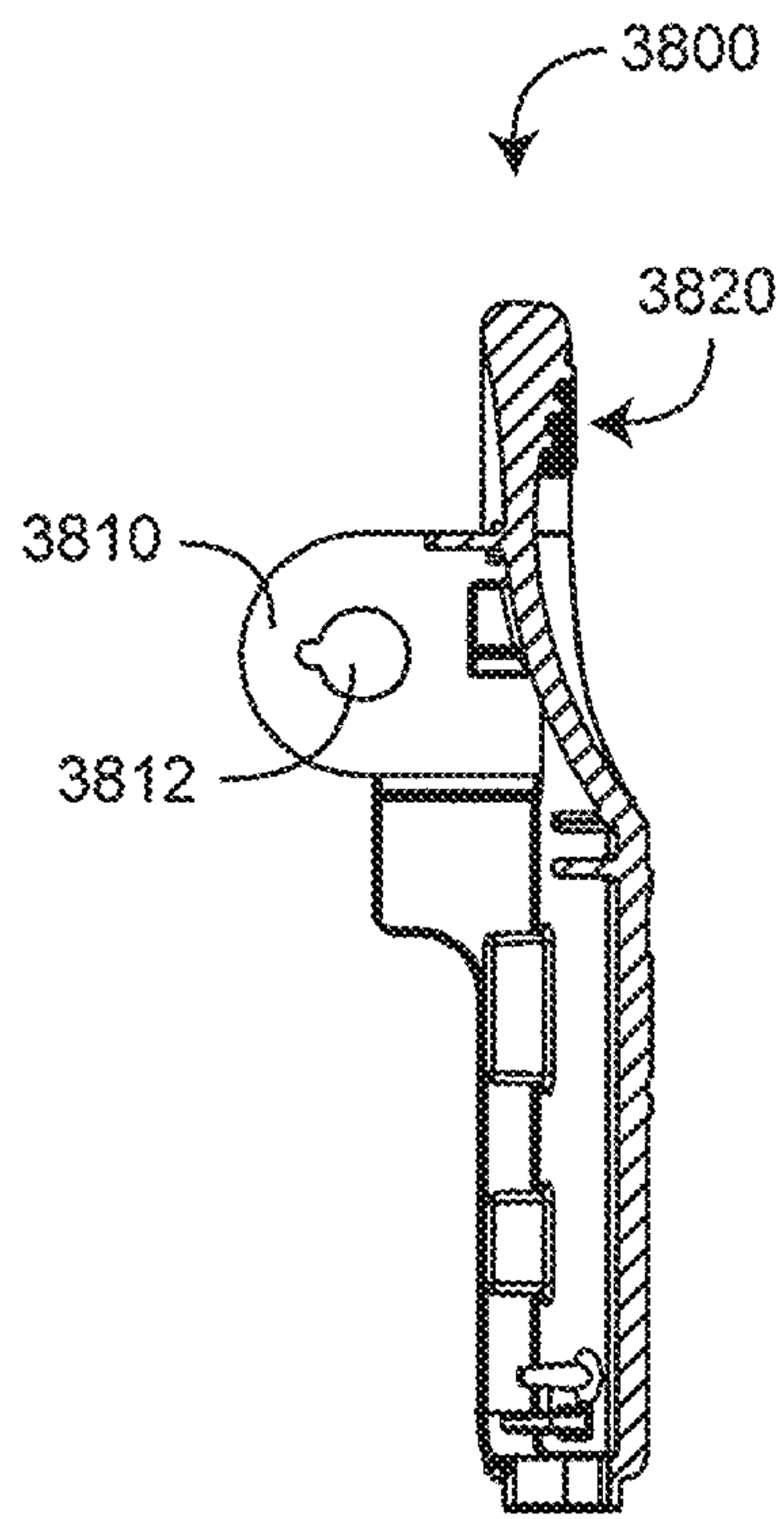
SECTION A-A
