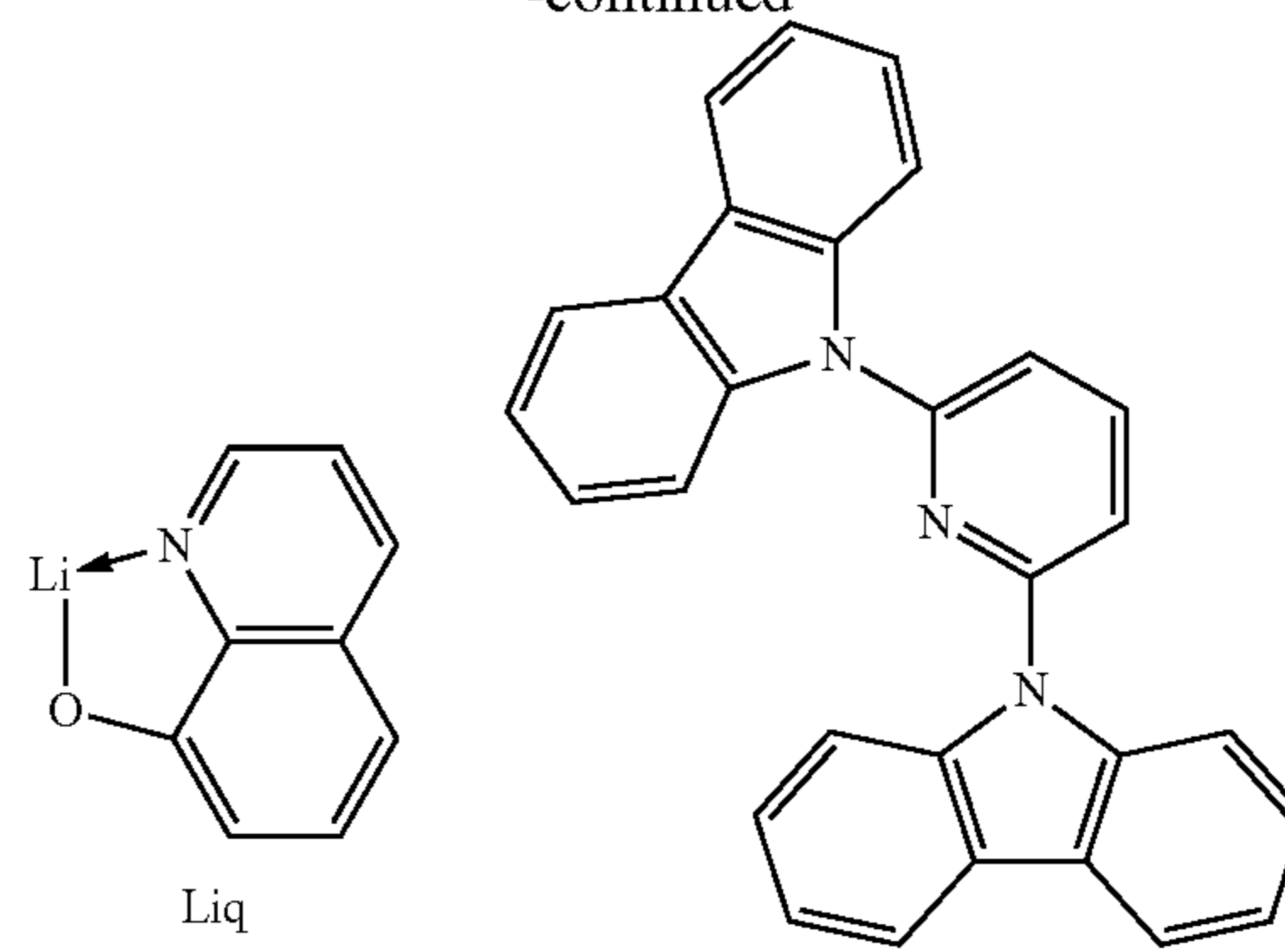
PYD2Cz
