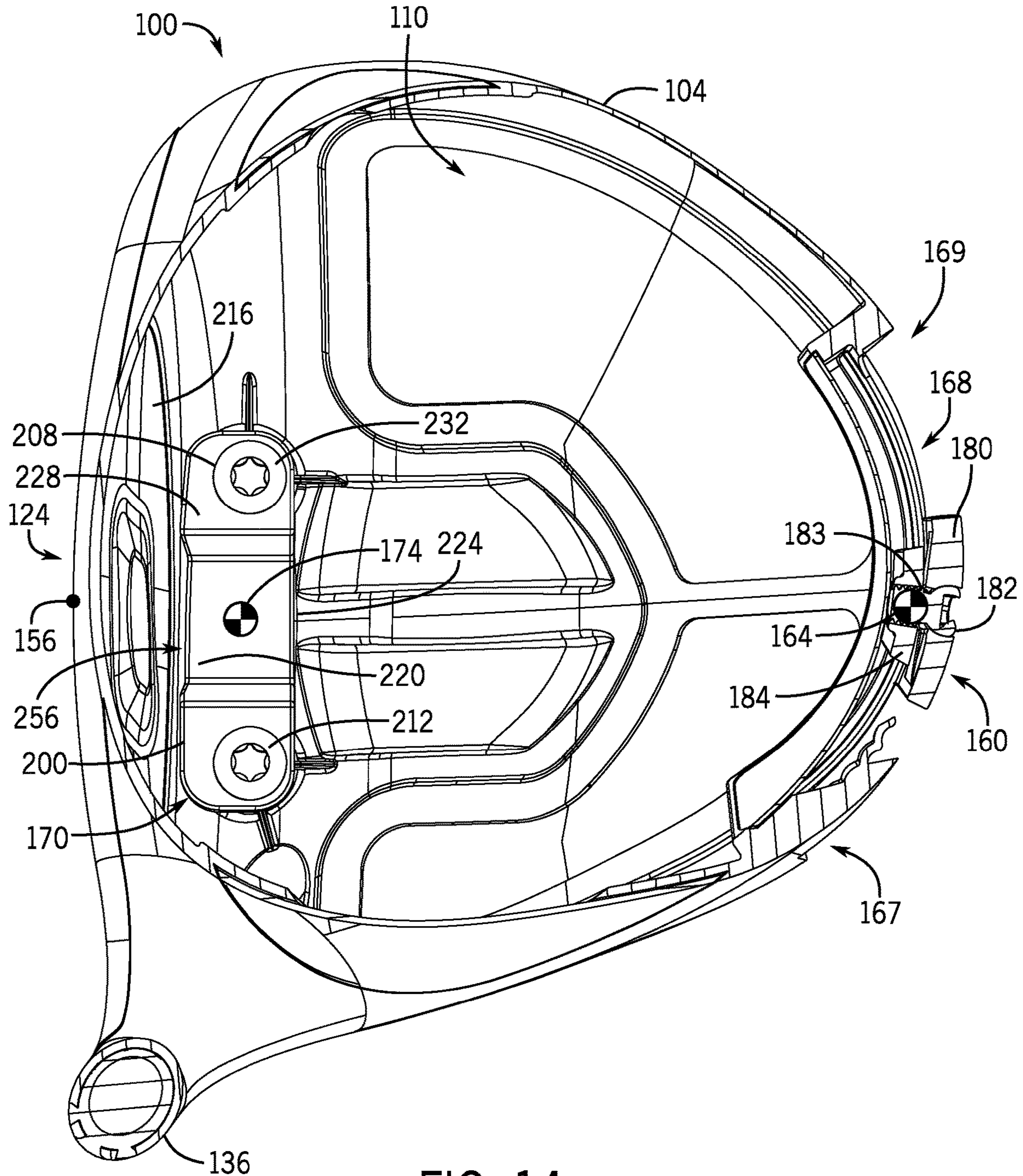
FIG. 14
