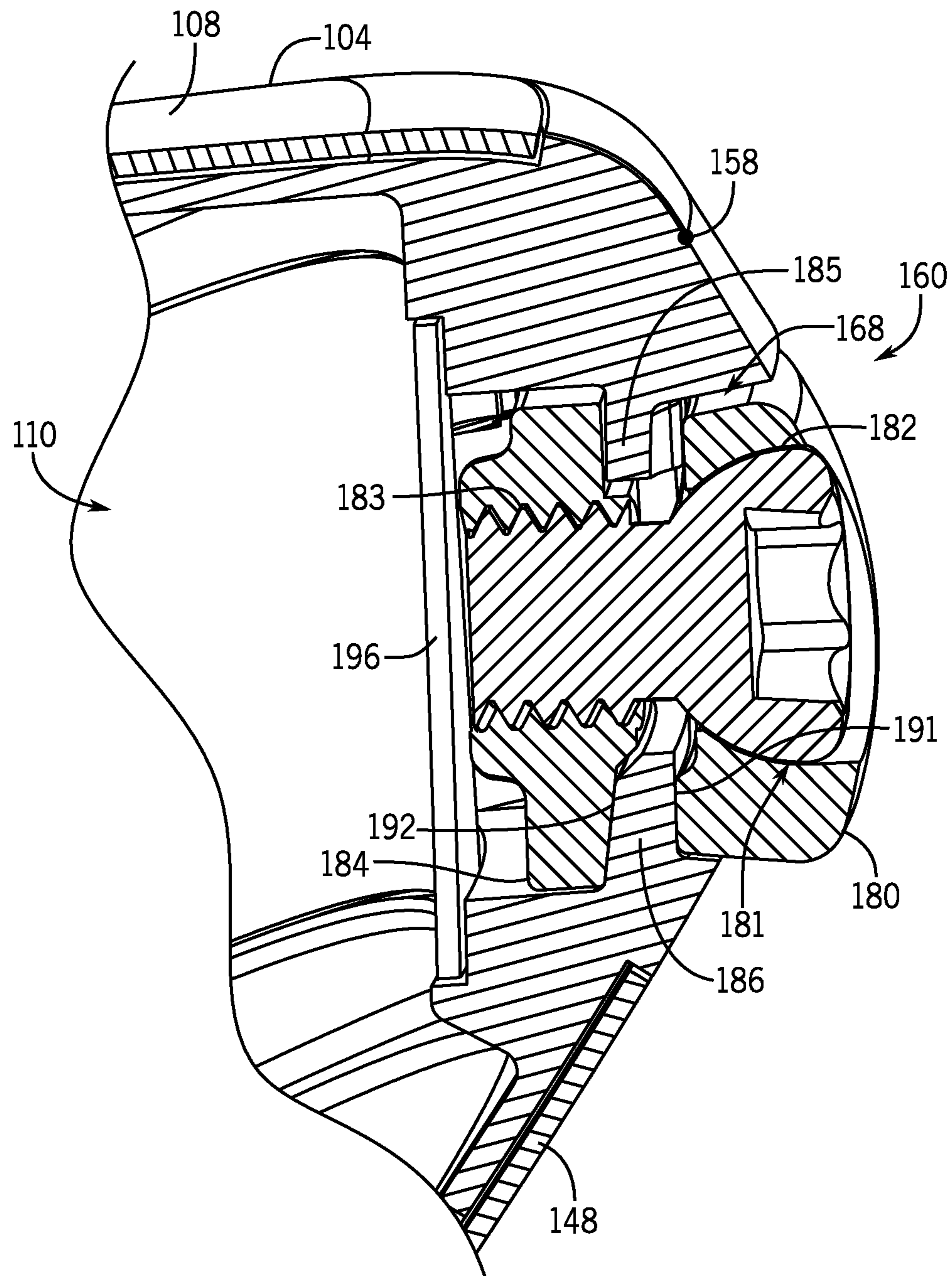
FIG. 12B
