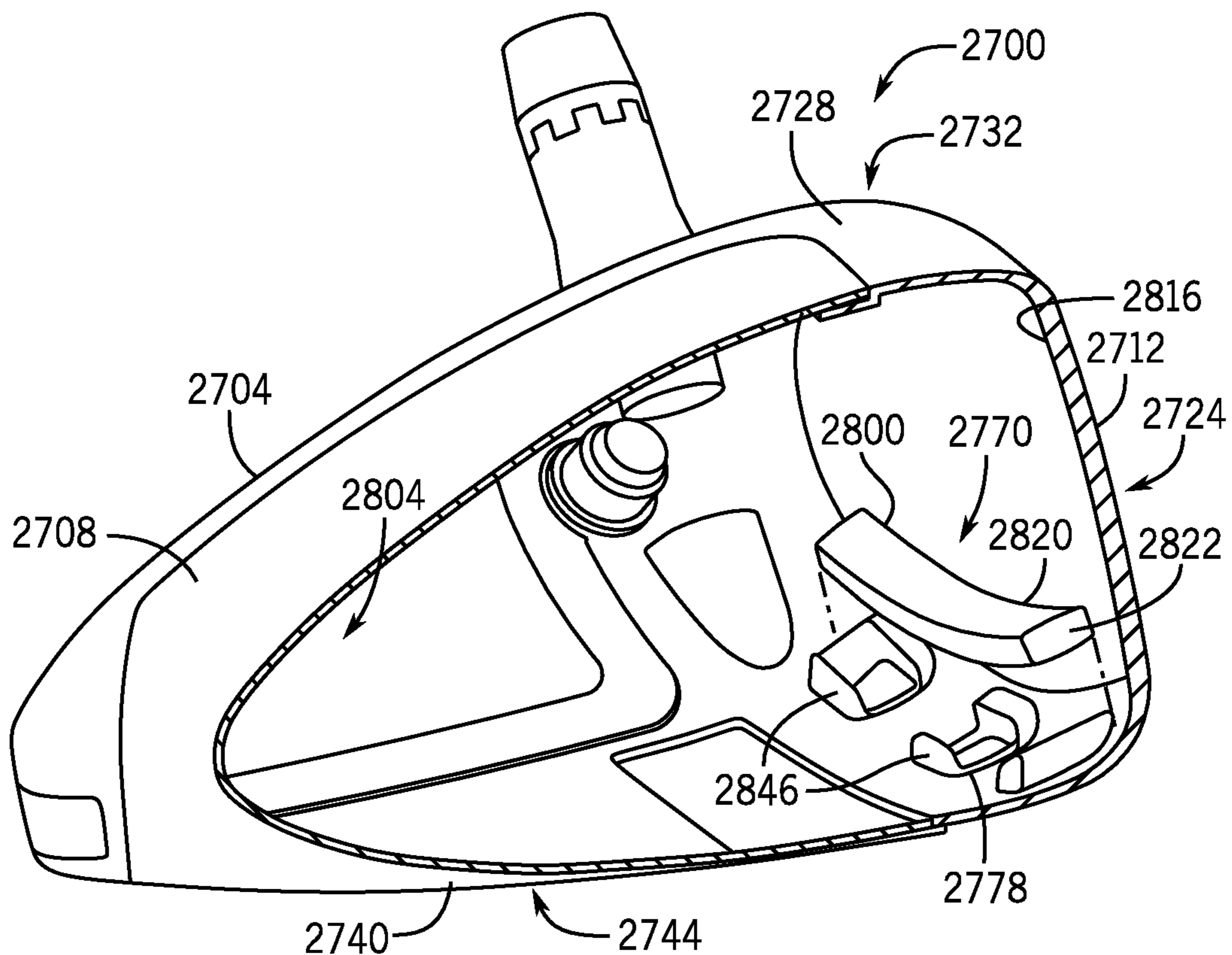
FIG. 27
