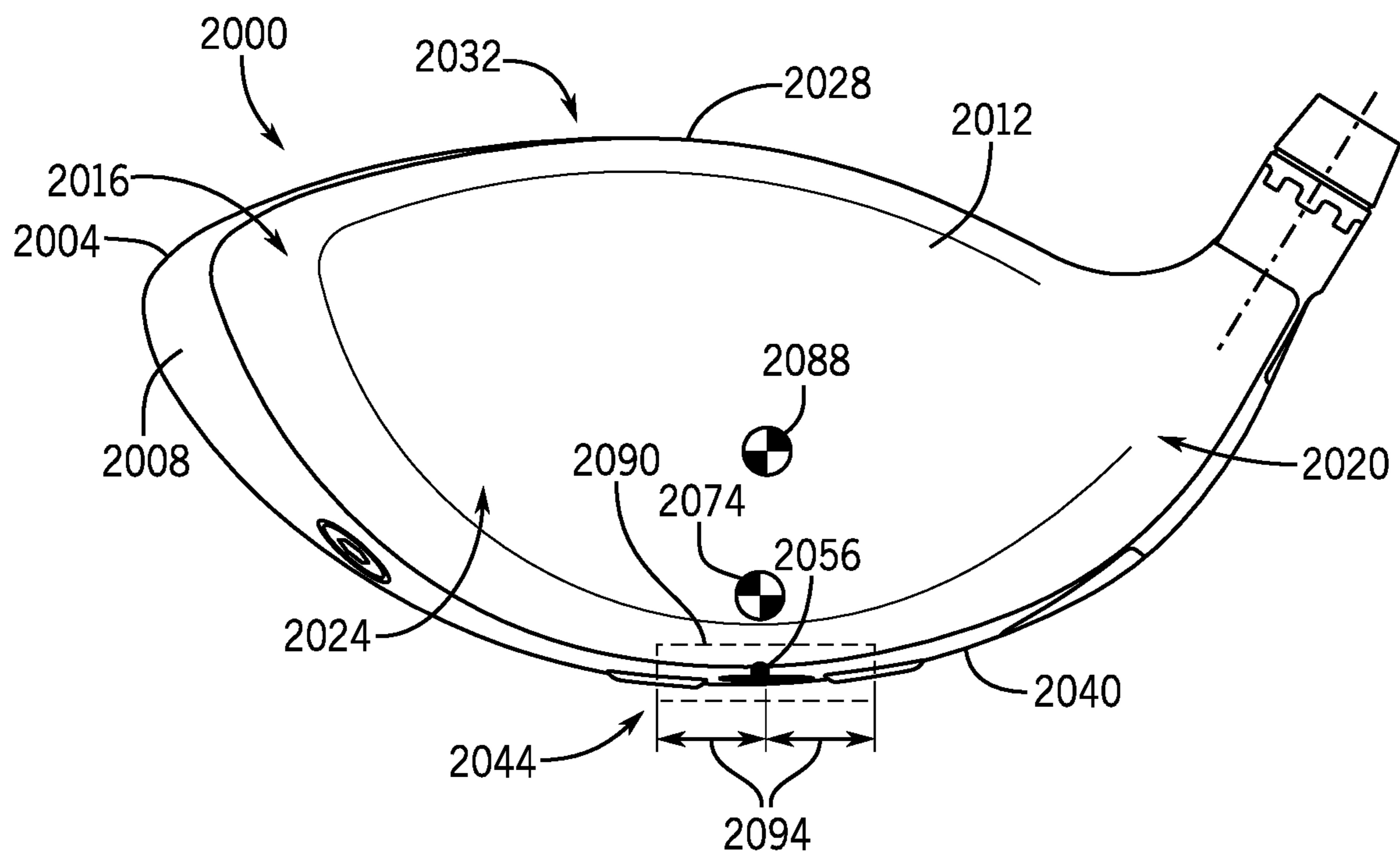
FIG. 20
