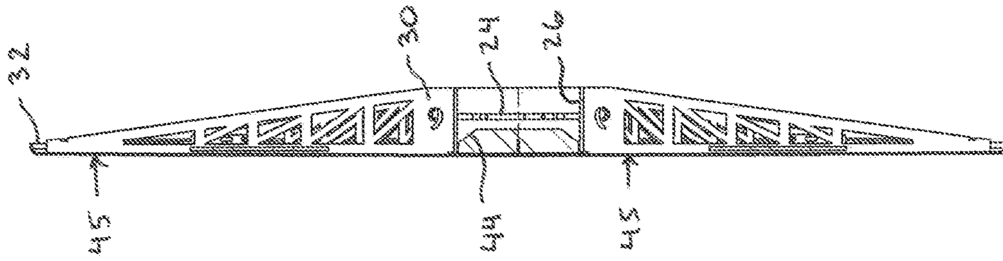
SECTION A-A
