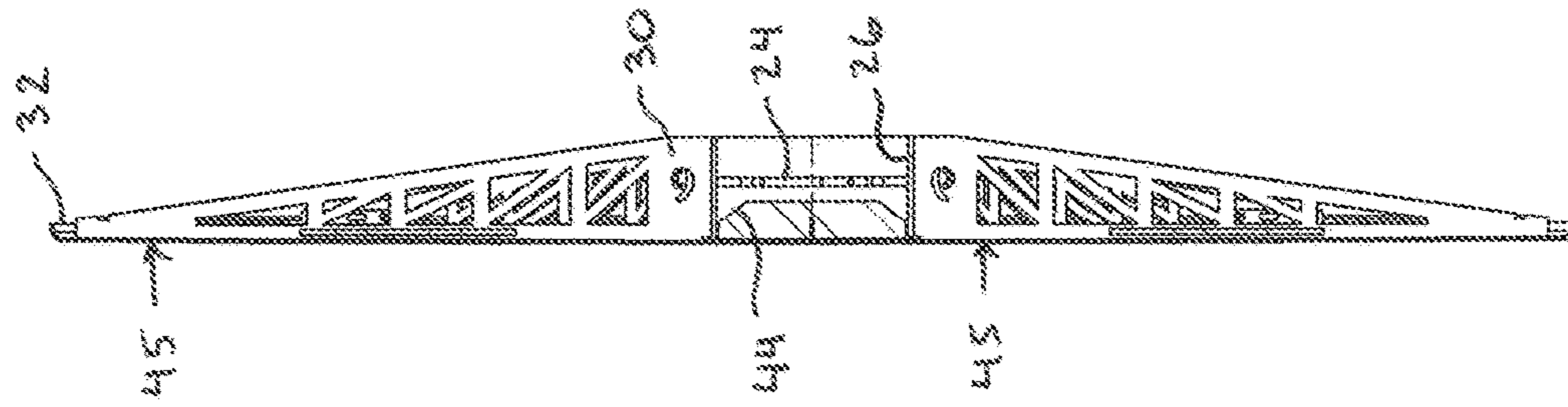
SECTION A-A
