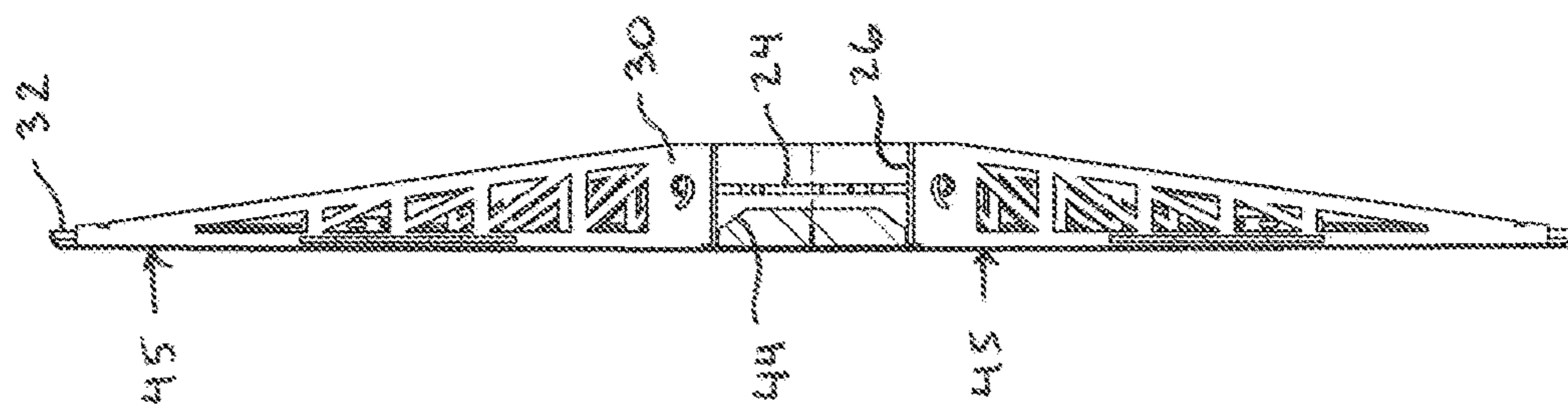
SECTION A-A
