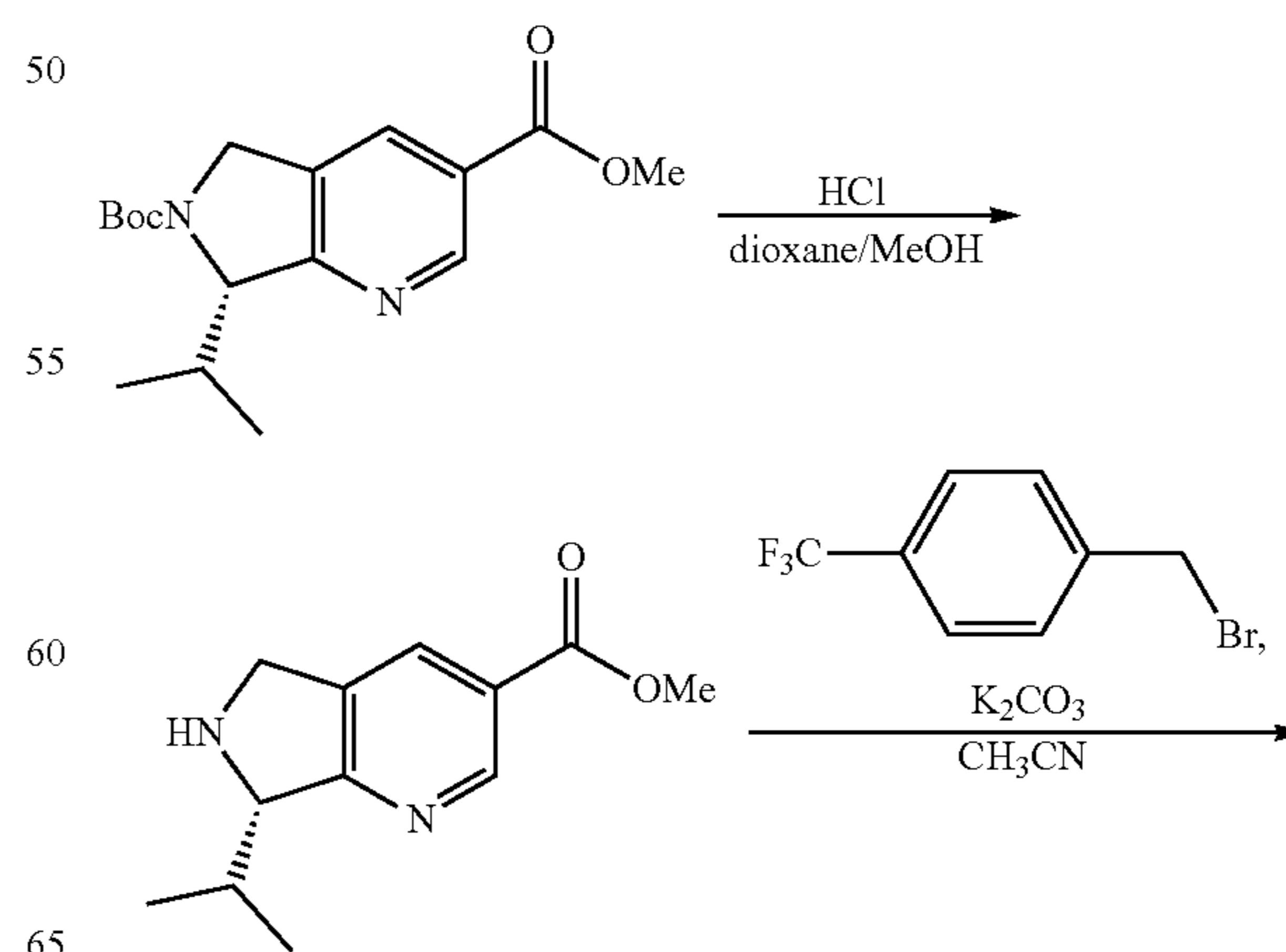
Scheme 14.
