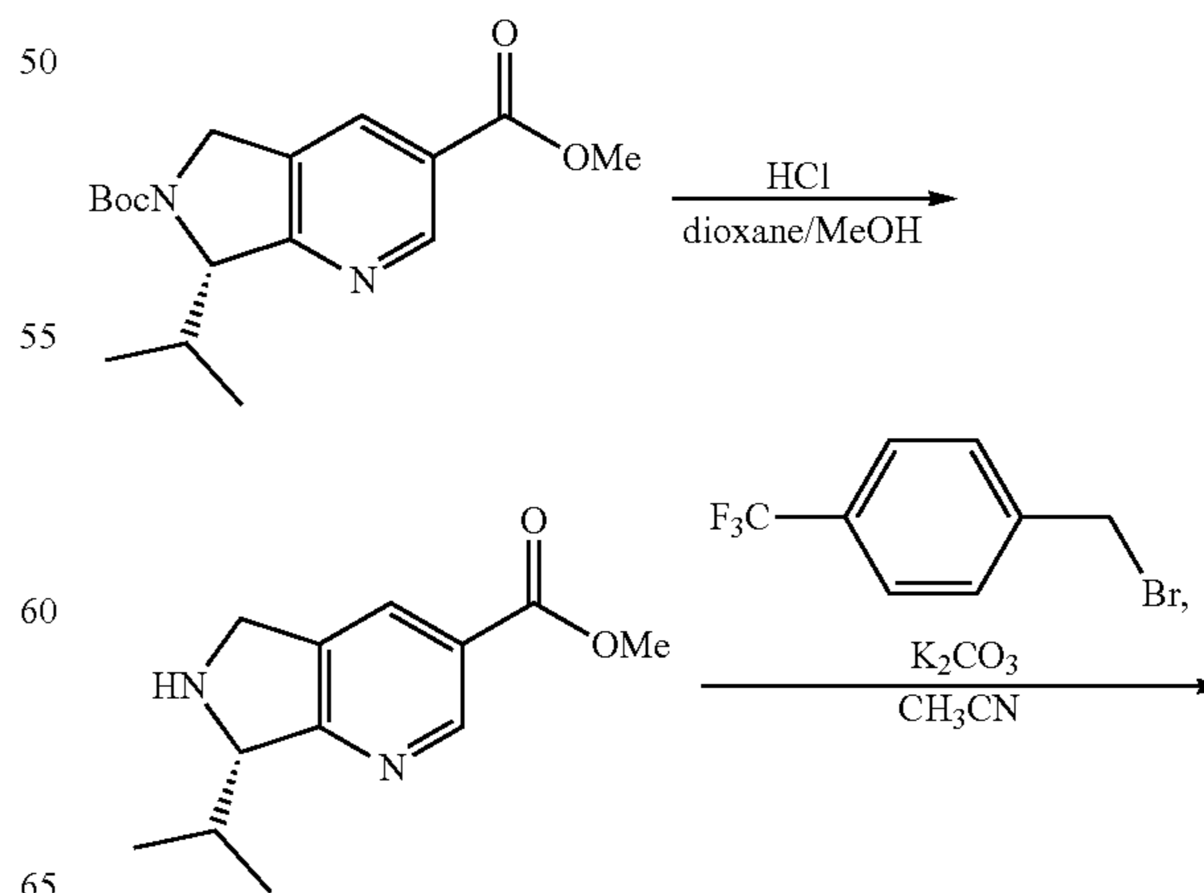
Scheme 14.
