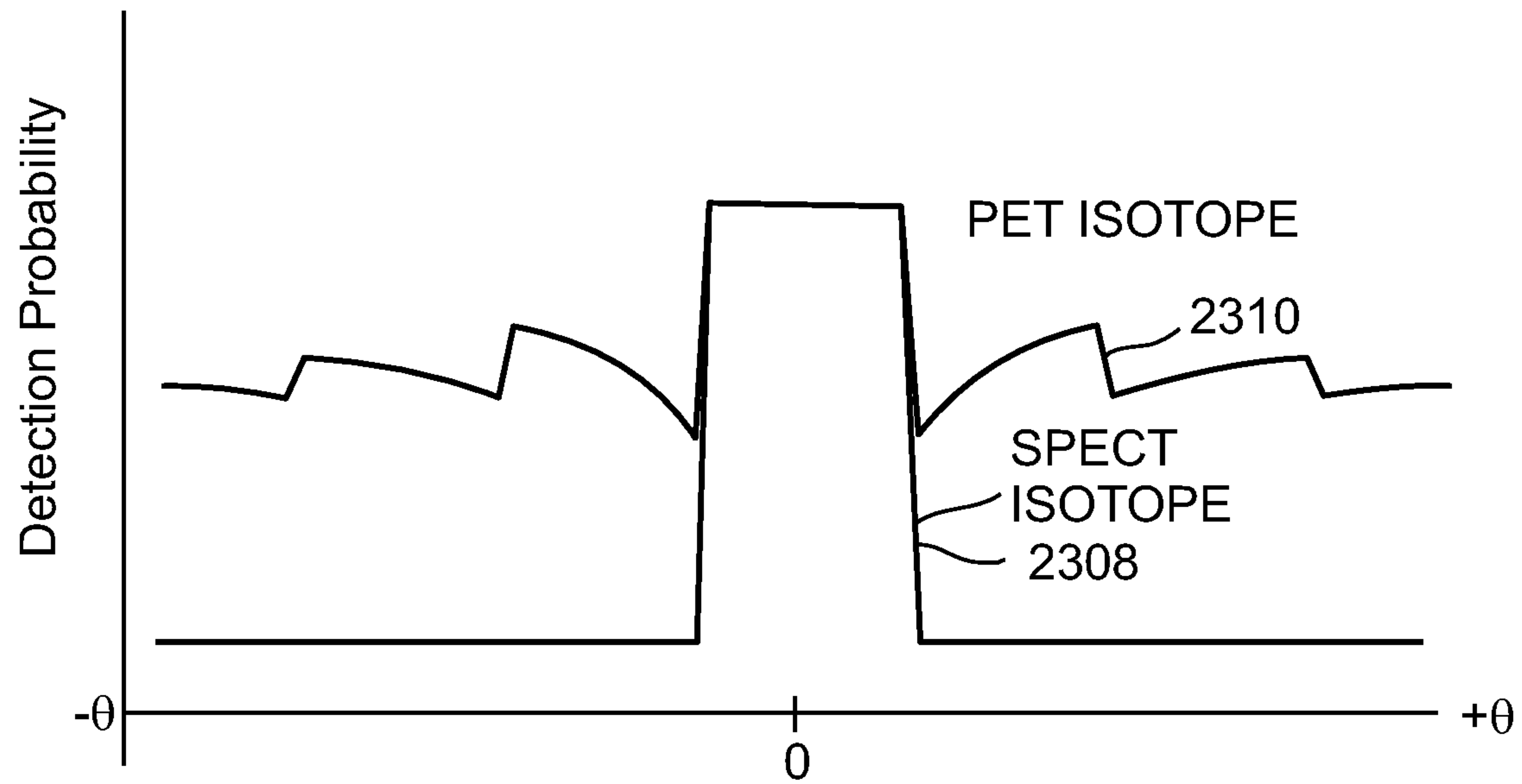
FIG. 23A
