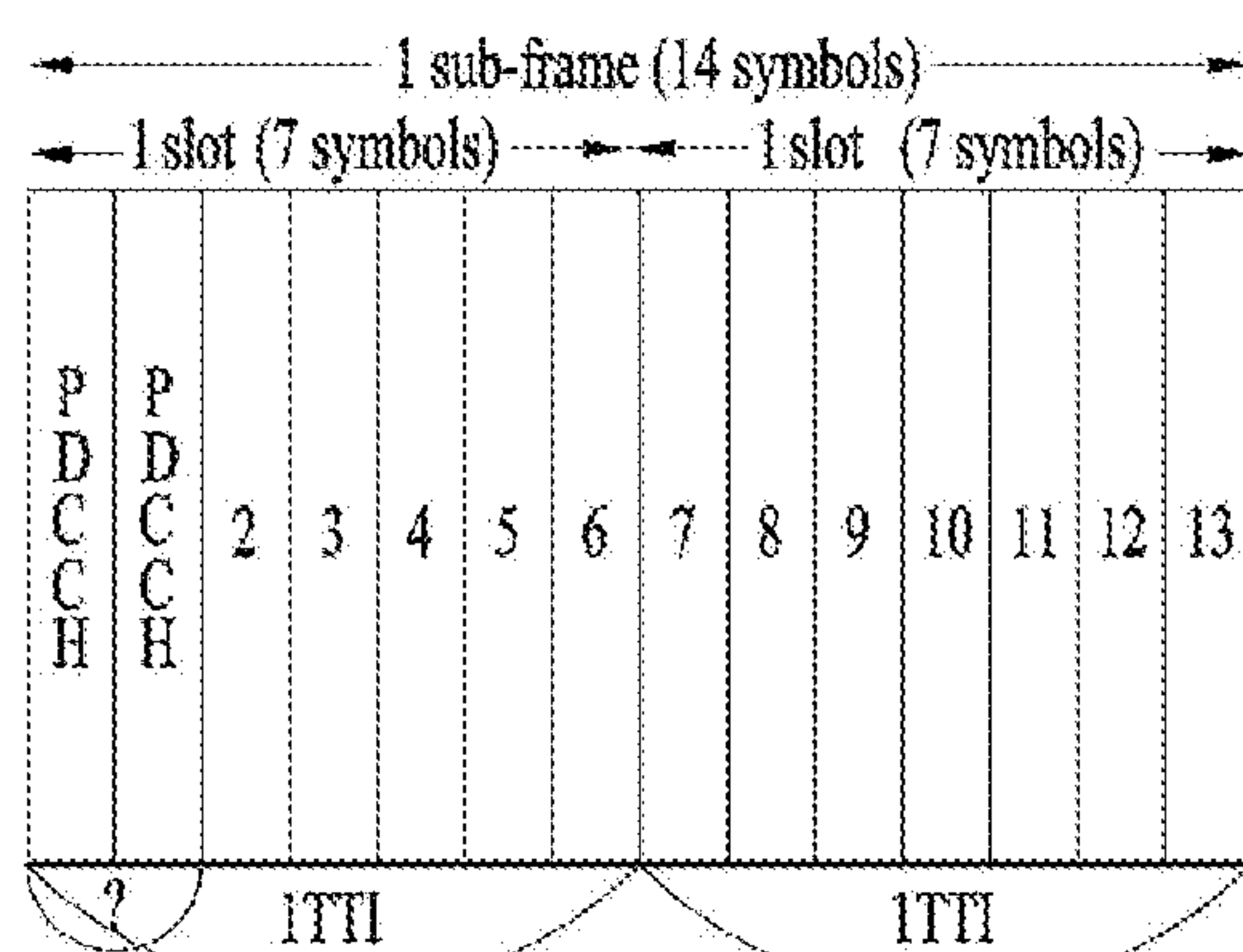
(d) 7 symbol TTI DL structure
