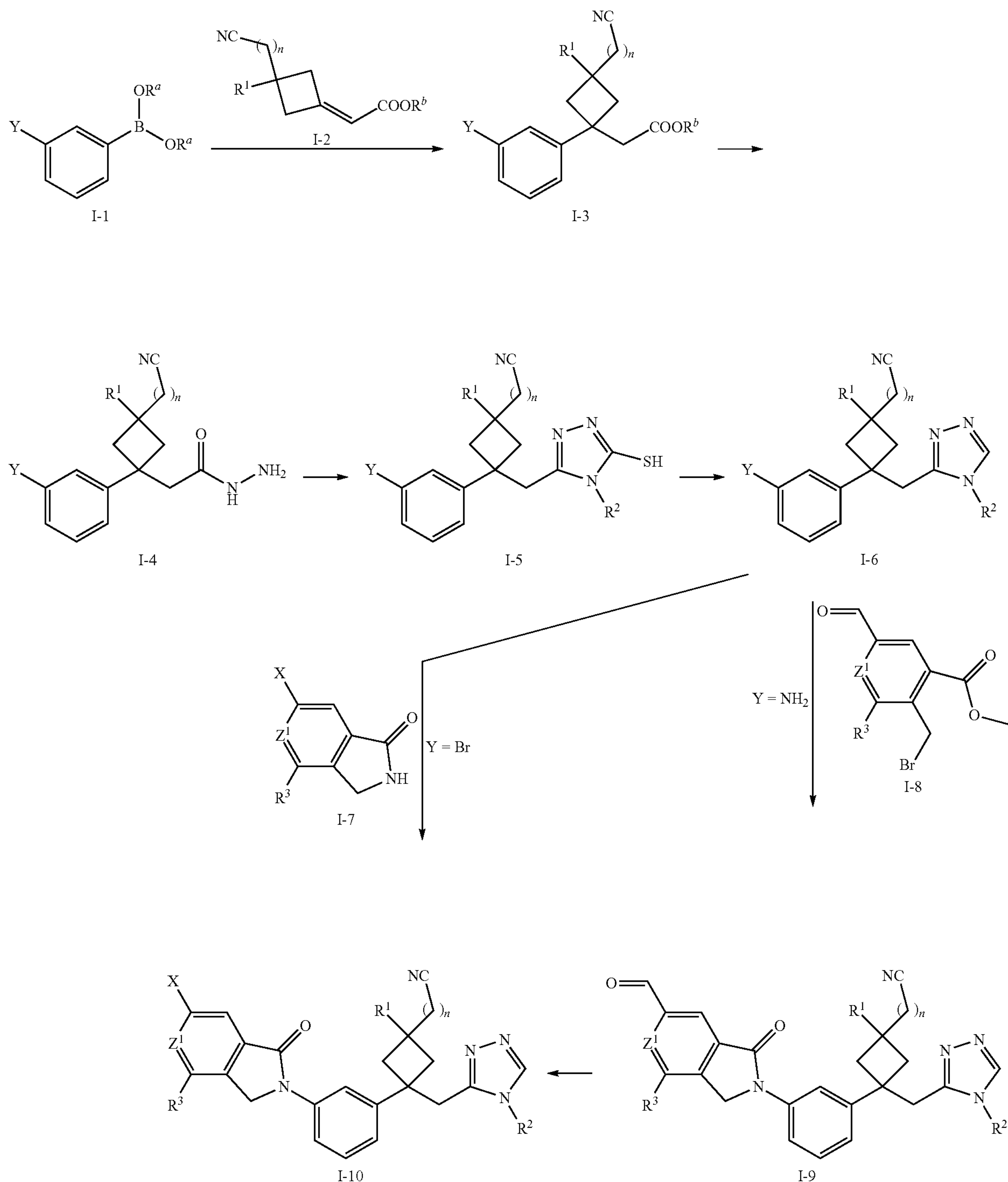
Scheme I.
