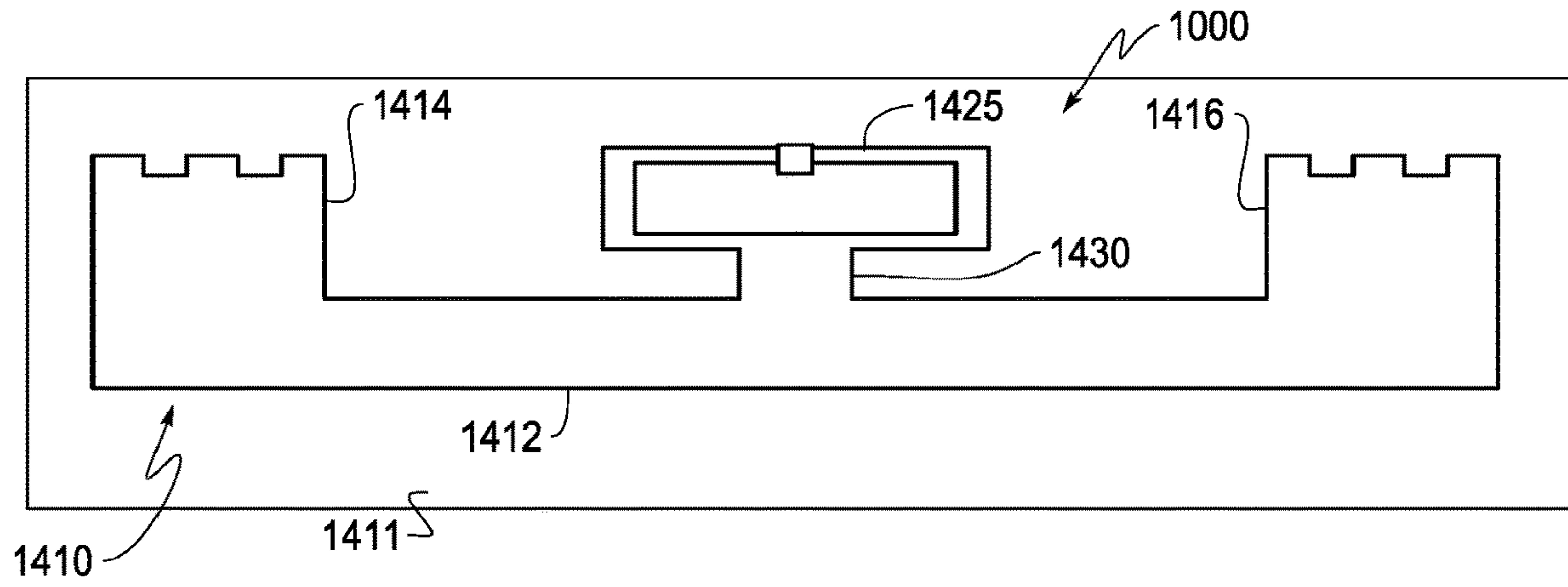
FIG. 14
