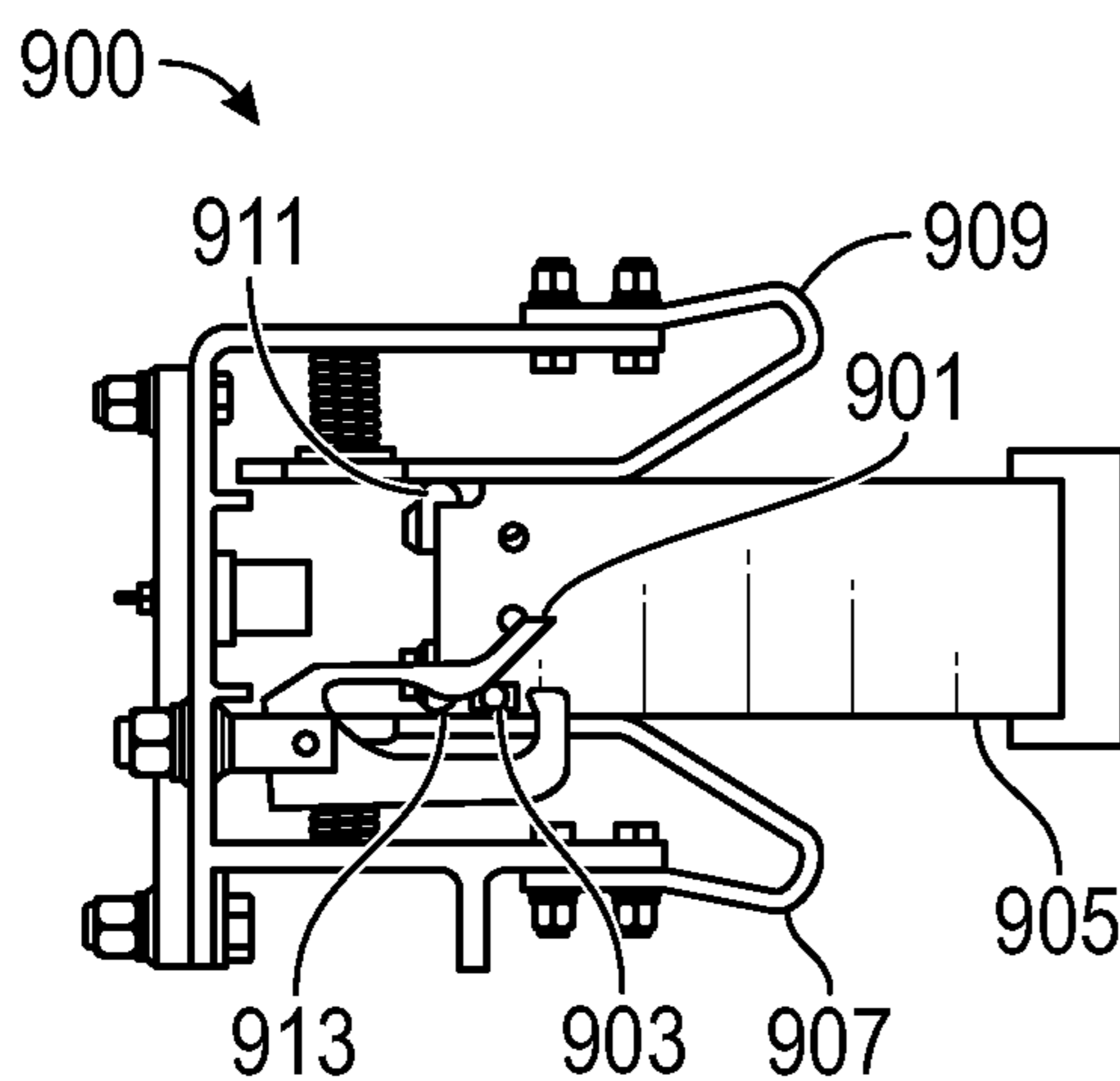
FIG. 9C
