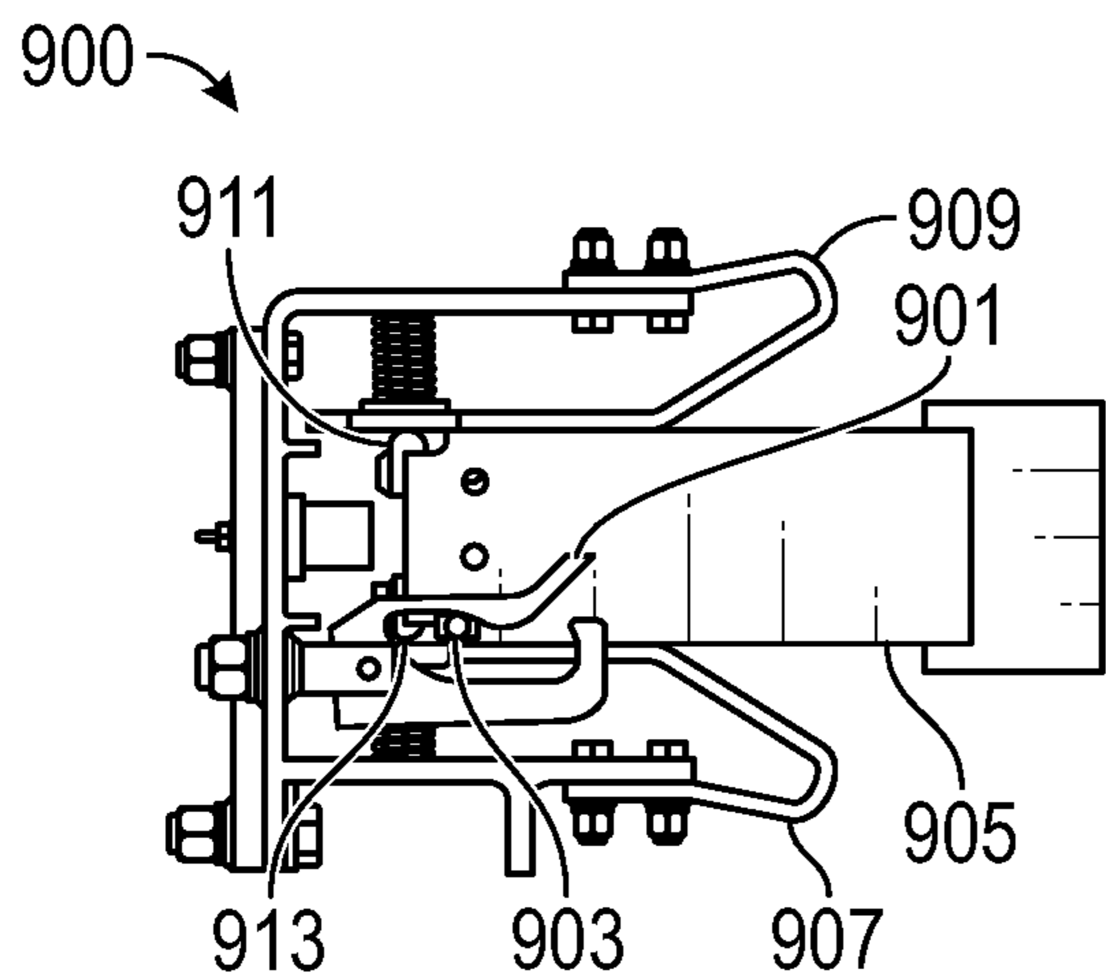
FIG. 9A
