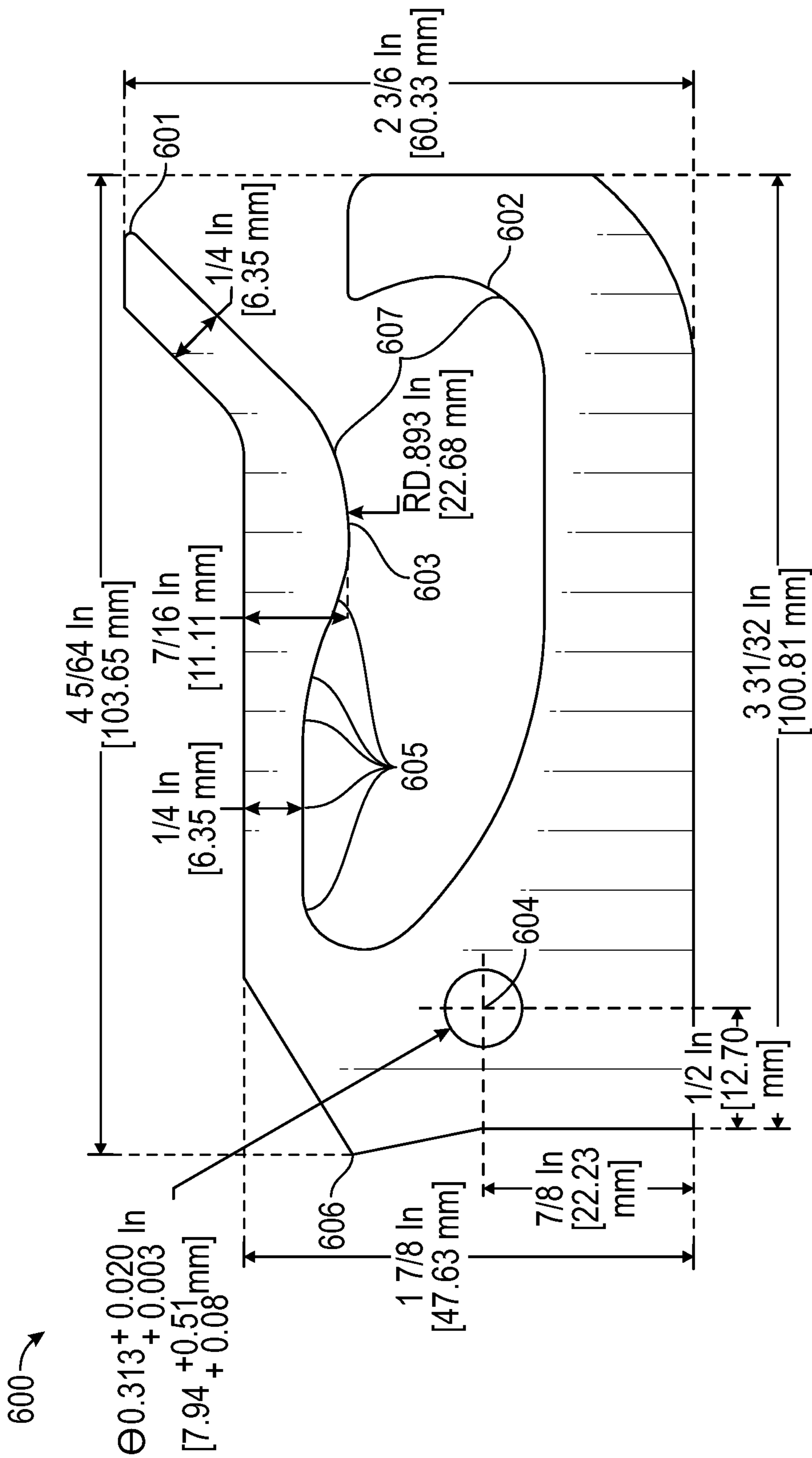
FIG. 6A
