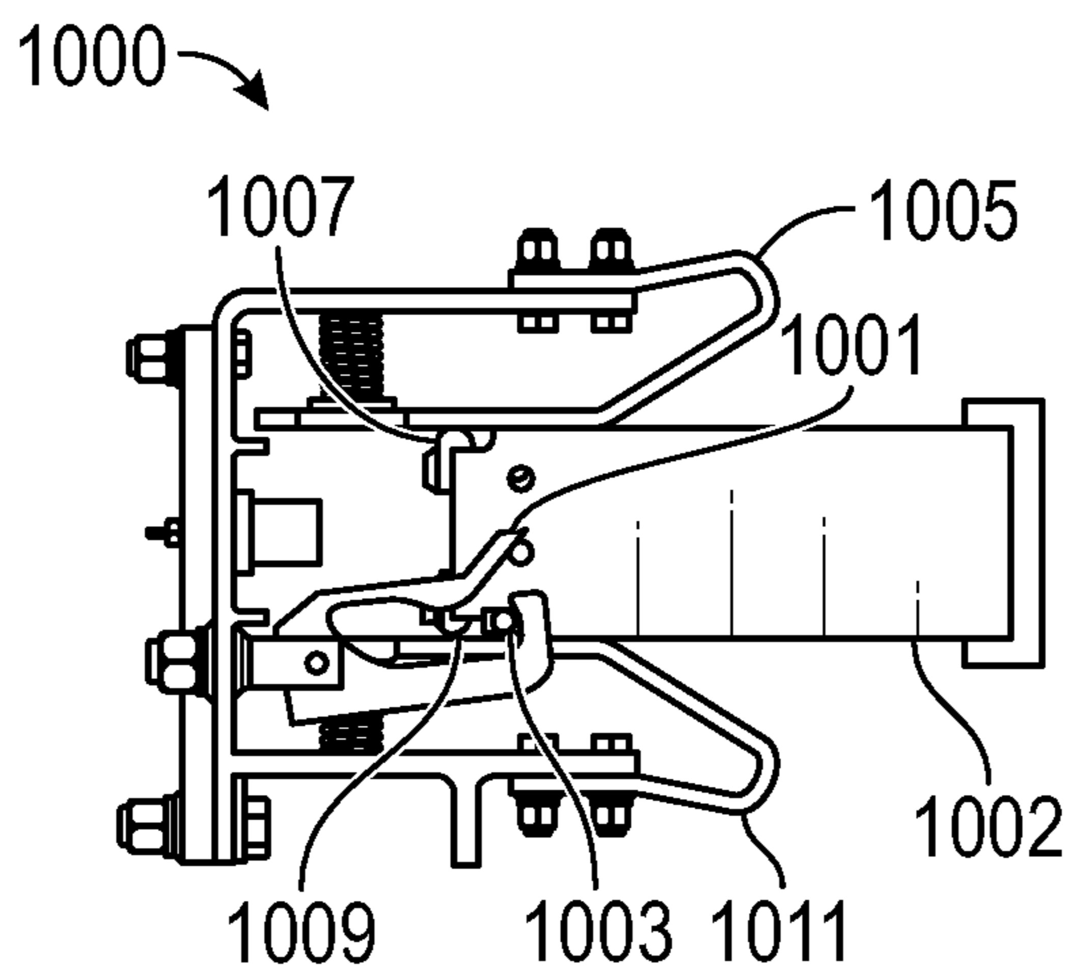
FIG. 10E
