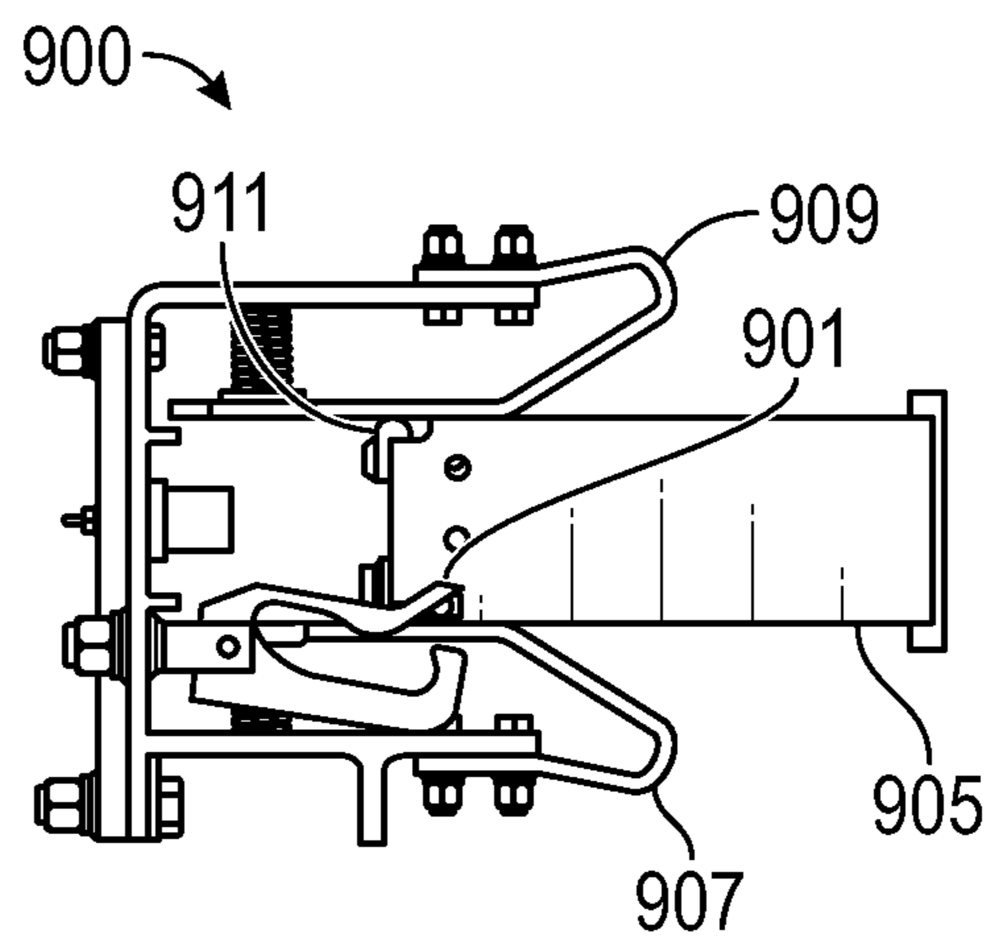
FIG. 9D
