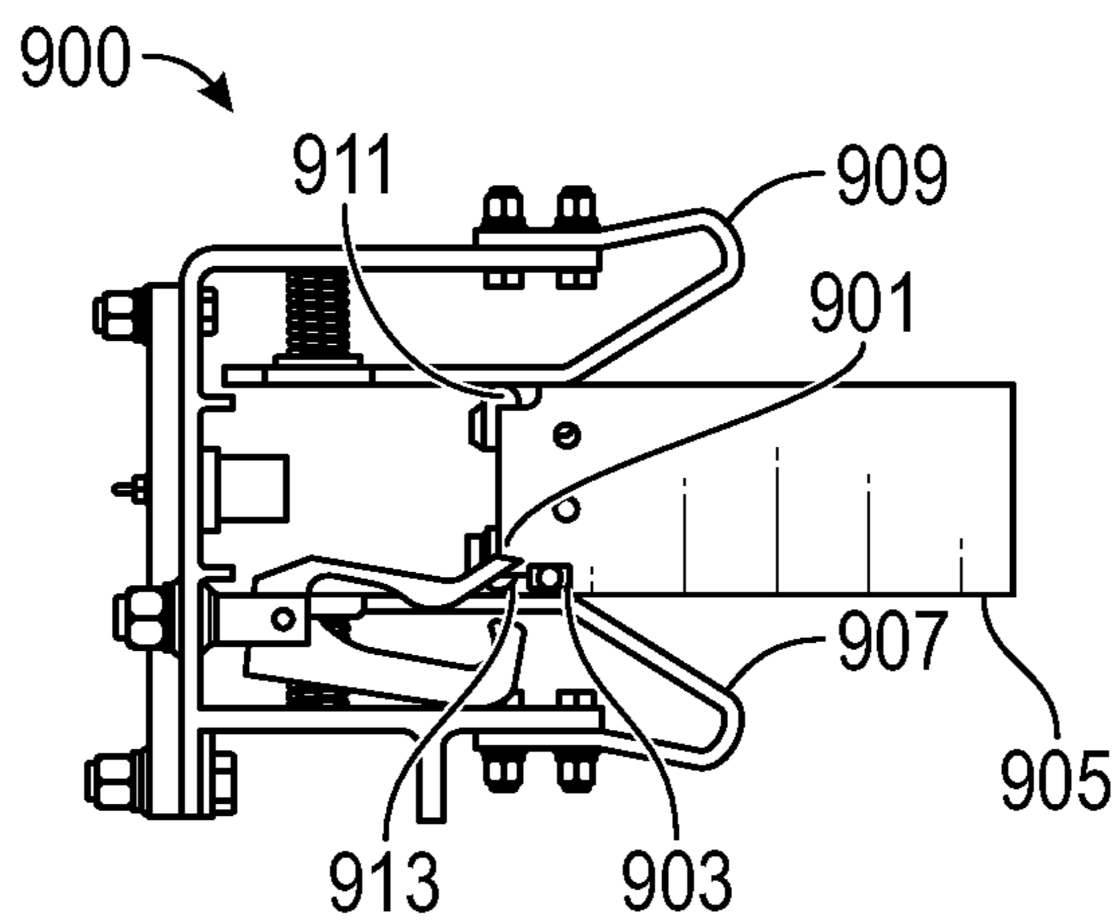
FIG. 9E
