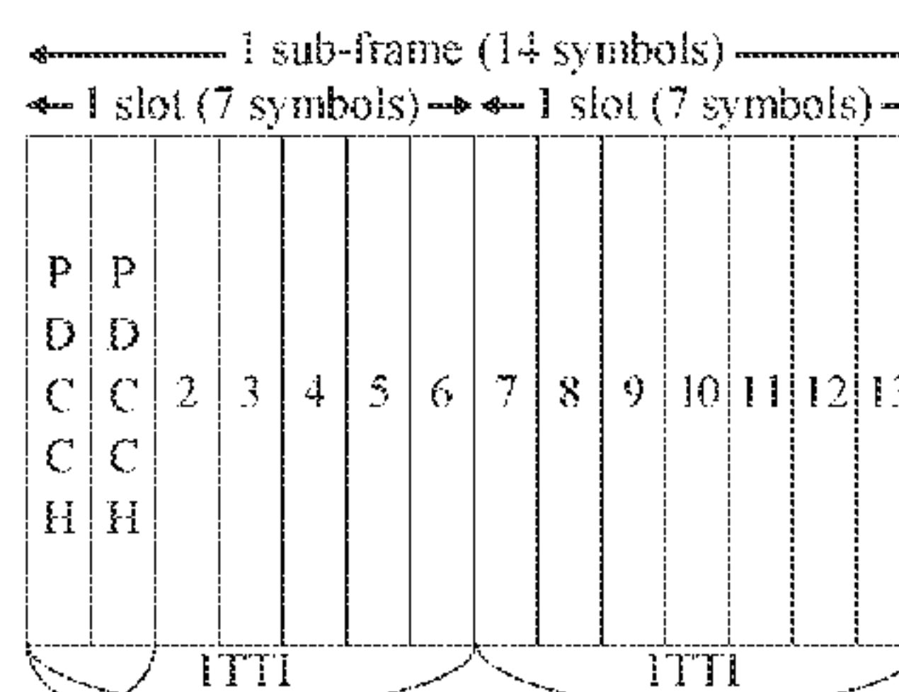
(d) 7 symbol TTI DL structure
