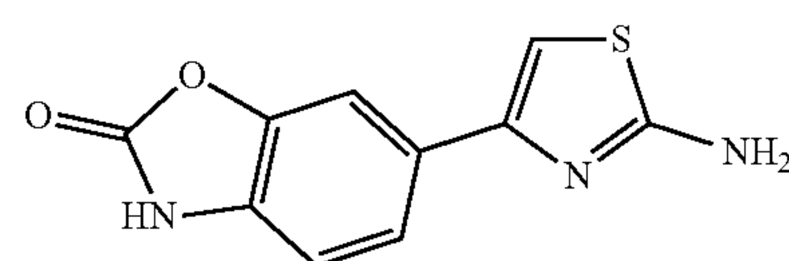
6-(2-aminothiazol-4-yl)benzo[d]oxazol-2(3H)-one
