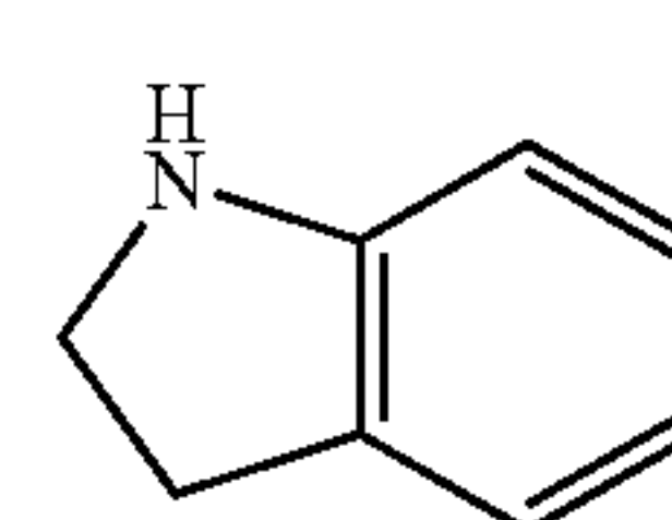
indoline
