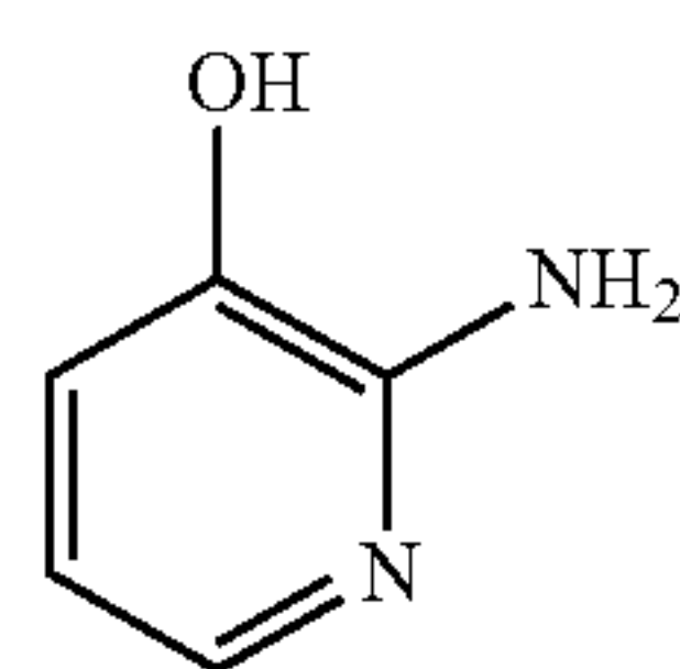
2-aminopyridin-3-ol
