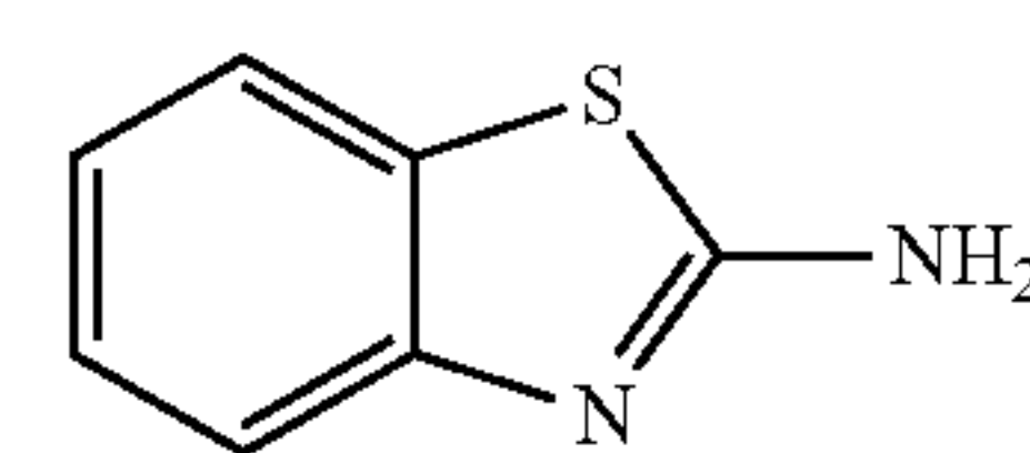
benzo[d]thiazol-2-amine
