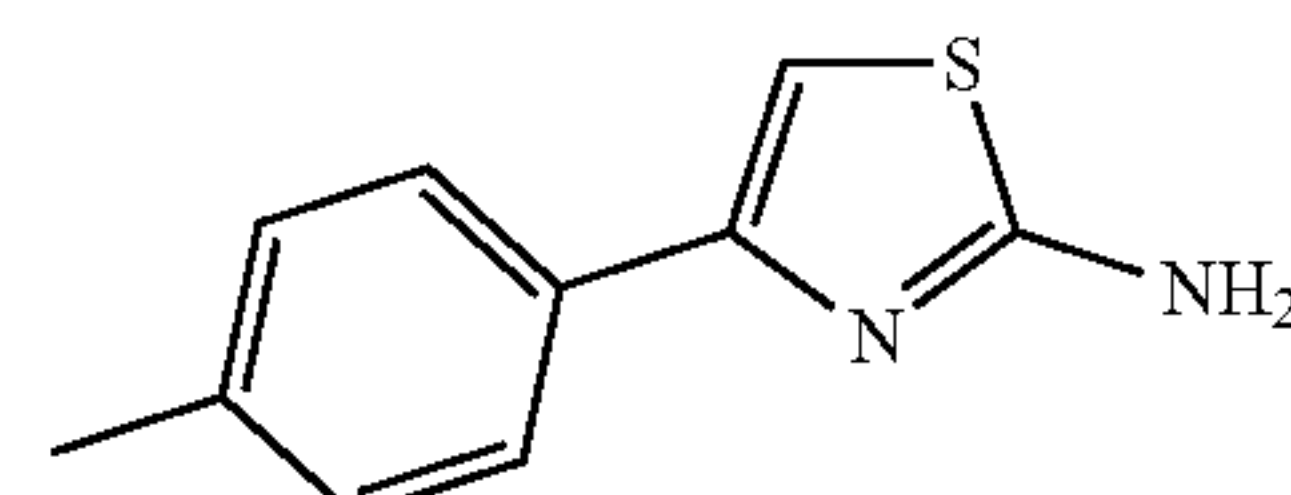
4-p-tolylthiazol-2-amine
