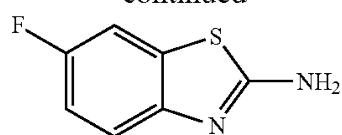
6-fluorobenzo[d]thiazol-2-amine
