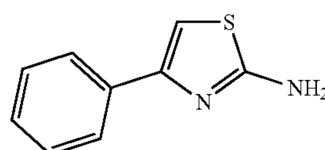
4-phenylthiazol-2-amine
