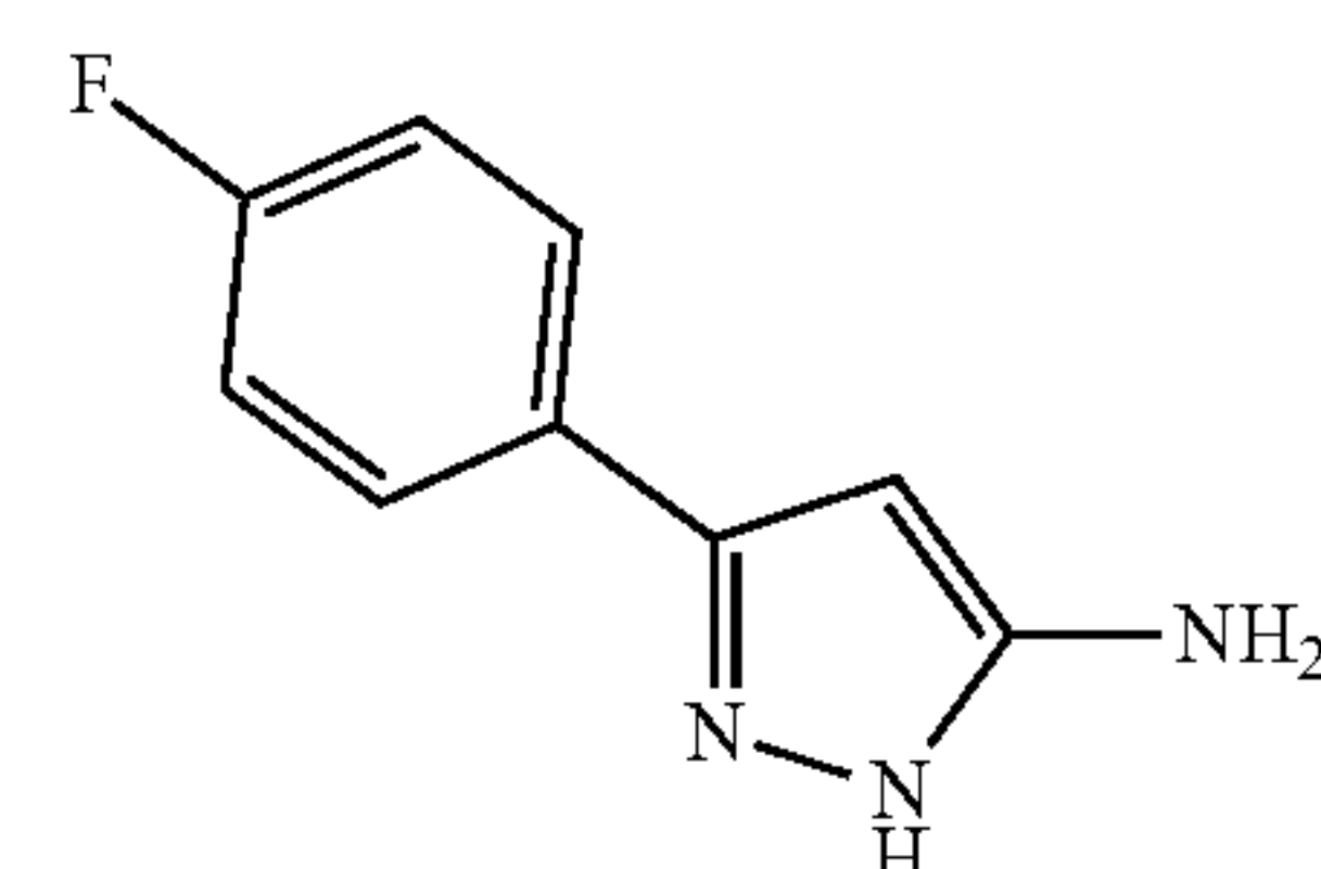
3-(4-fluorophenyl)-1H-pyrazol-5-amine
