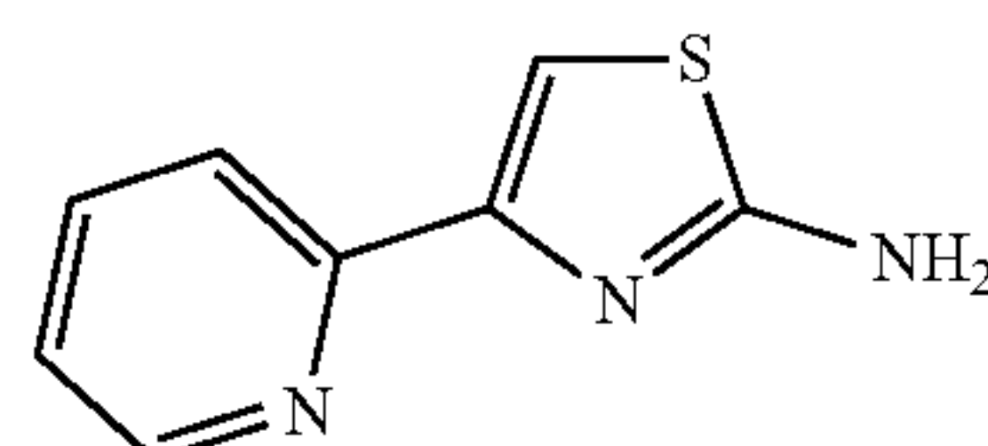
4-(pyridin-2-yl)thiazol-2-amine
