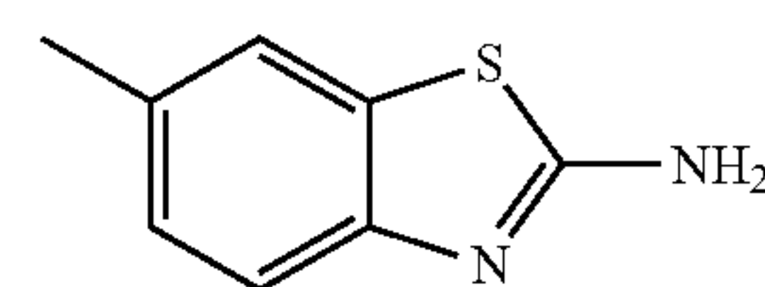
6-methylbenzo[d]thiazol-2-amine
