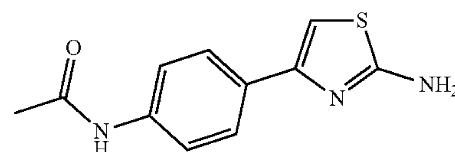
N-(4-(2-aminothiazol-4-yl)phenyl)acetamide
