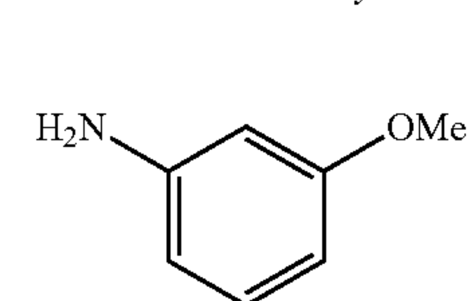
3-methoxyaniline
