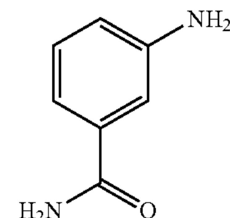
3-aminobenzamide
