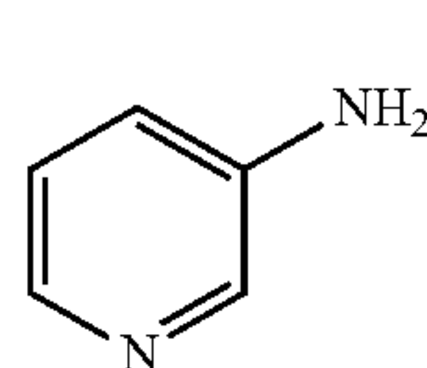
pyridin-3-amine
