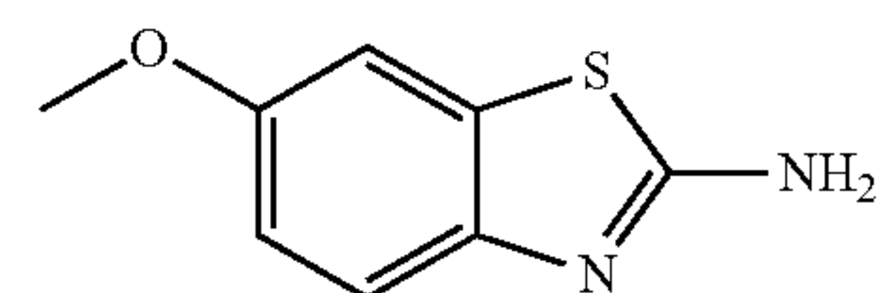
6-methoxybenzo[d]thiazol-2-amine
