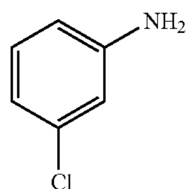
3-chloroaniline
