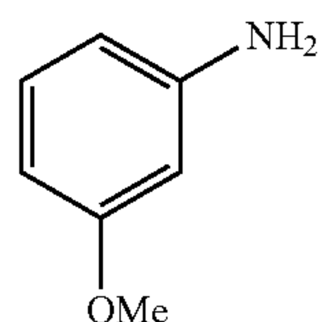
3-methoxyaniline
