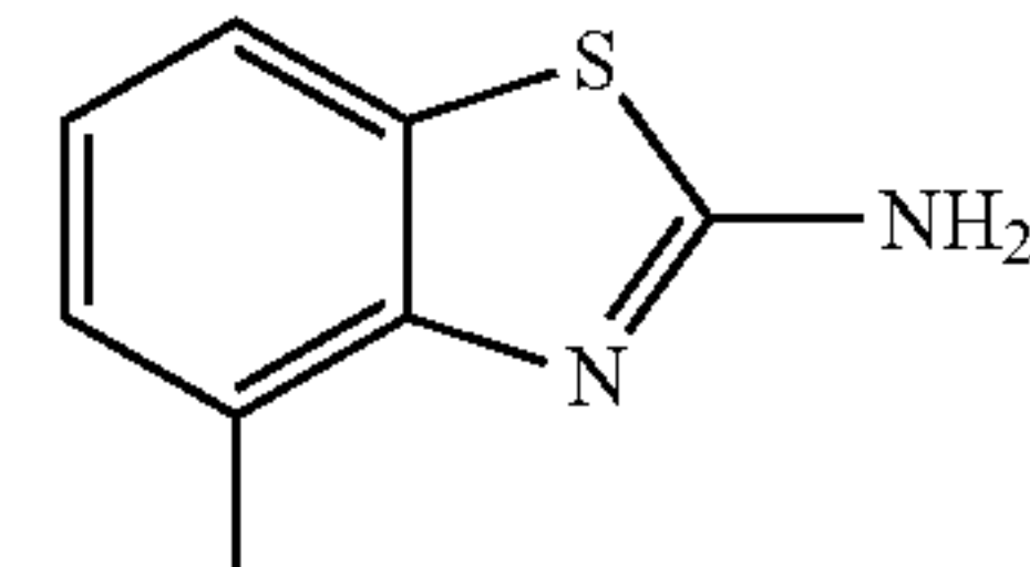
4-methylbenzo[d]thiazol-2-amine
