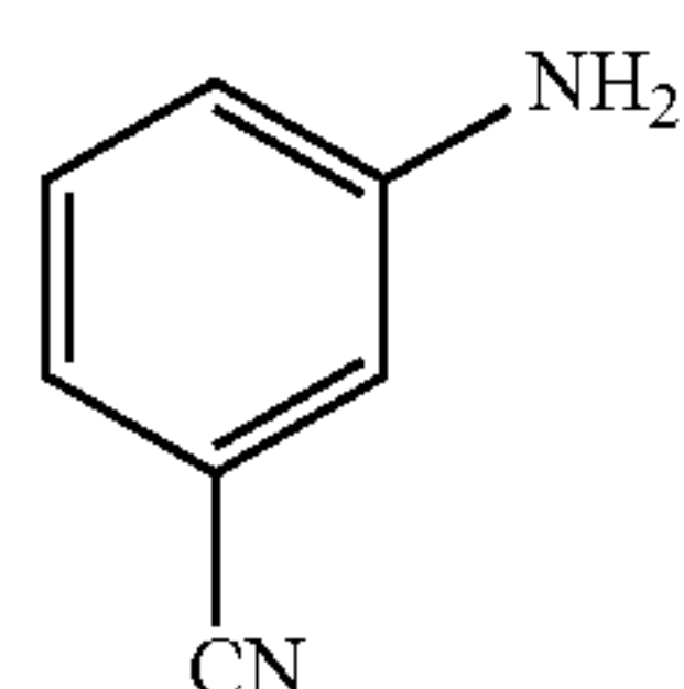
3-aminobenzonitrile
