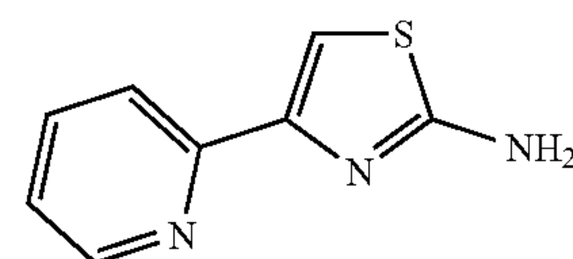
4-(pyridin-2-yl)thiazol-2-amine
