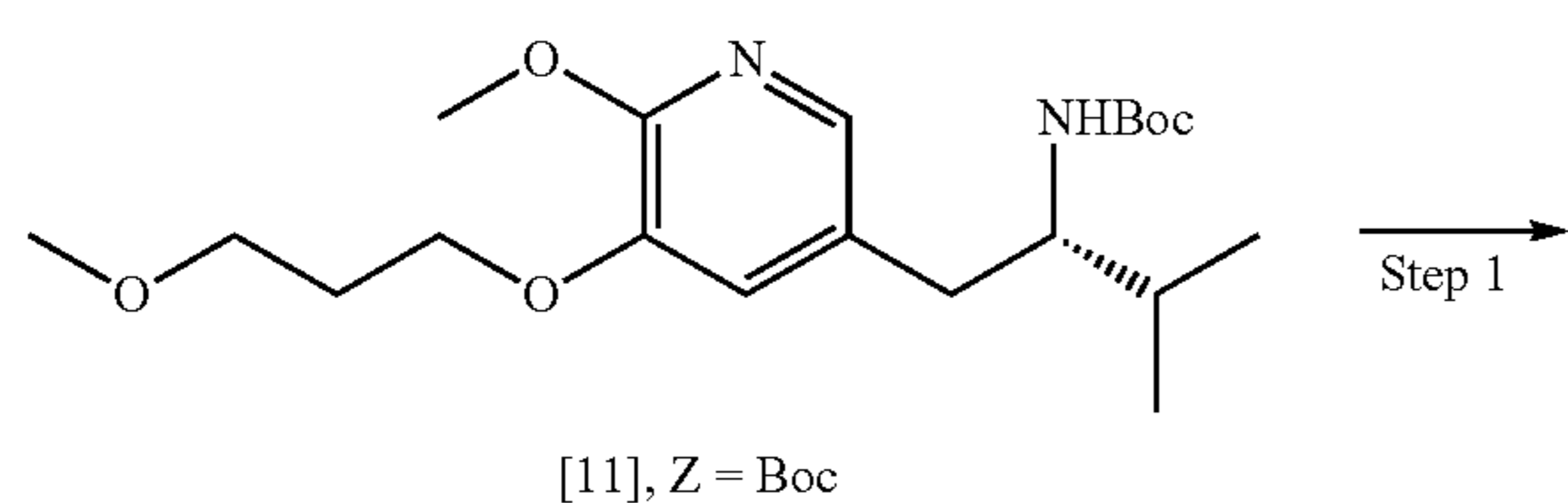
Scheme 19.
