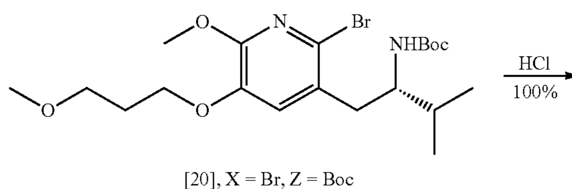
Scheme 20.
