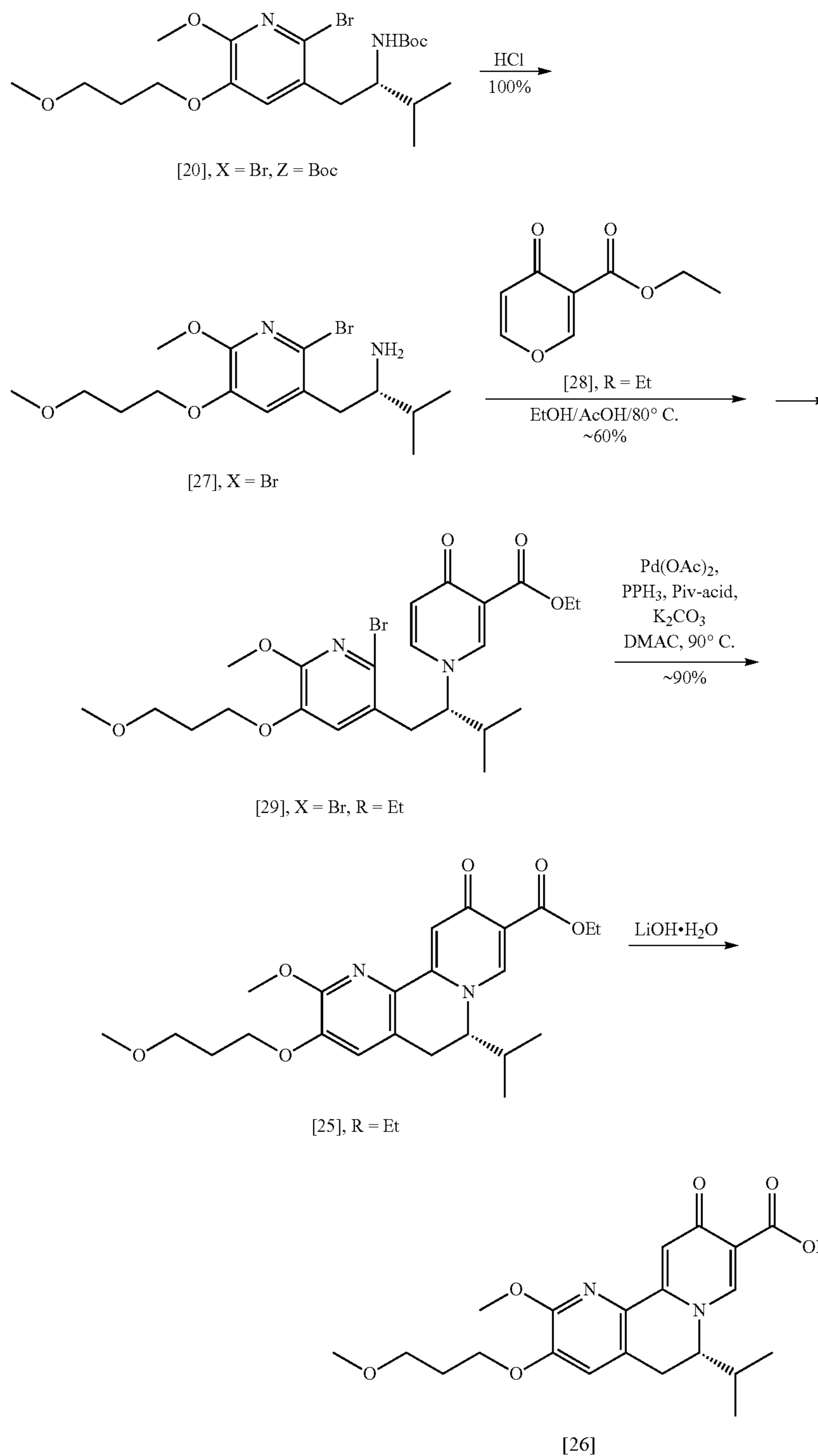
Scheme 21.
