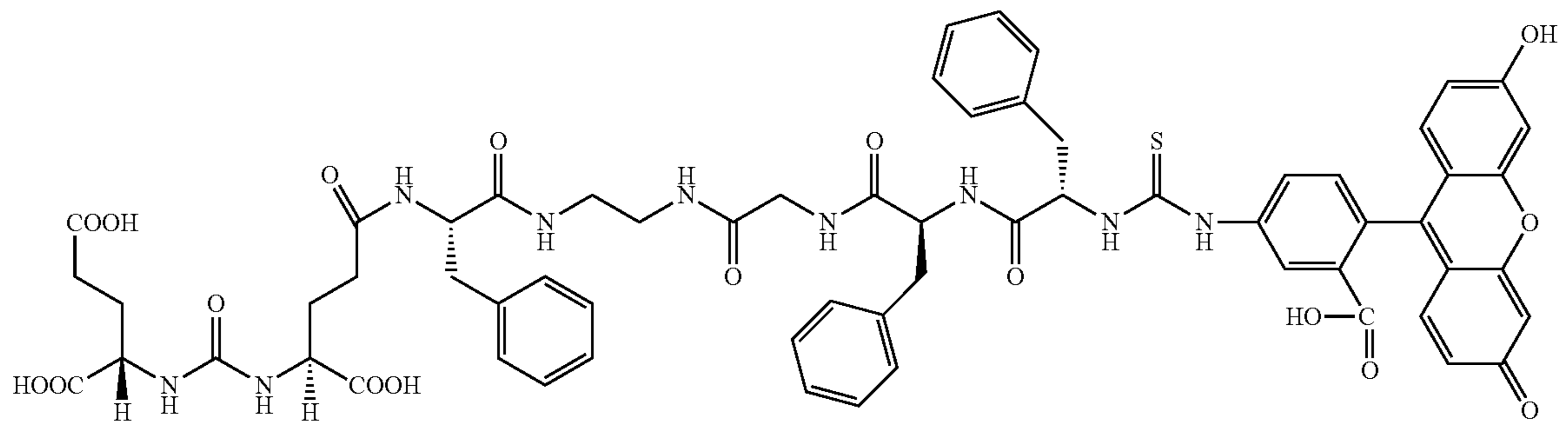
FITC conjugate
