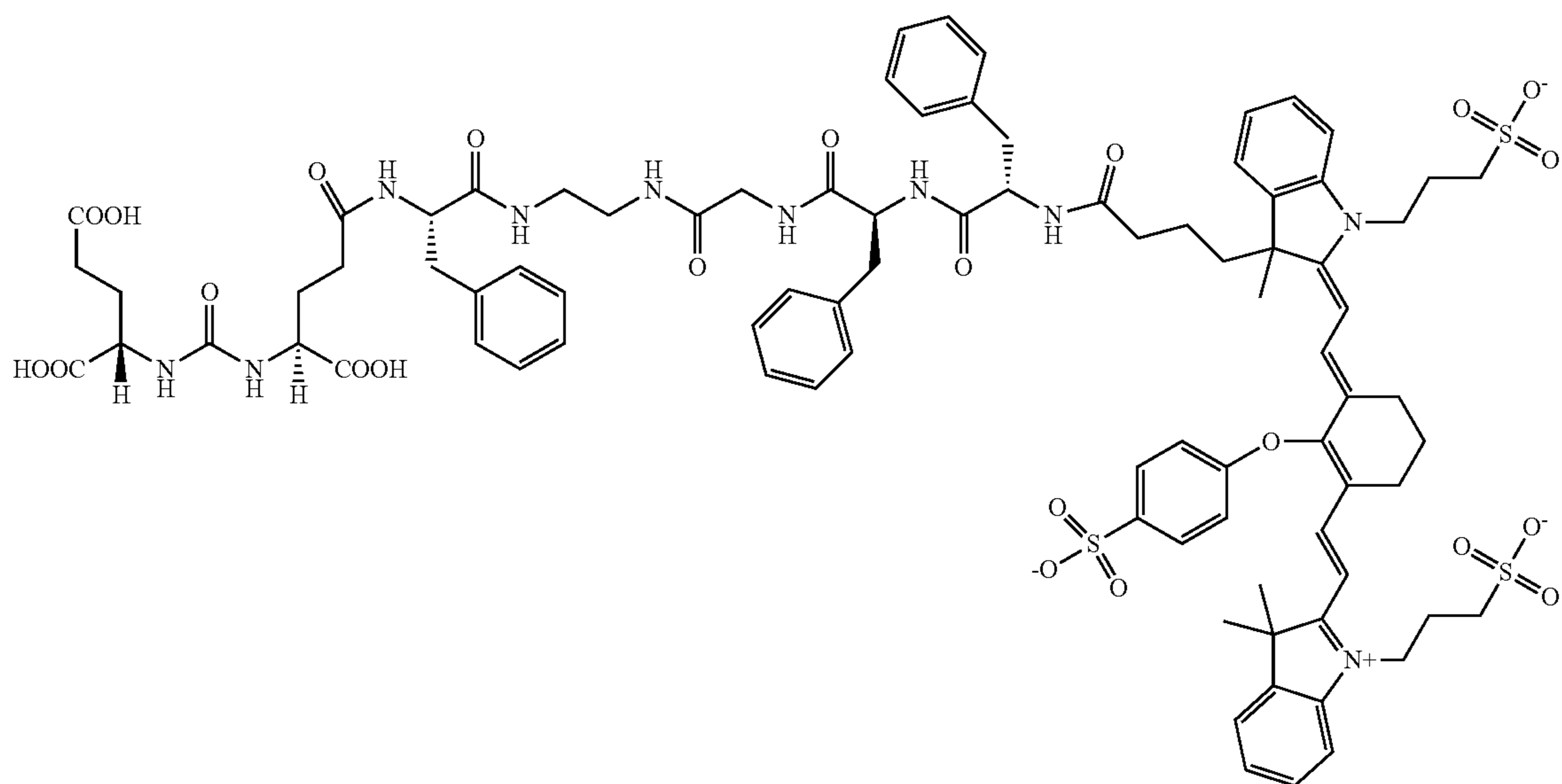
DyLight 800 Conjugate
