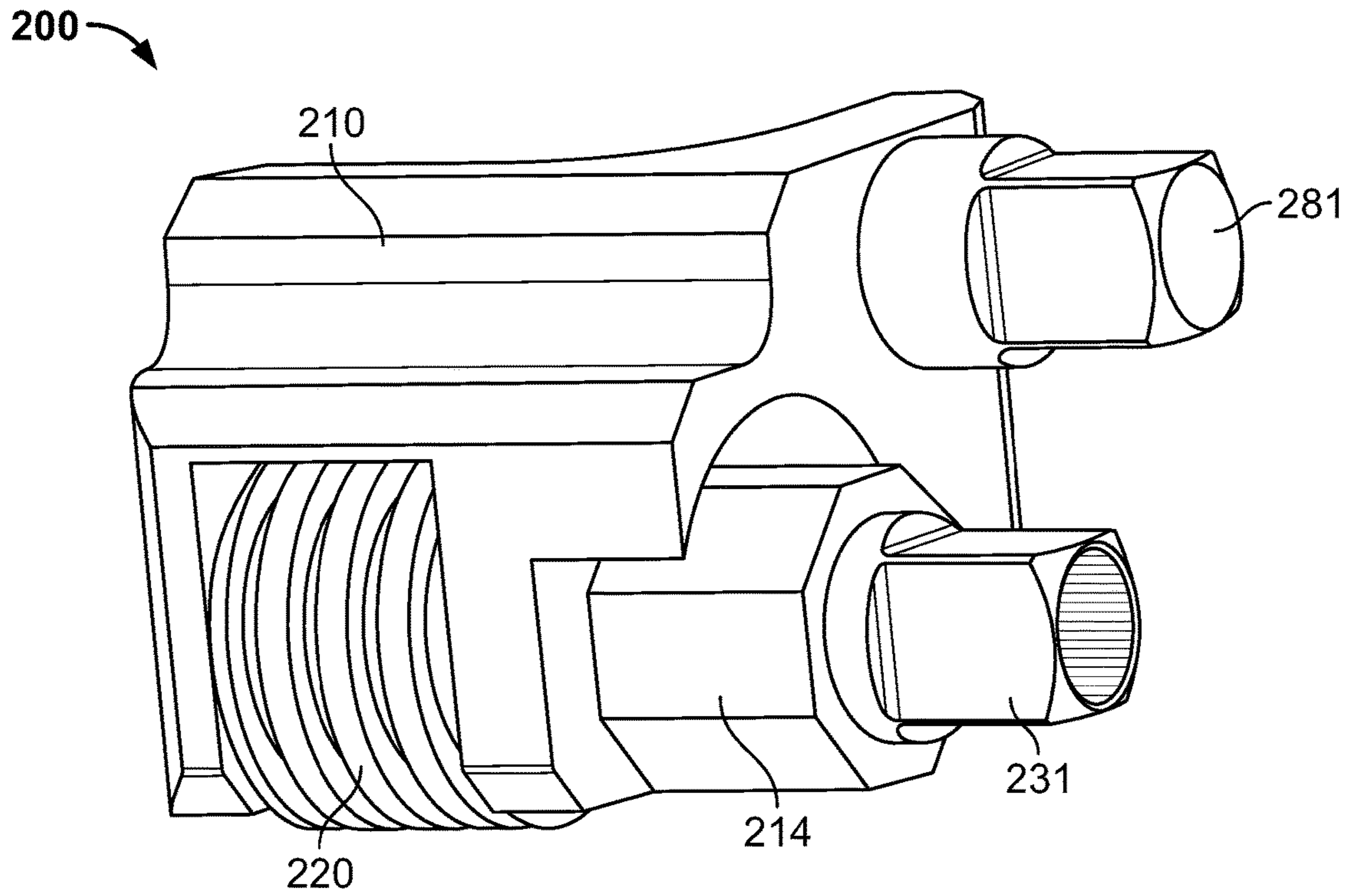
FIG. 4A
