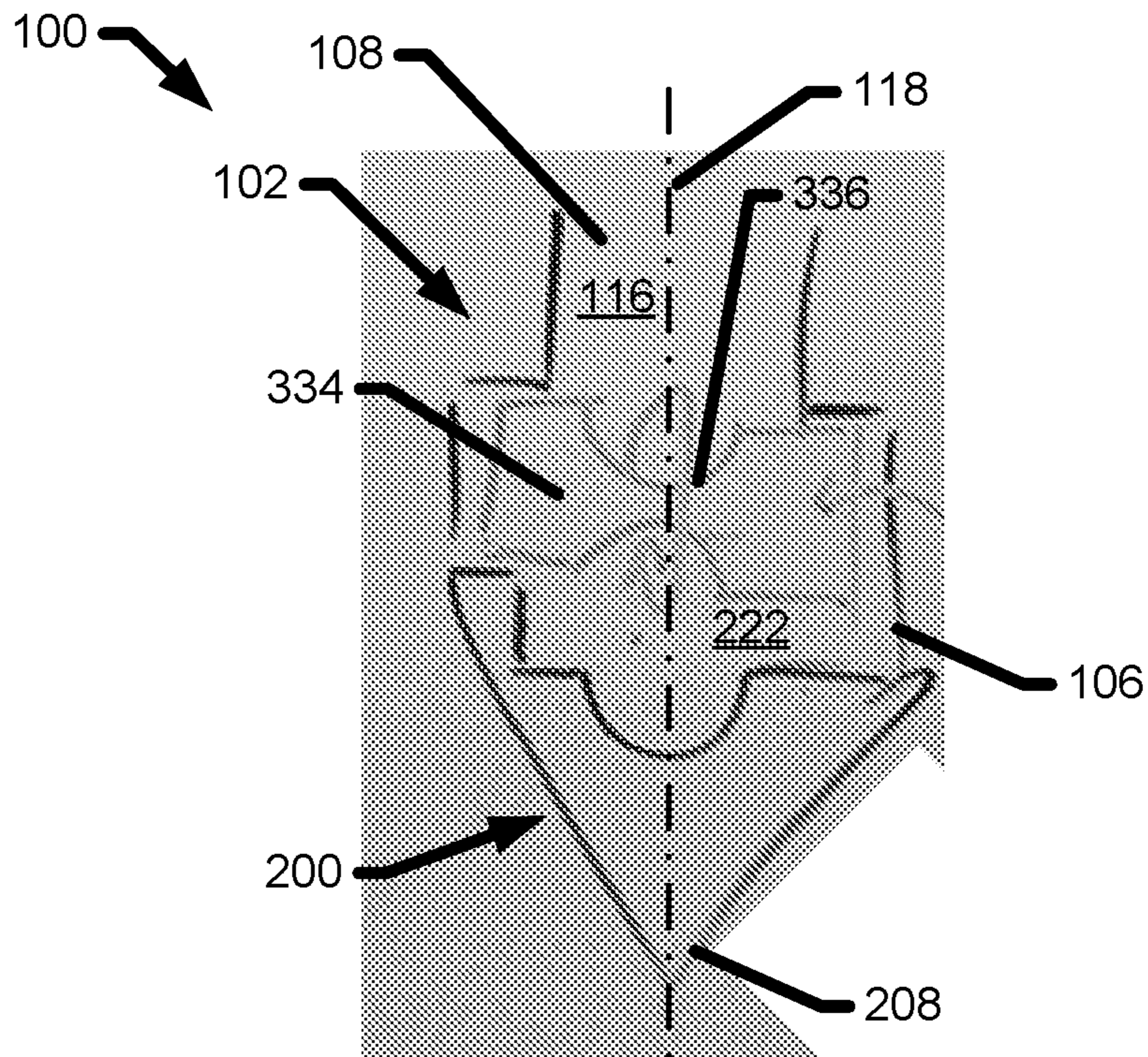
FIG. 28
