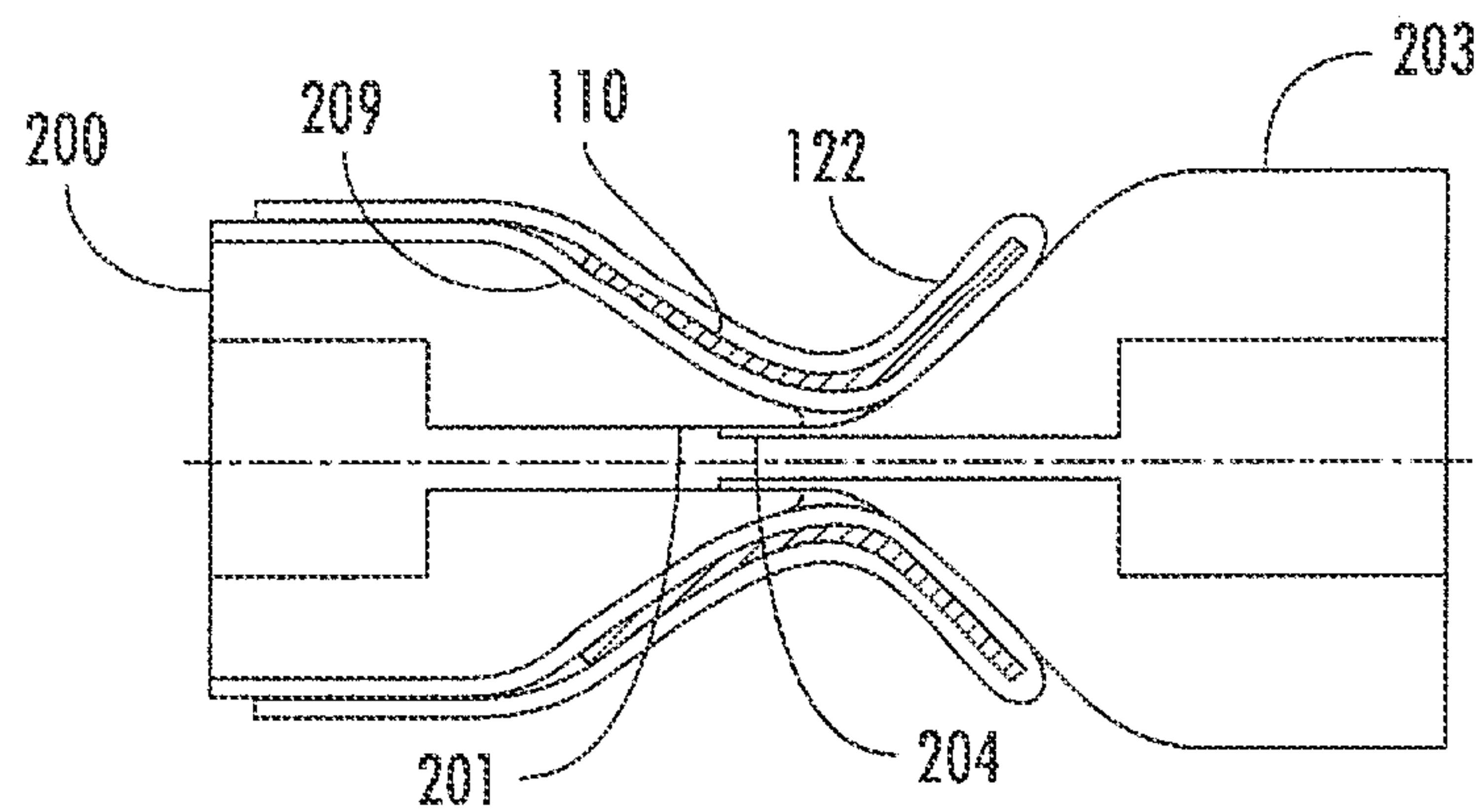
FIG. 15F
