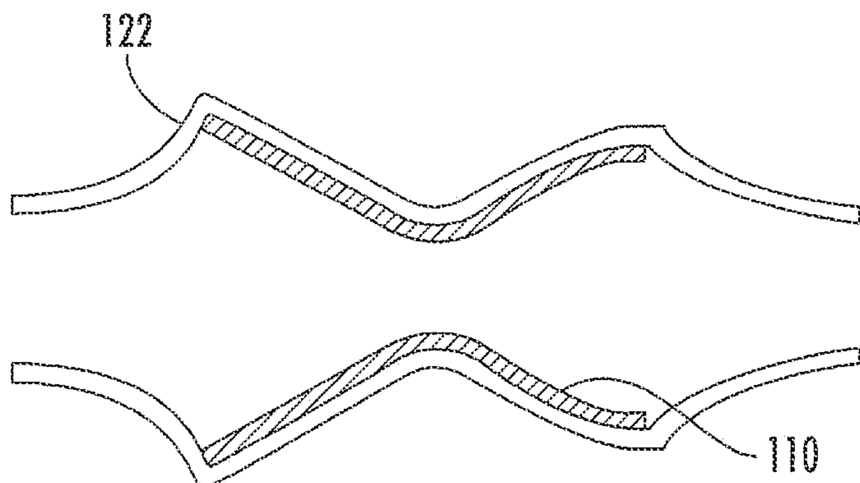
FIG. 12A
