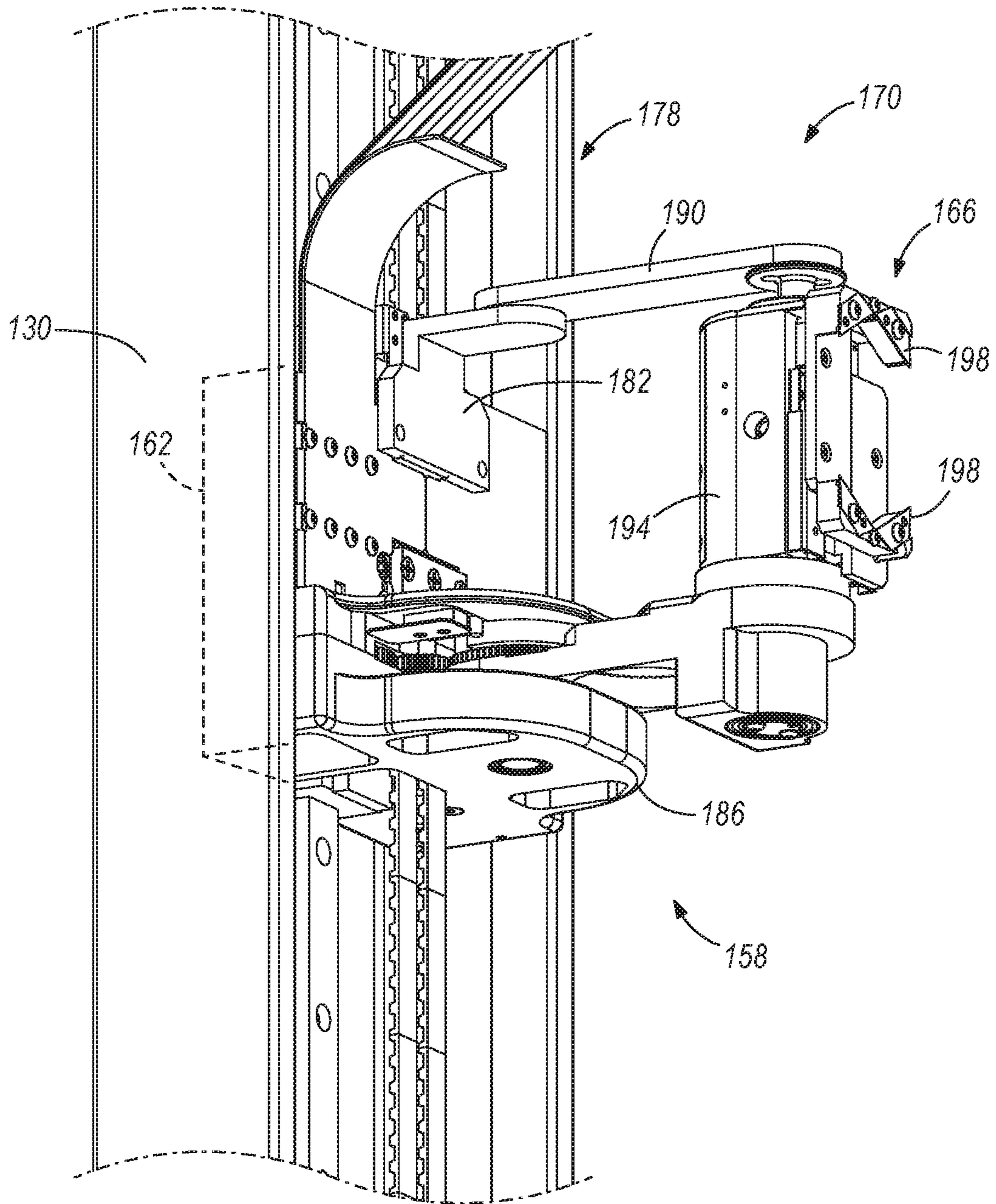
FIG. 12
