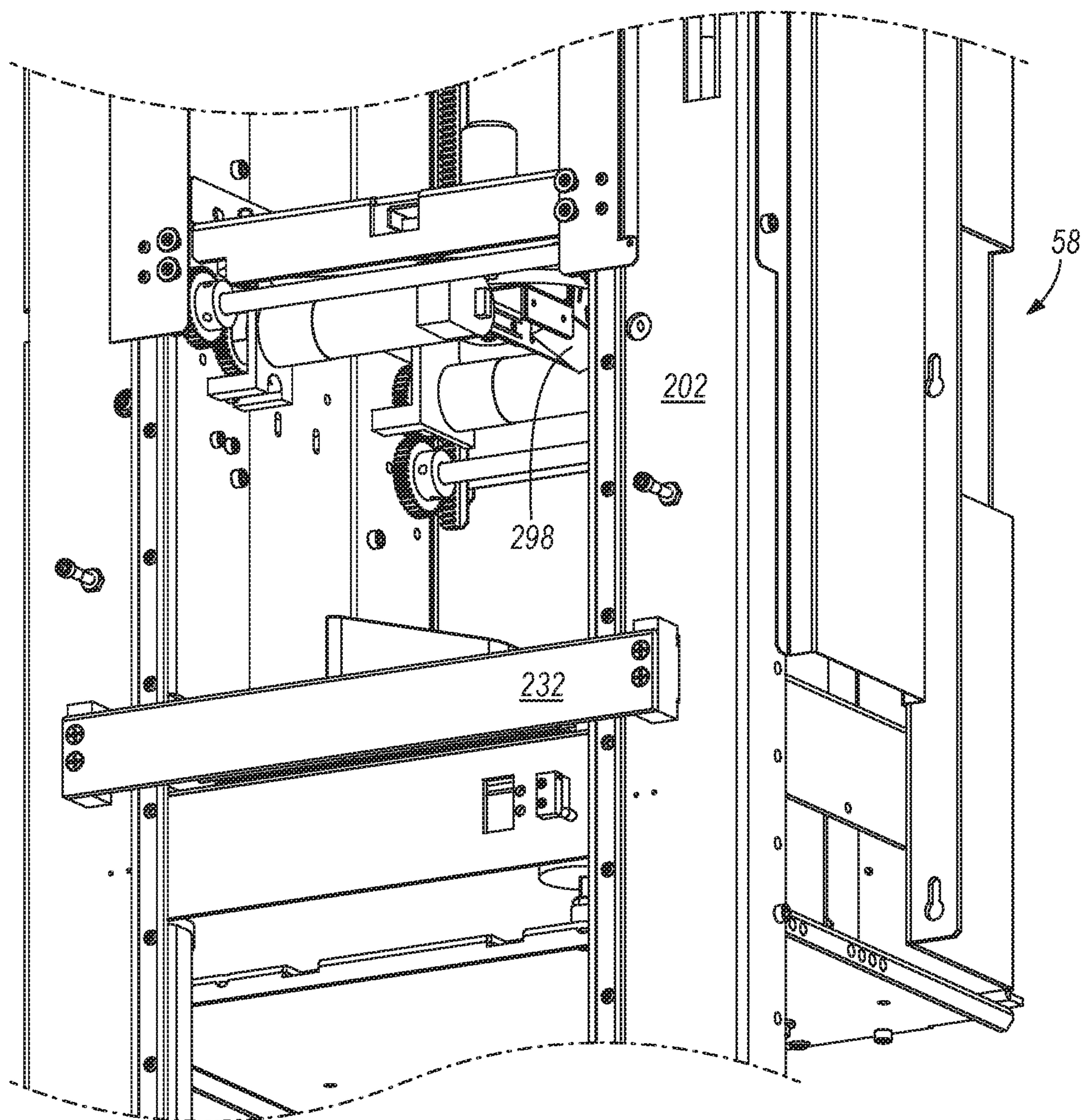
FIG. 26
