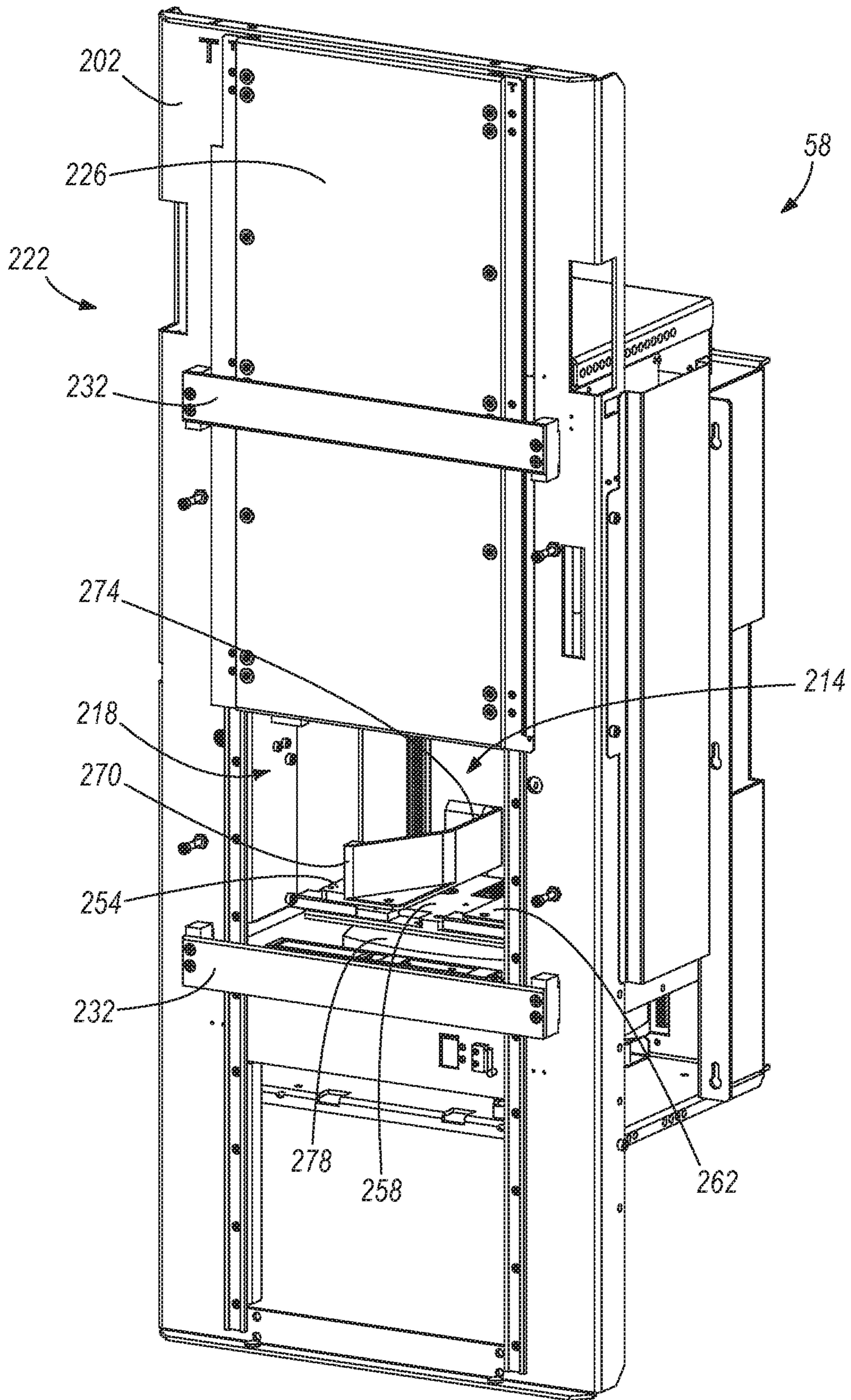
FIG. 22
