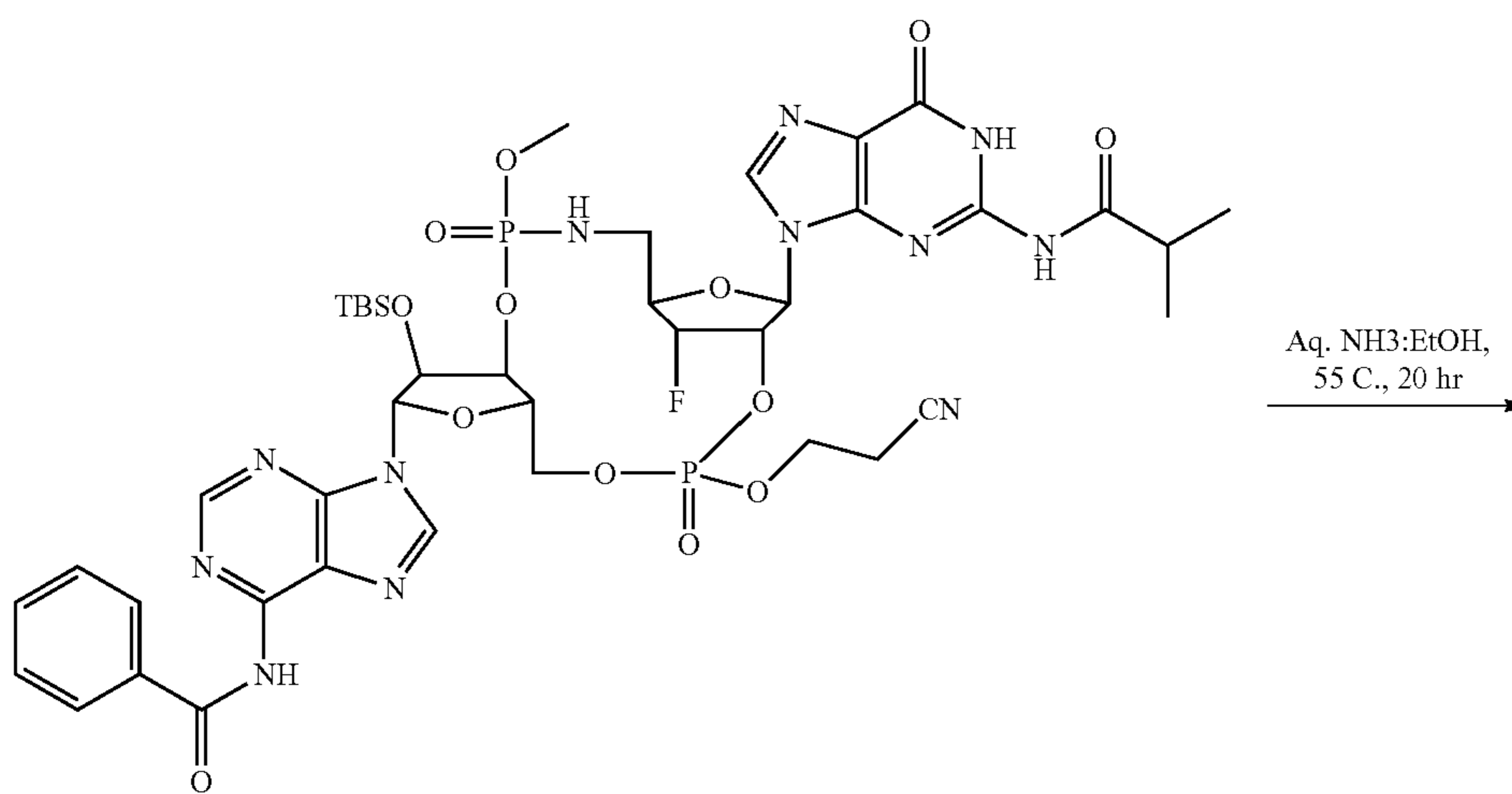
18f
