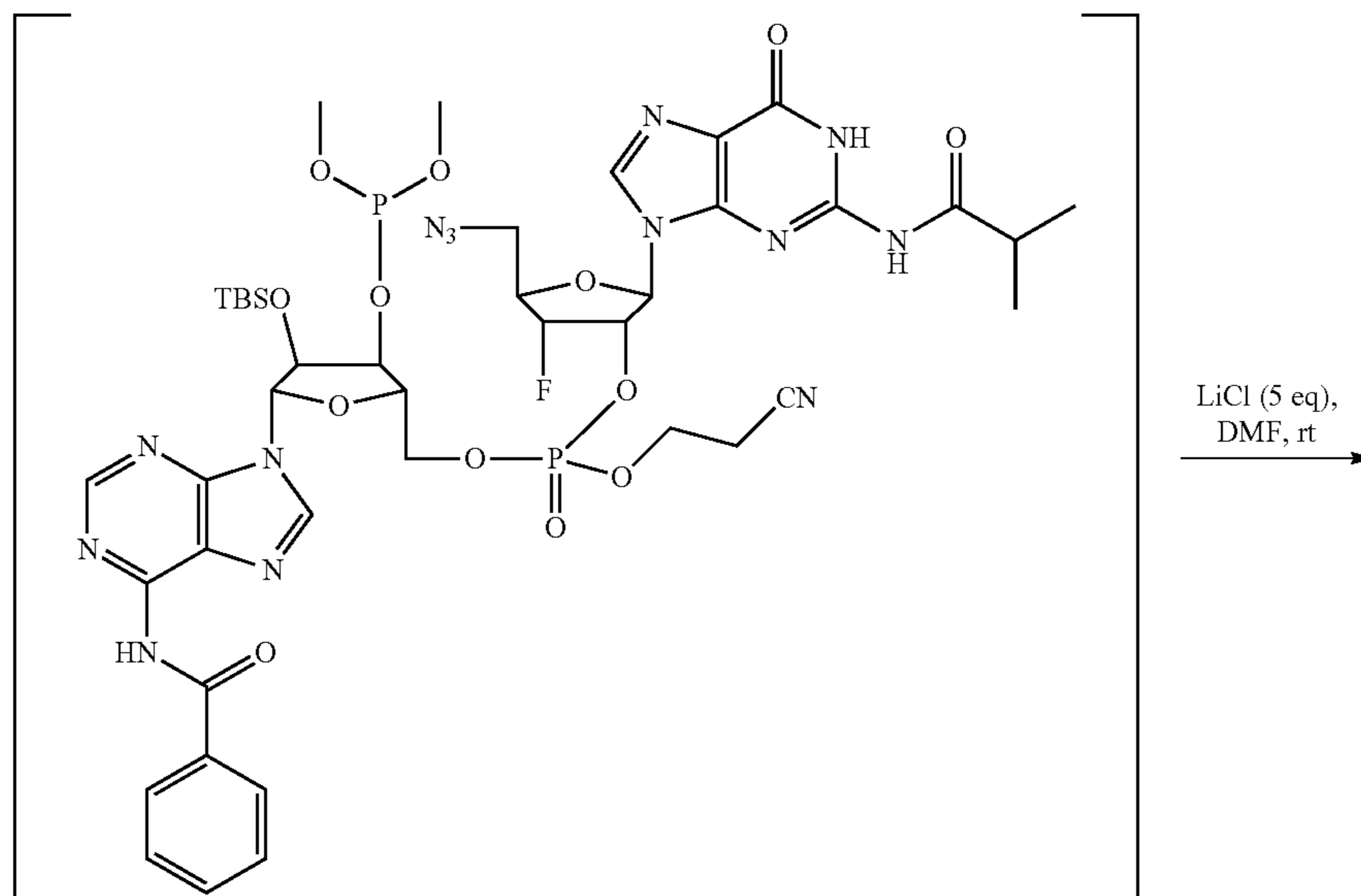
18e
