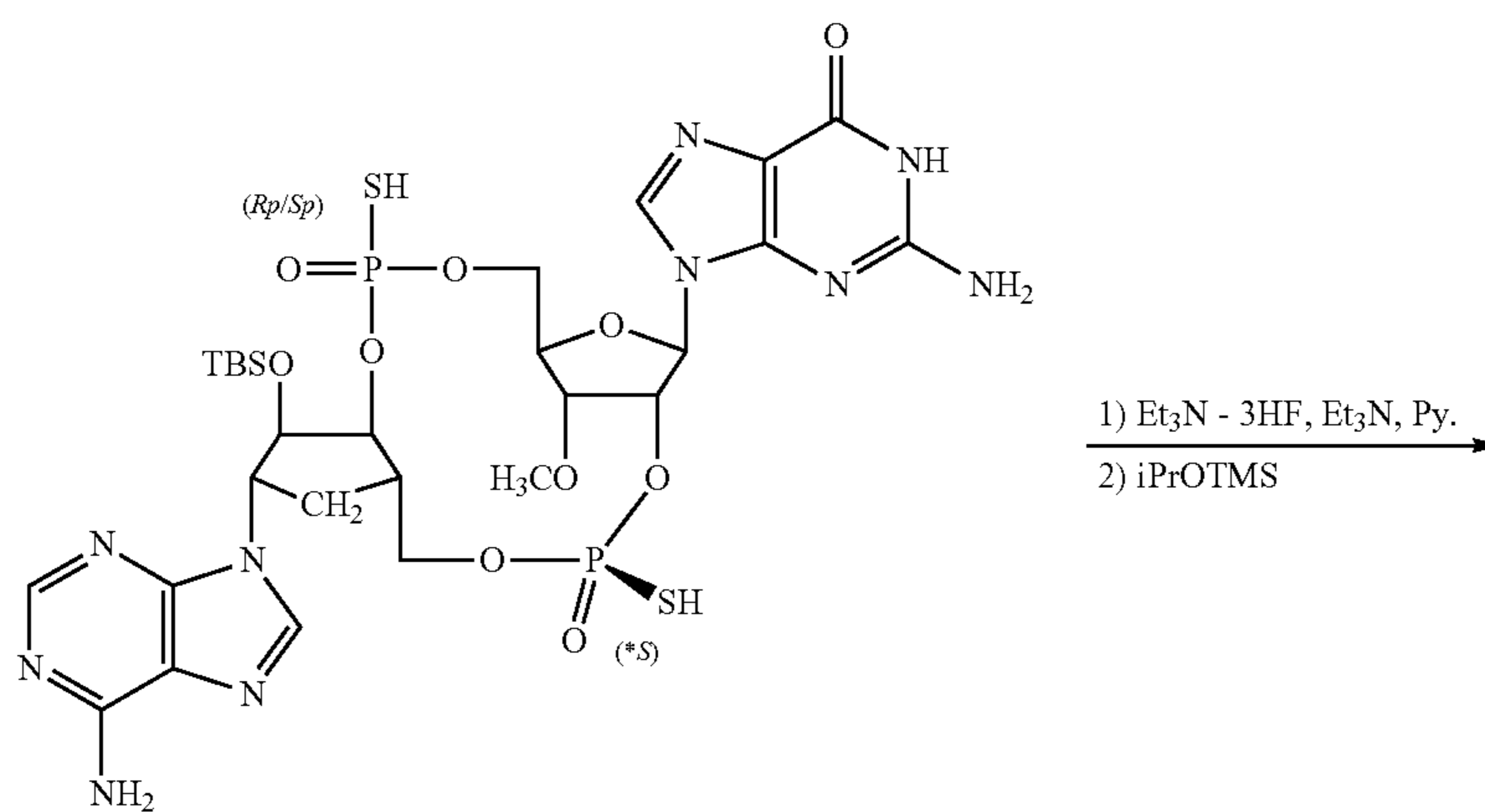
5p
