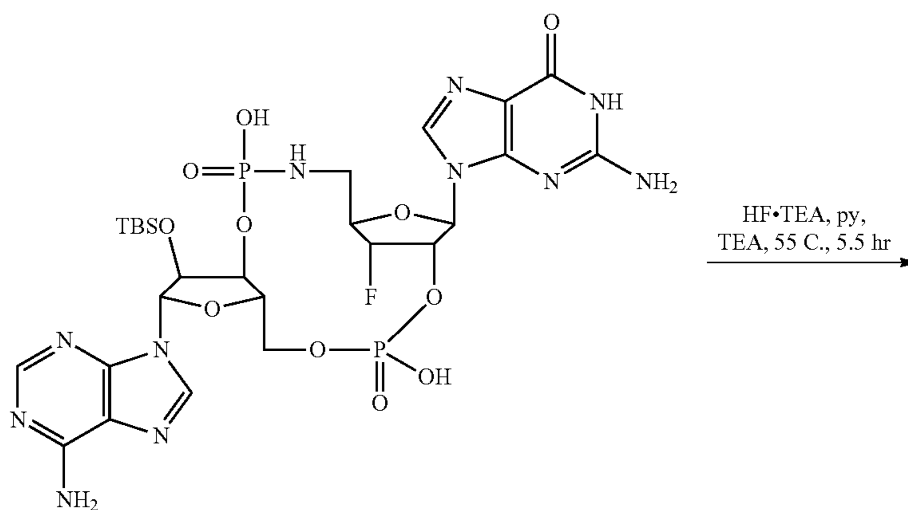
18g
