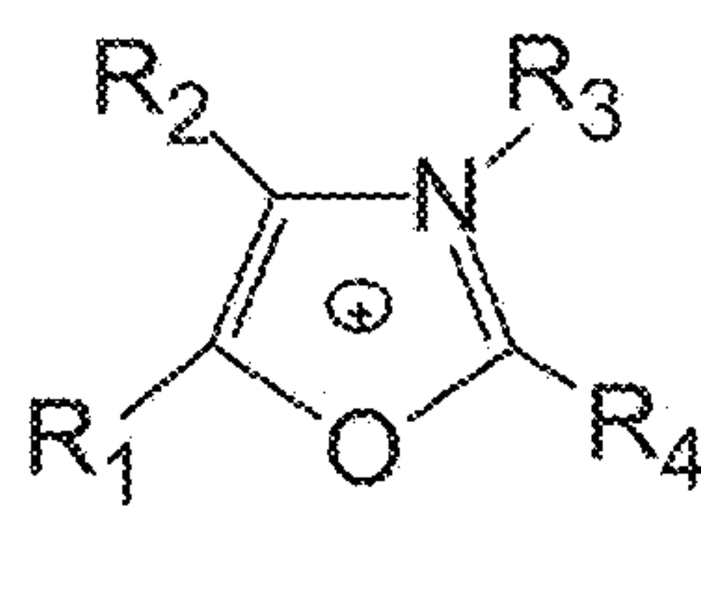
Oxazolium
