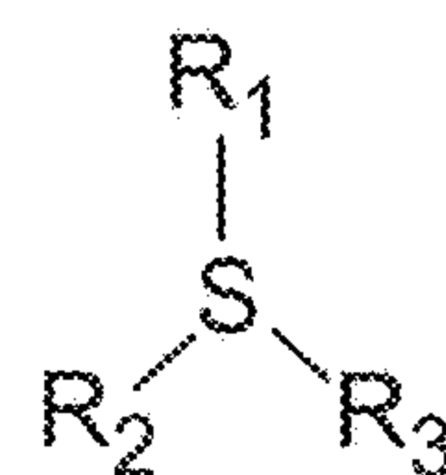
Sulfonium
