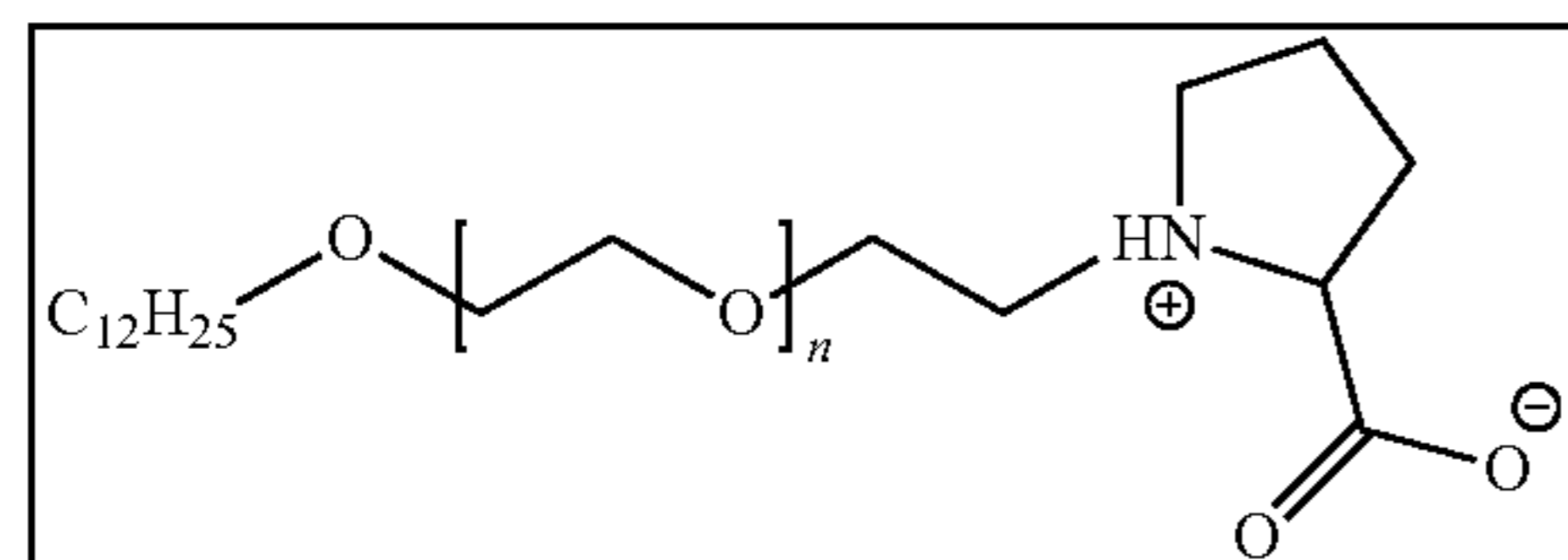
BrijL-23-Proline
