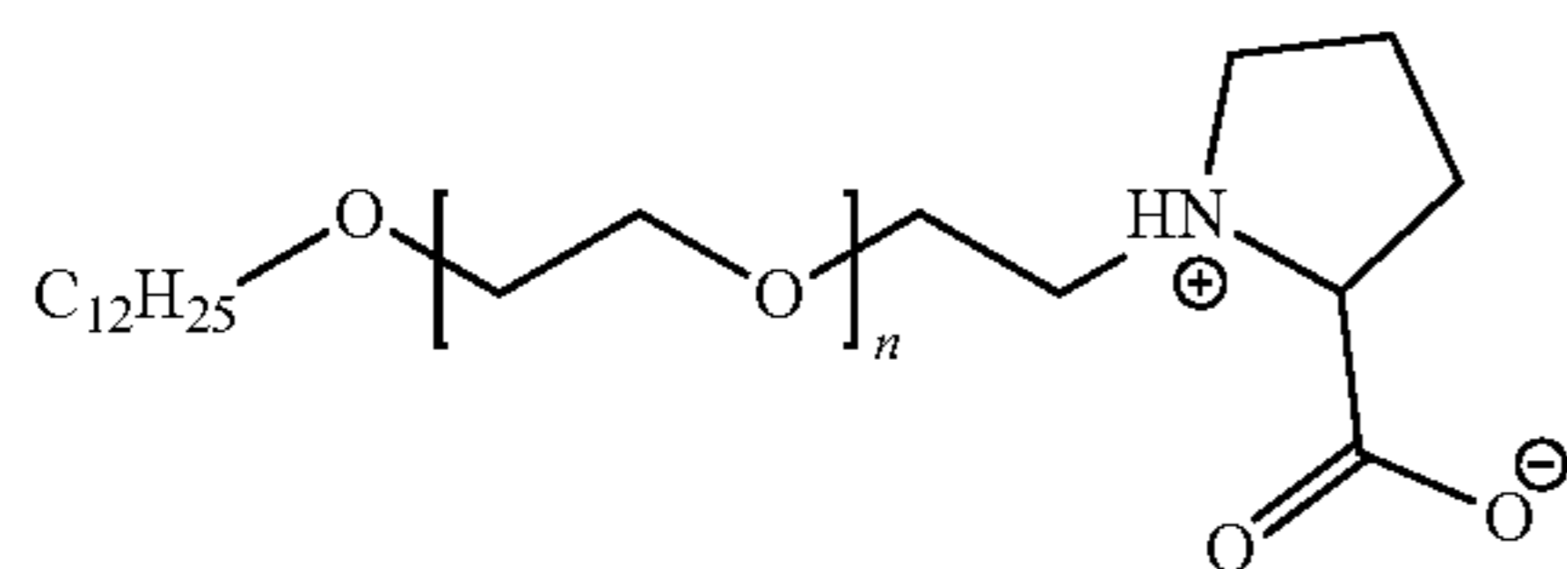
BrijL-23-Proline
