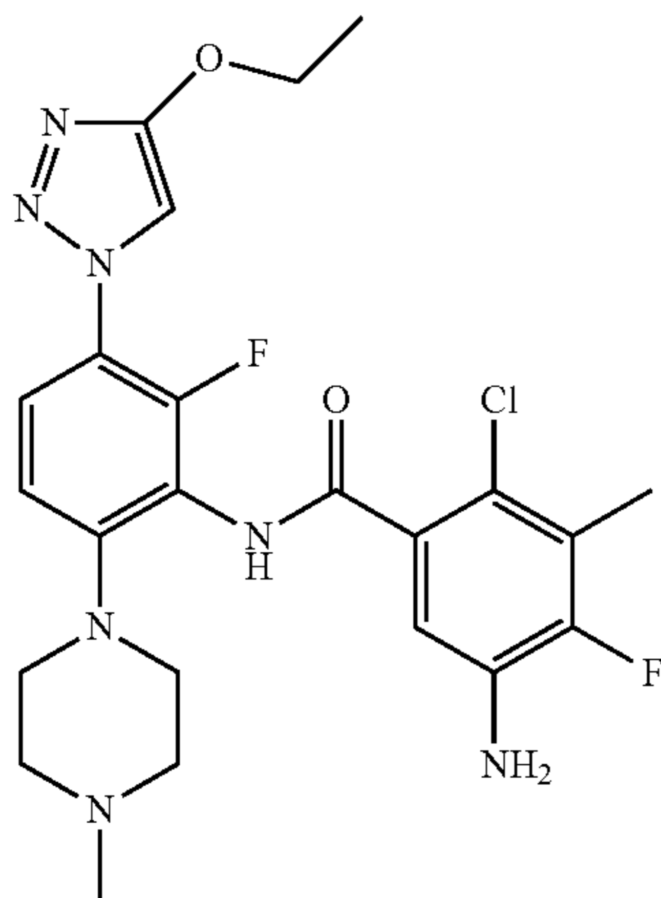
5-amino-2-fluoro-N-(3-(4-Ethoxy-1H-1,2,3-triazol-1-yl)-2-fluoro-6-(4-methylpiperazin-1-yl)phenyl)-4-fluoro-3-Methyl benzamide (20)
