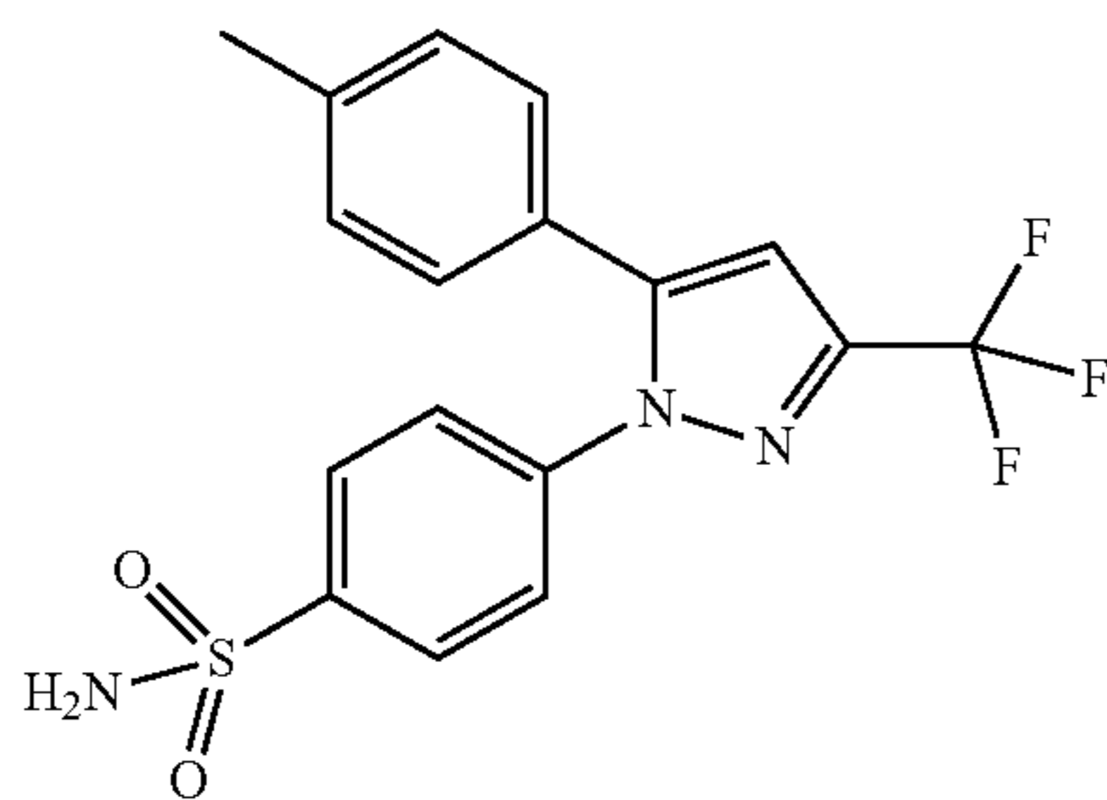
Celecoxib
