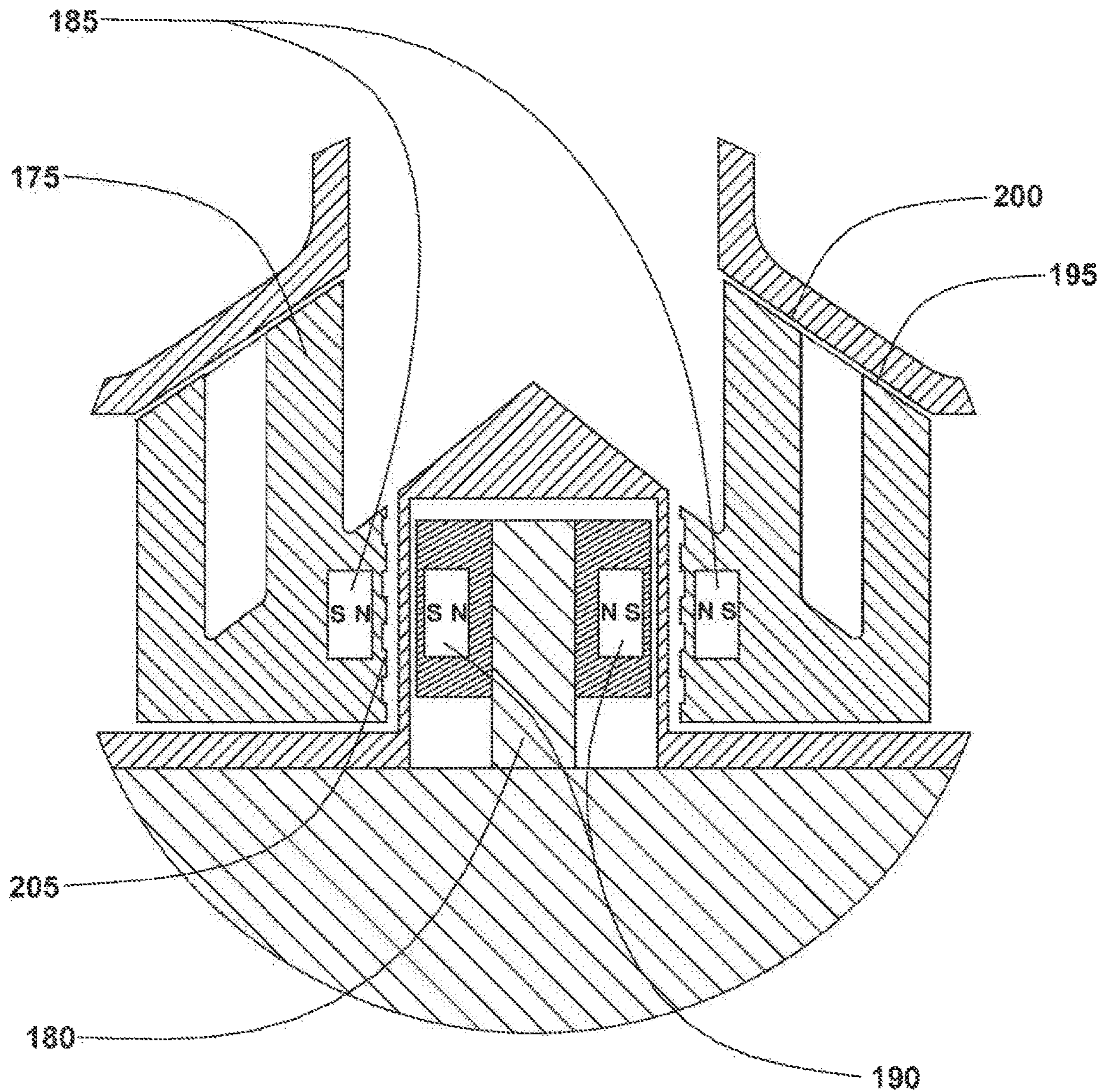
FIG. 17 (DETAIL E)
