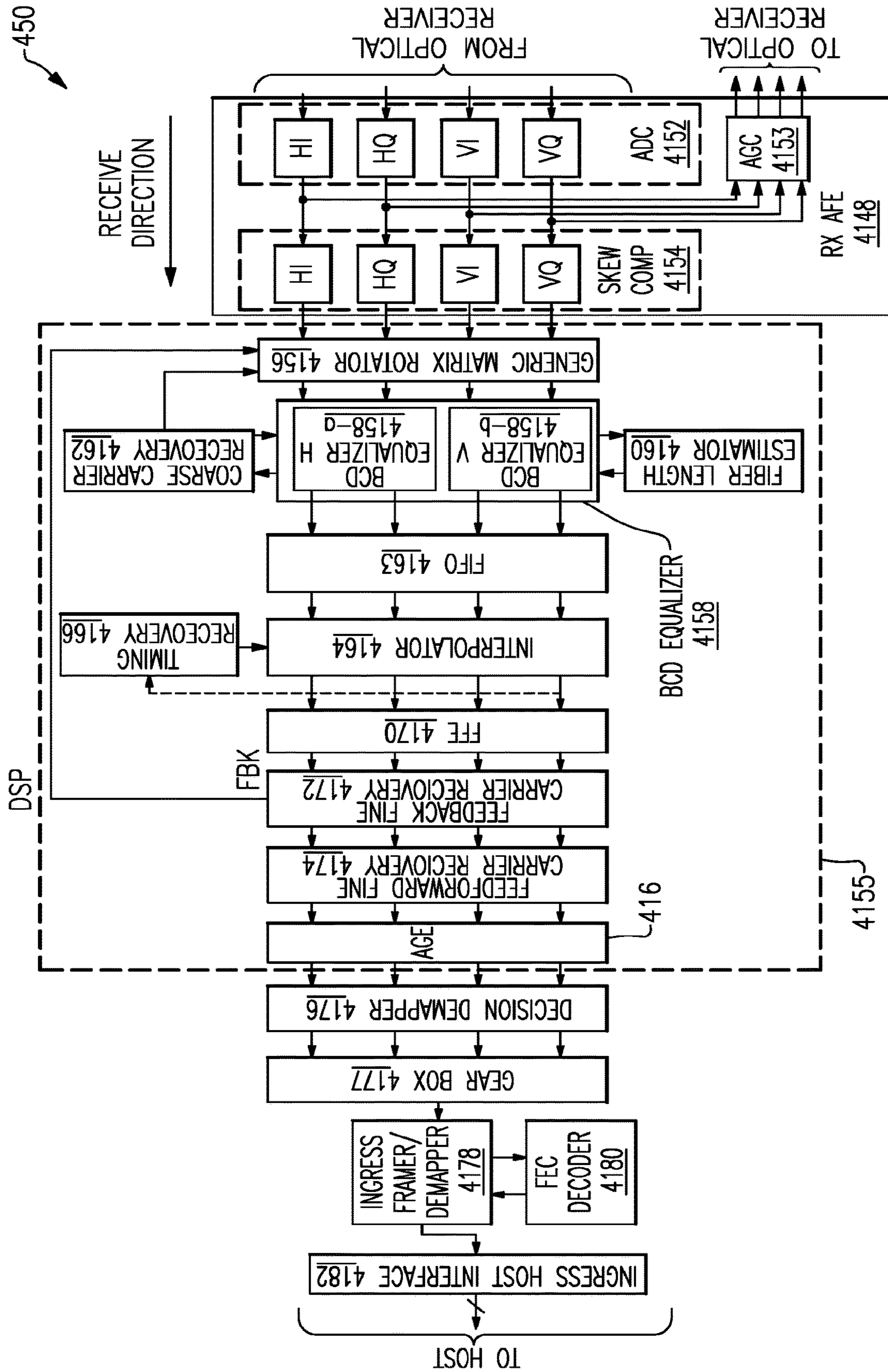
FIG.4C
