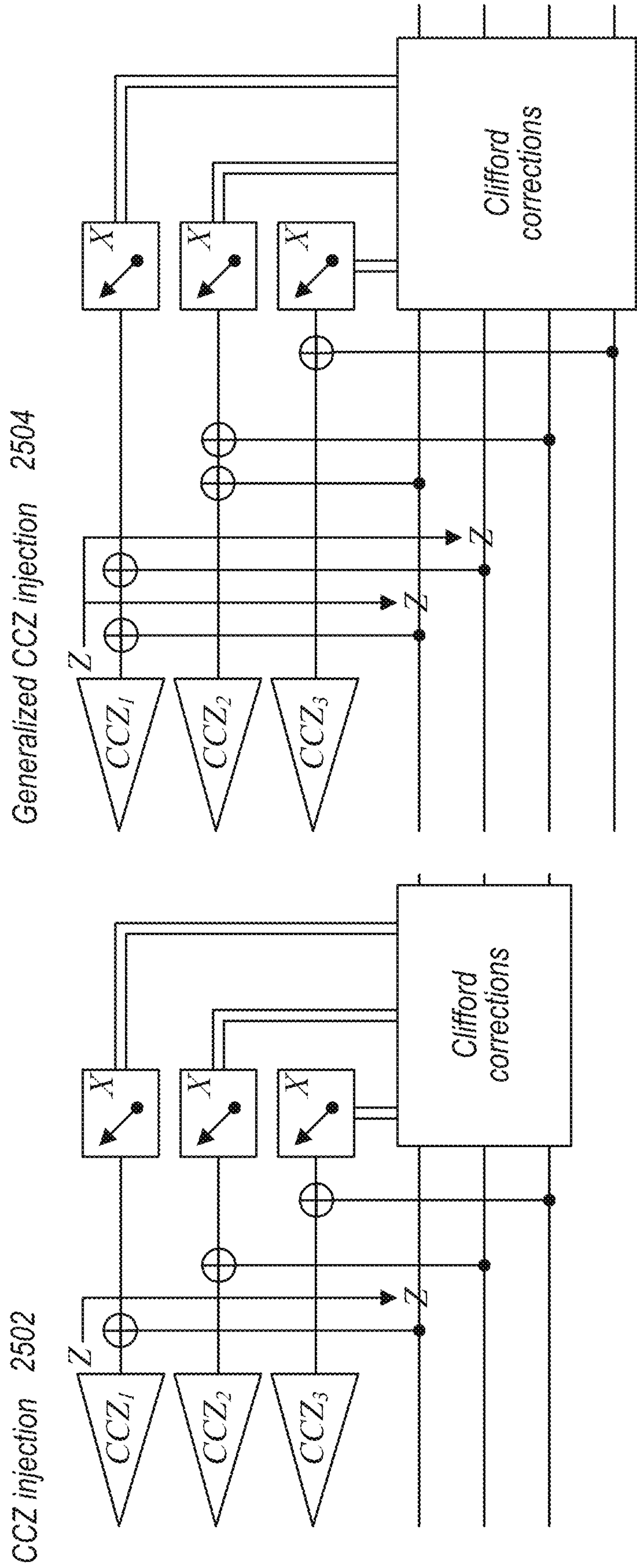
FIG. 25
