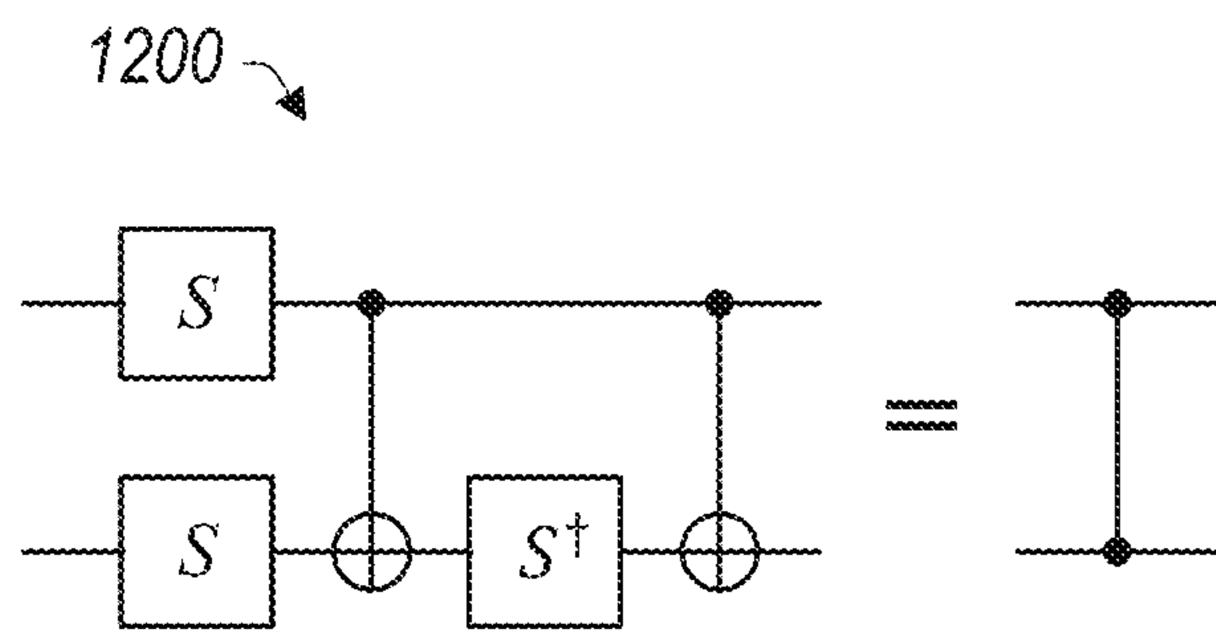
FIG. 12
