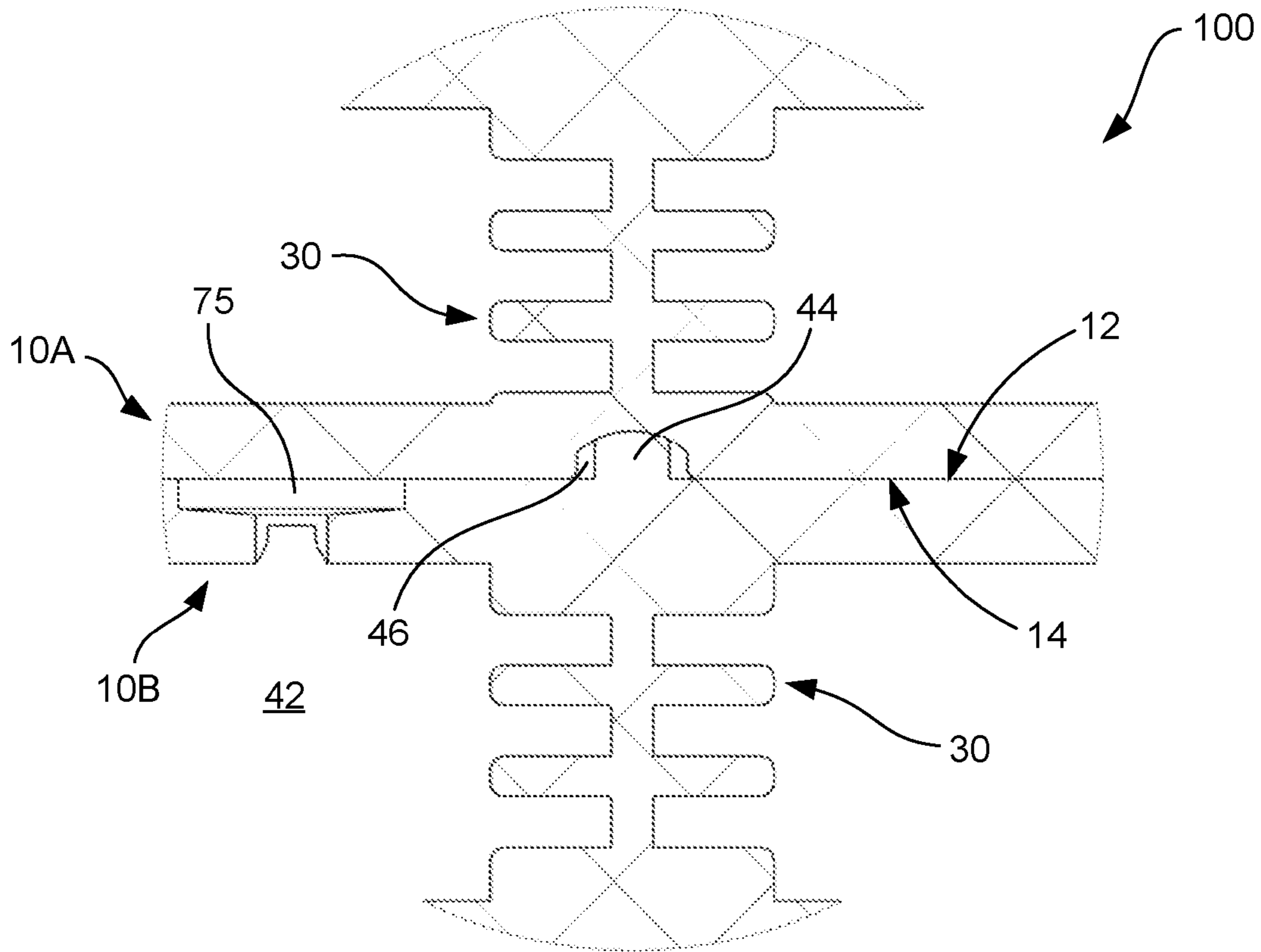
FIG. 29
