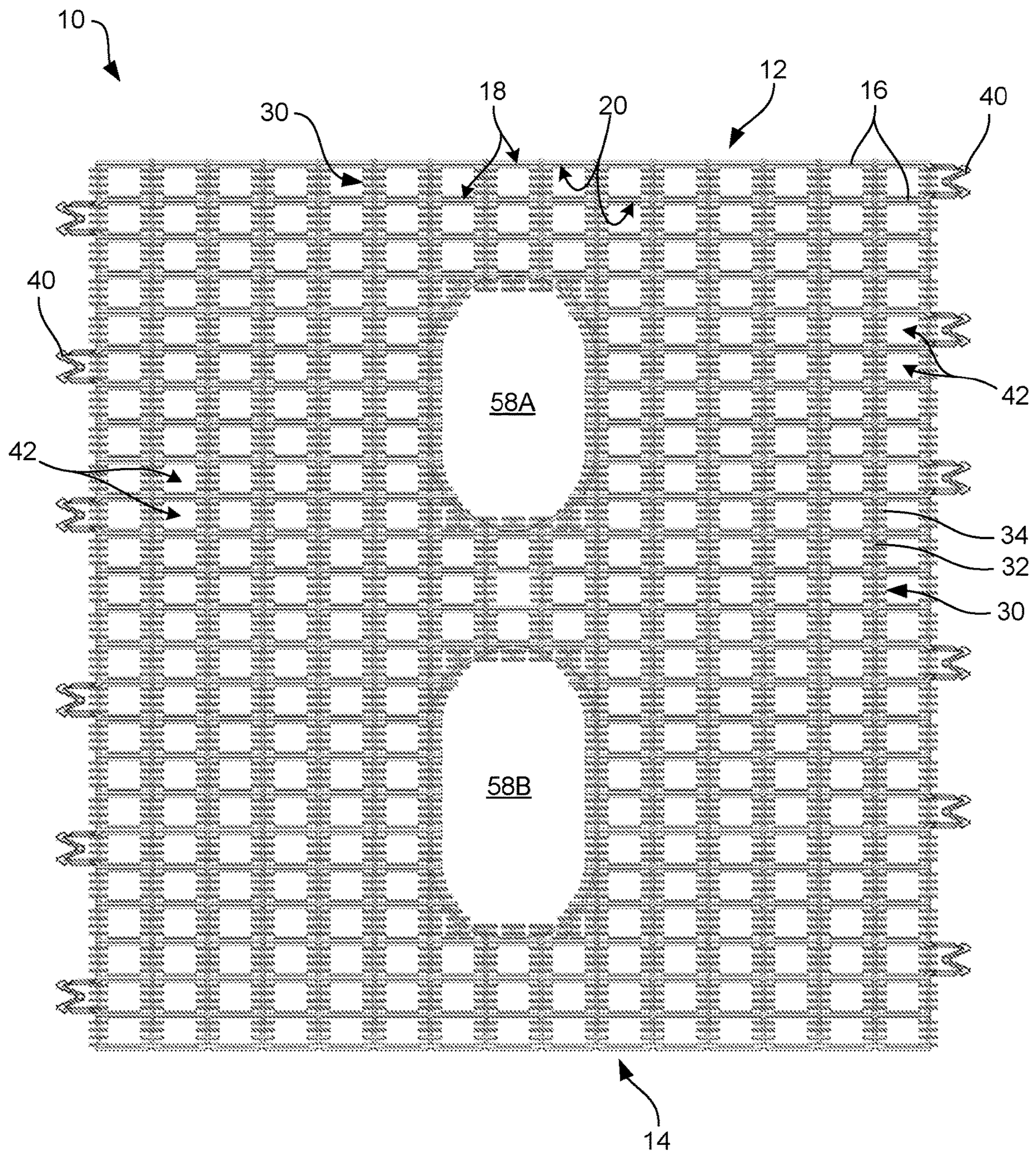
FIG. 21A
