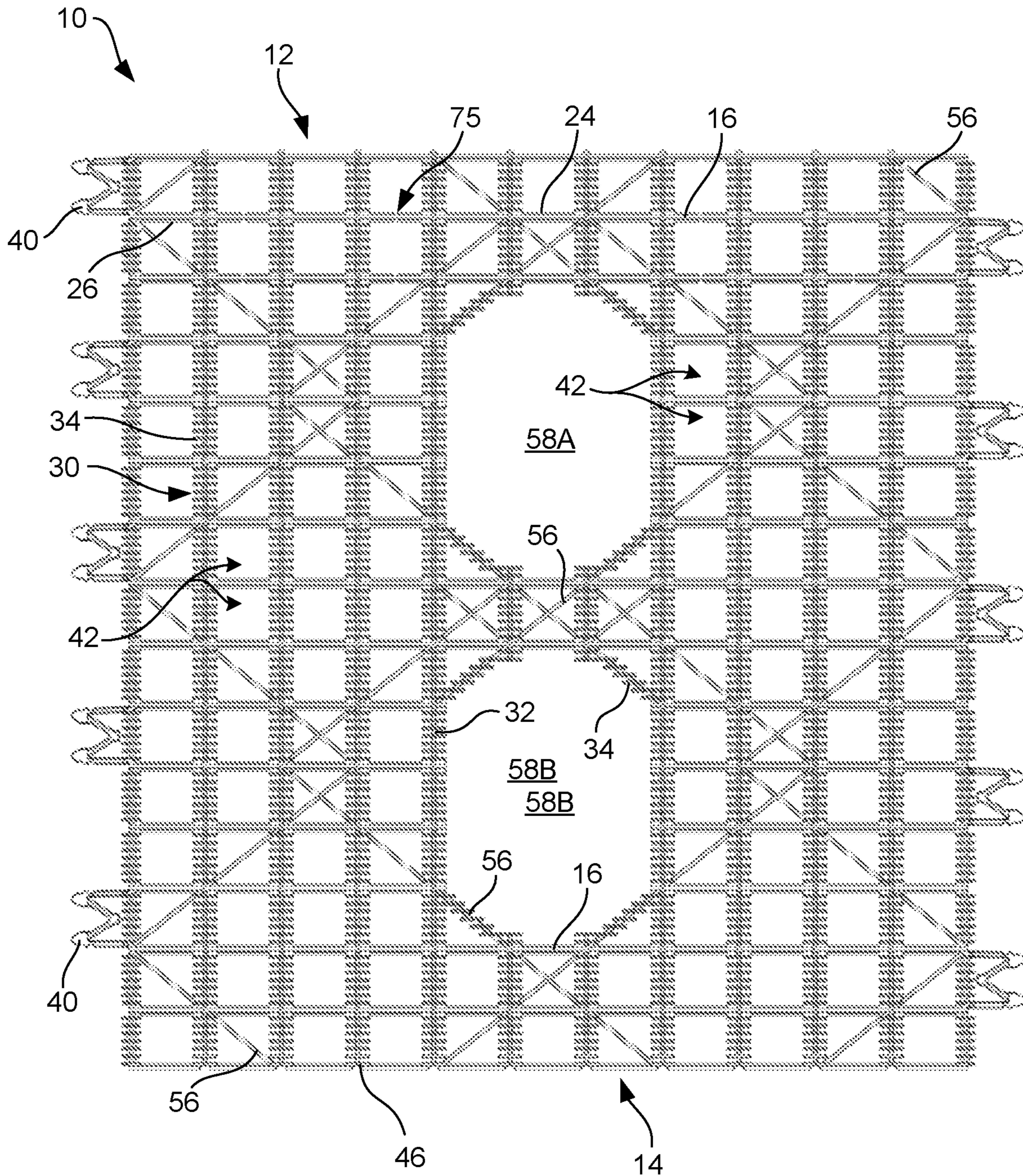
FIG. 24C
