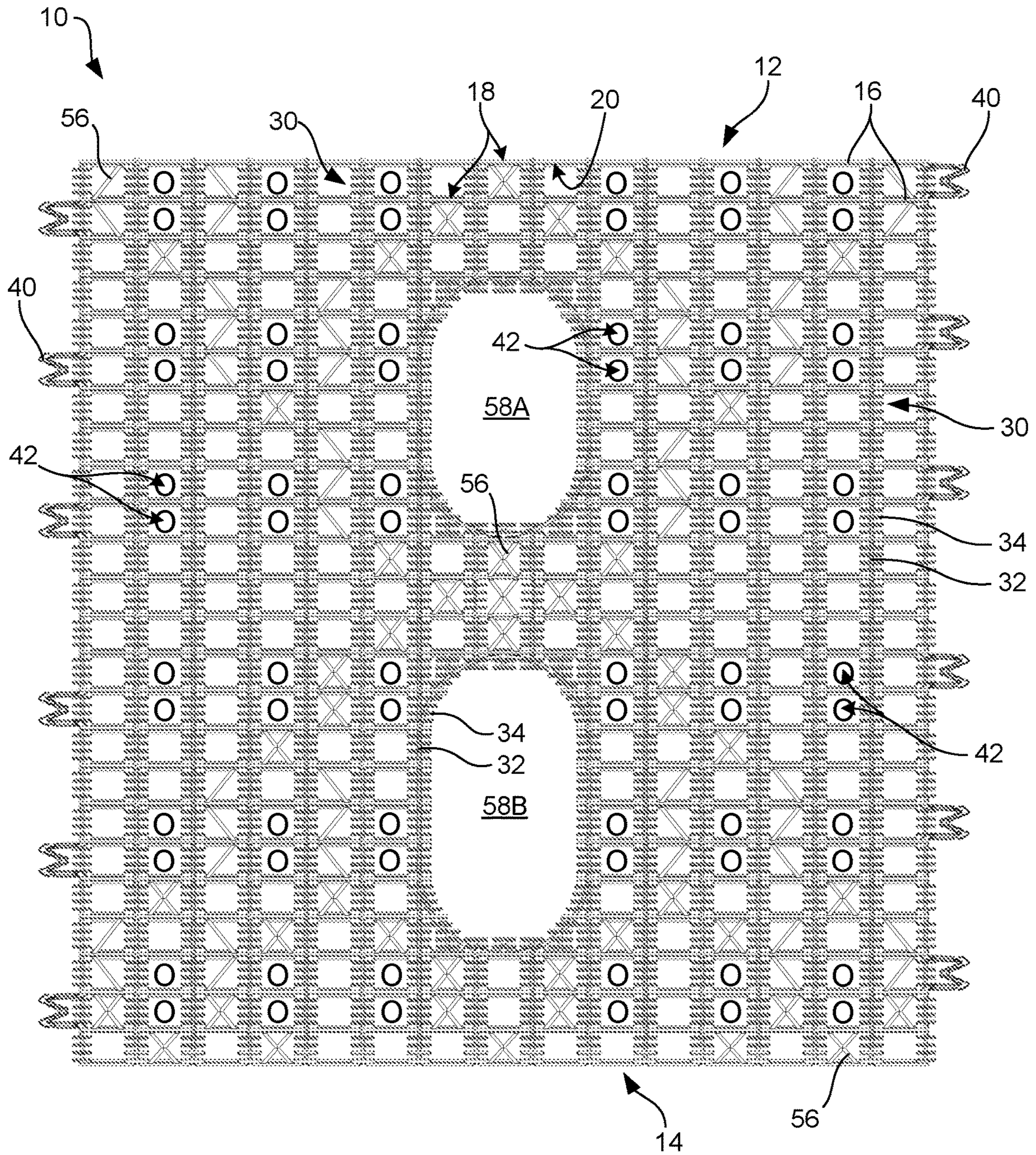
FIG. 23
