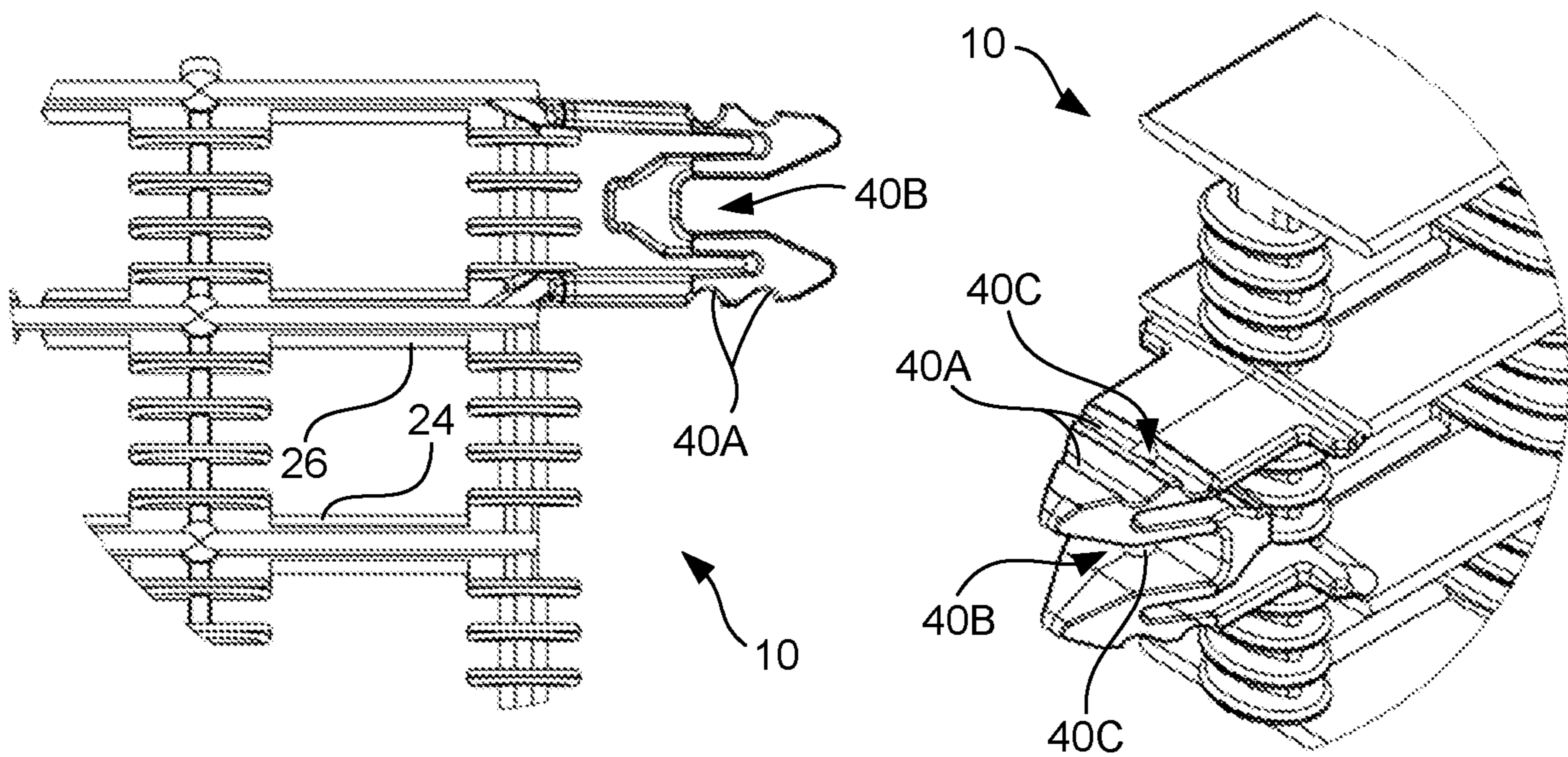
FIG. 30A
