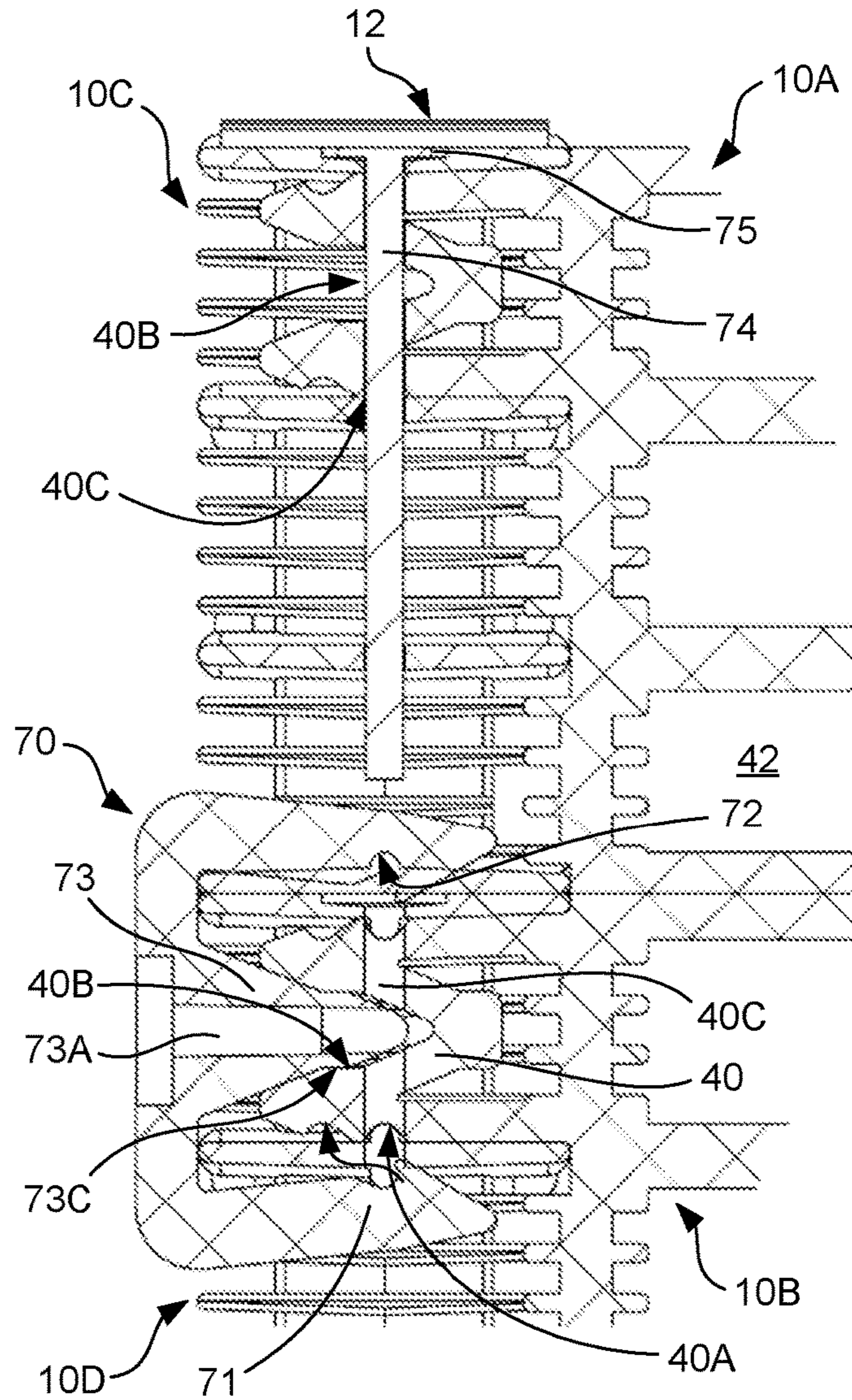
FIG. 32D
