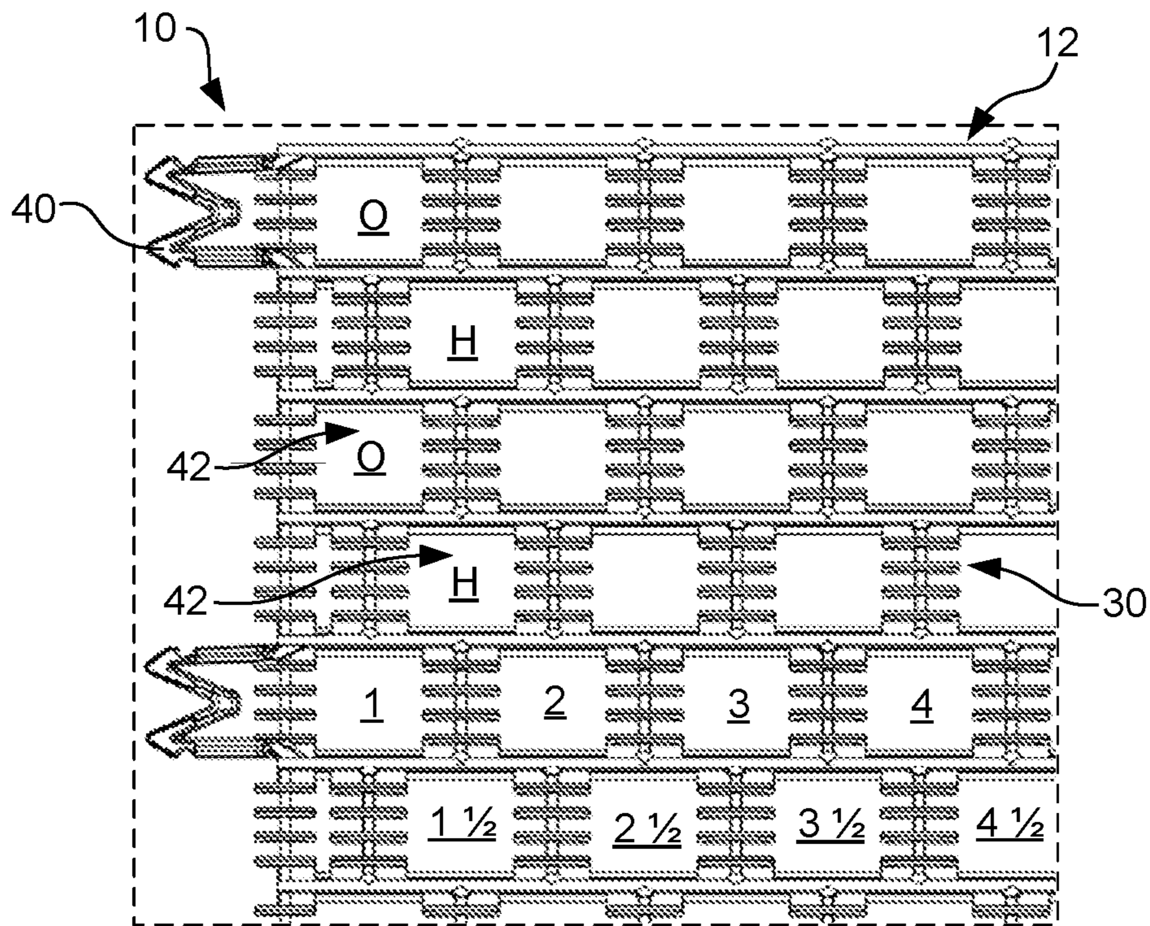
FIG. 6B
