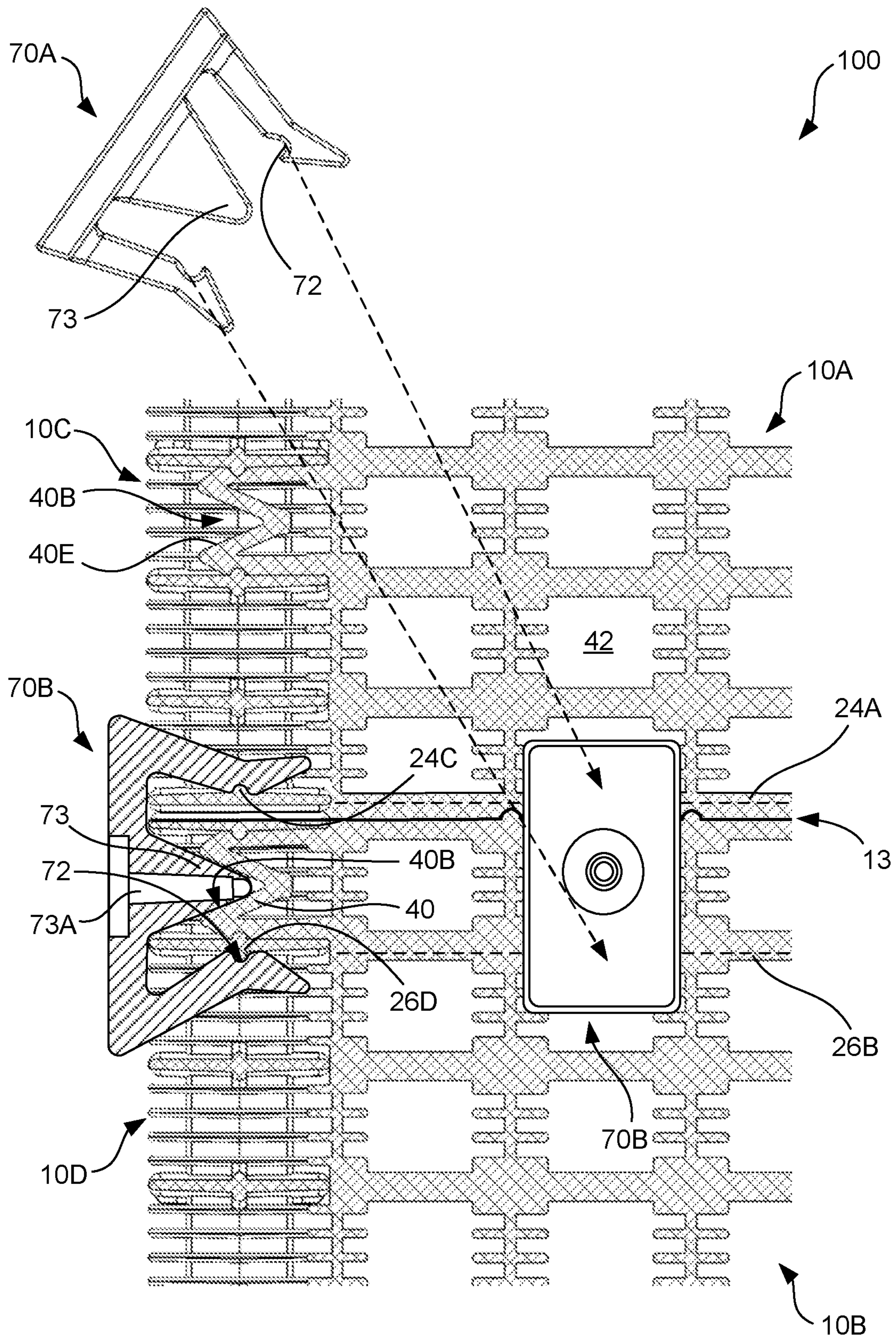
FIG. 26
