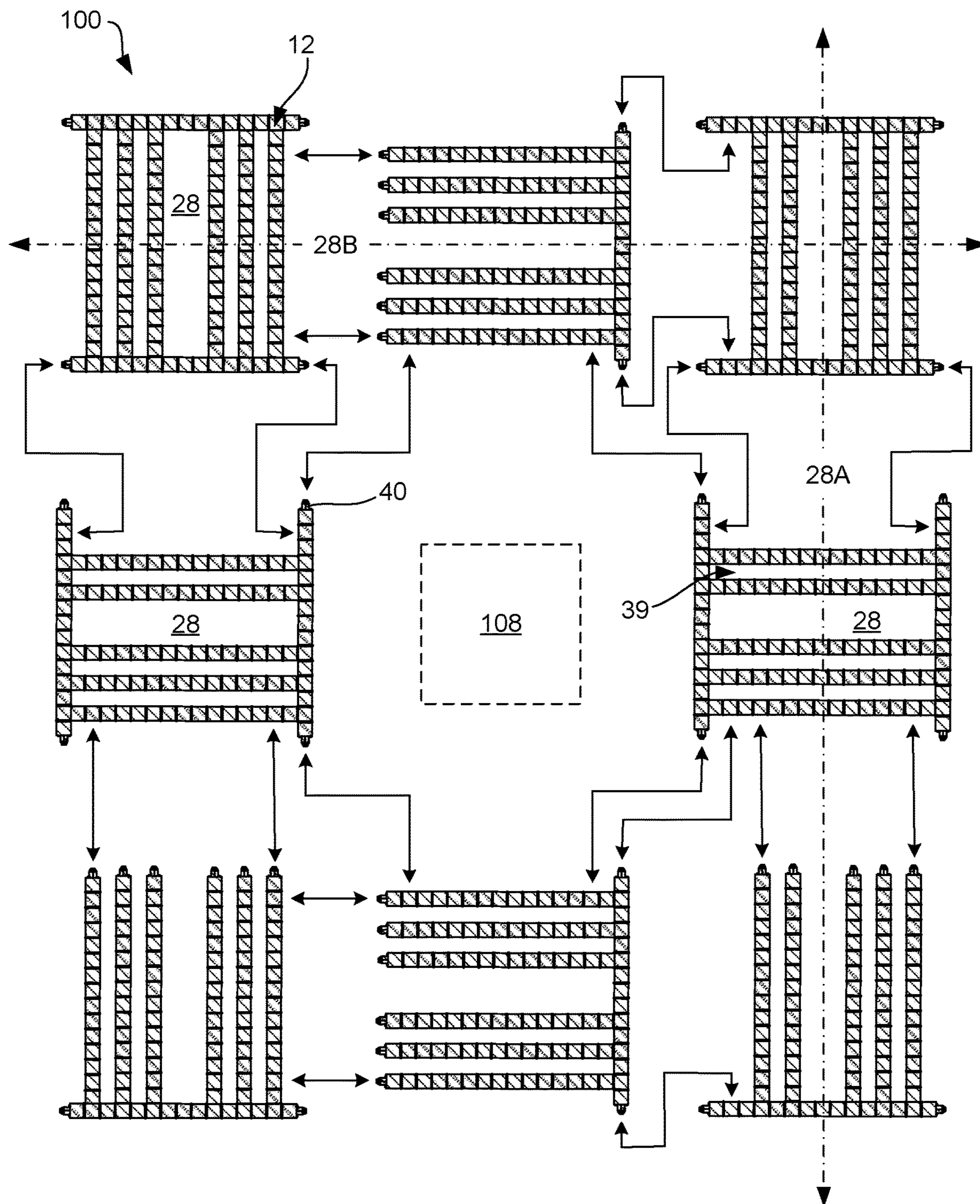
FIG. 12E
