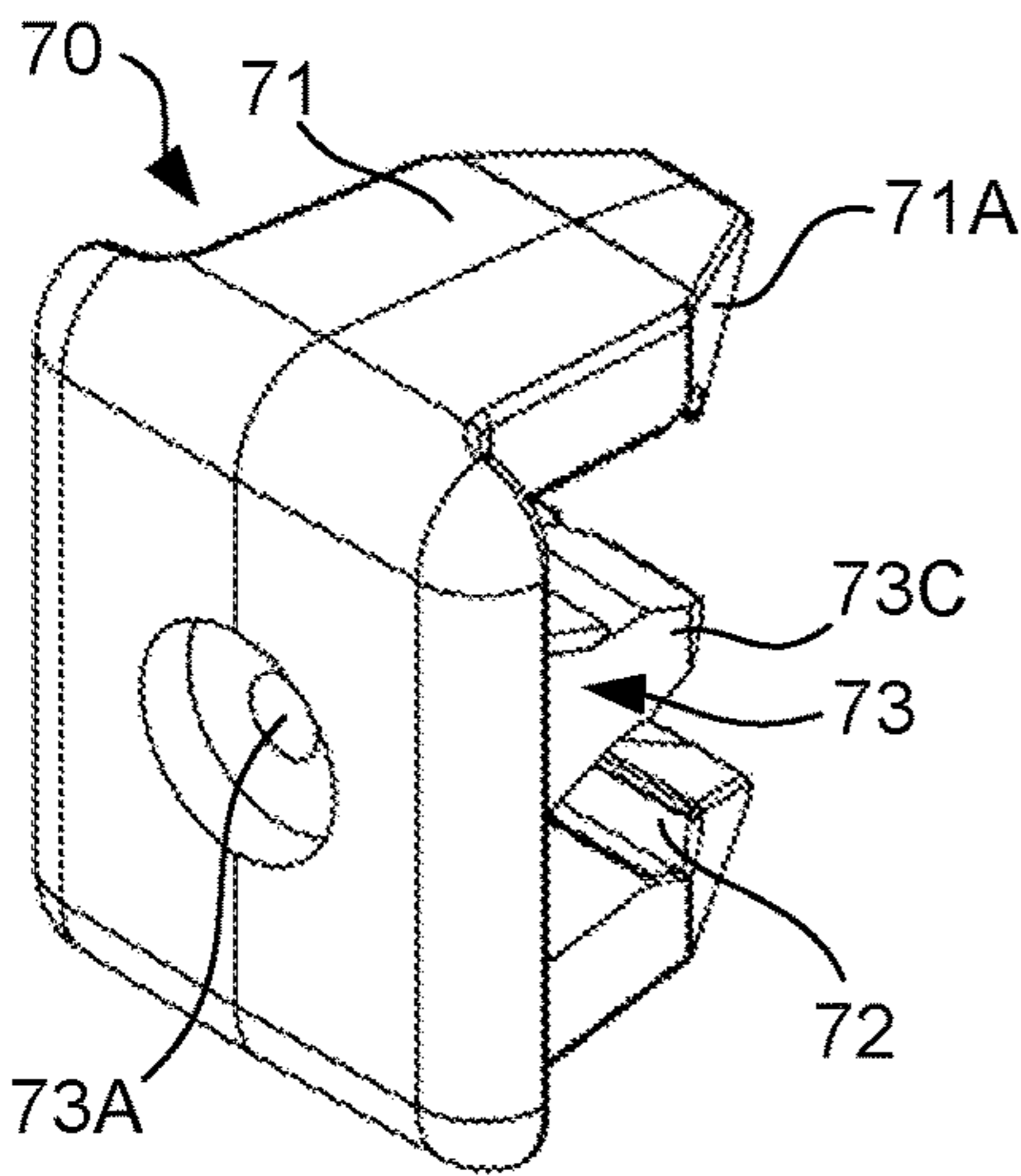
FIG. 32E
