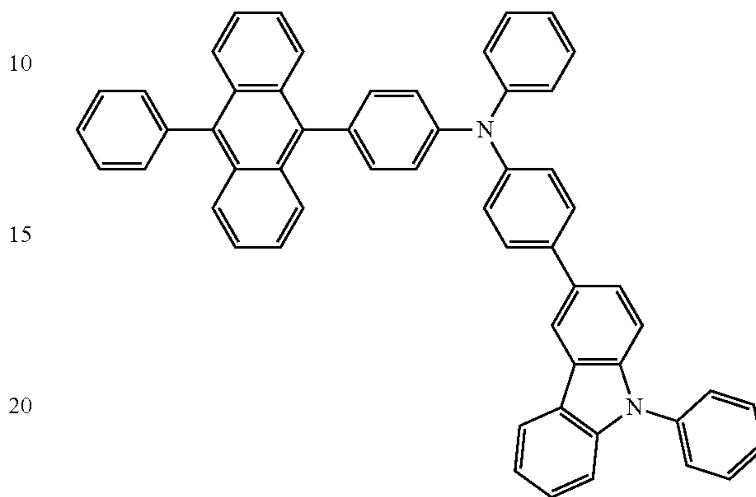
PCBAPA
