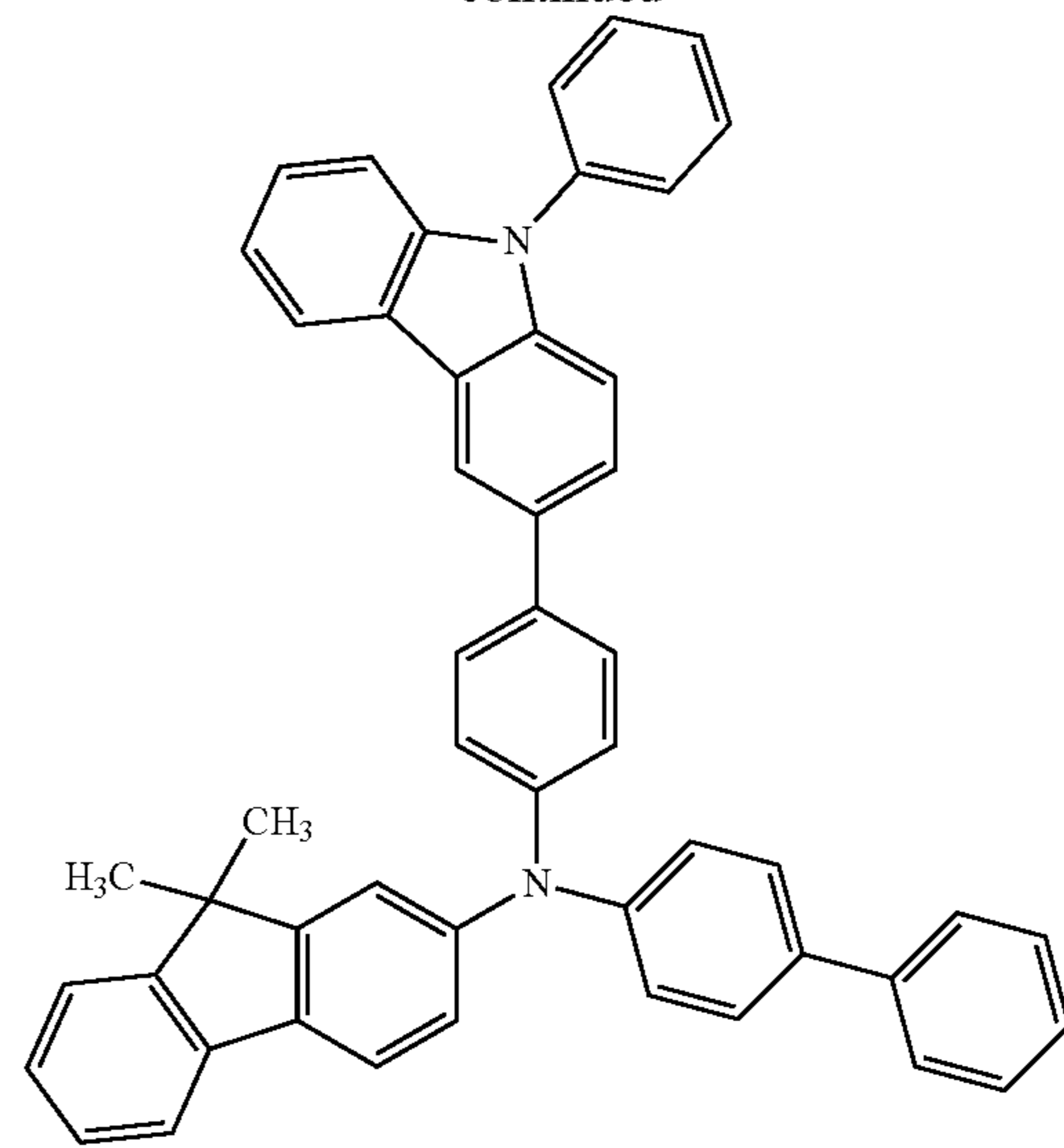
PCBBiF
