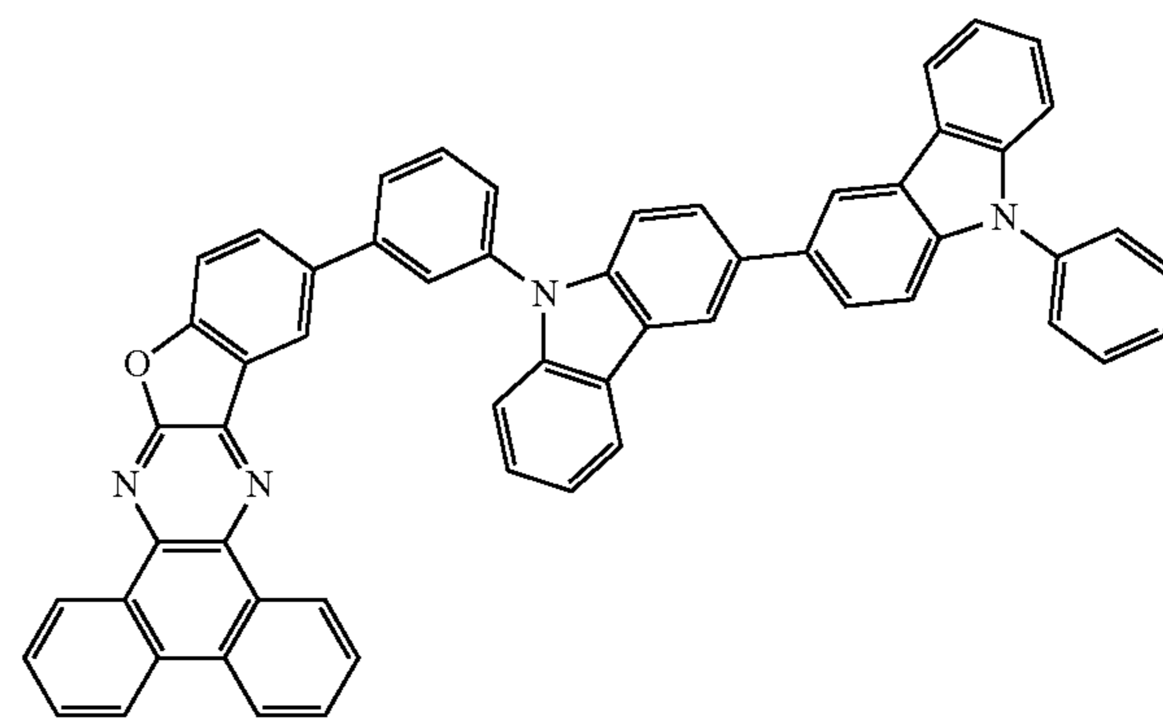
13mPCCzPBfdbq
