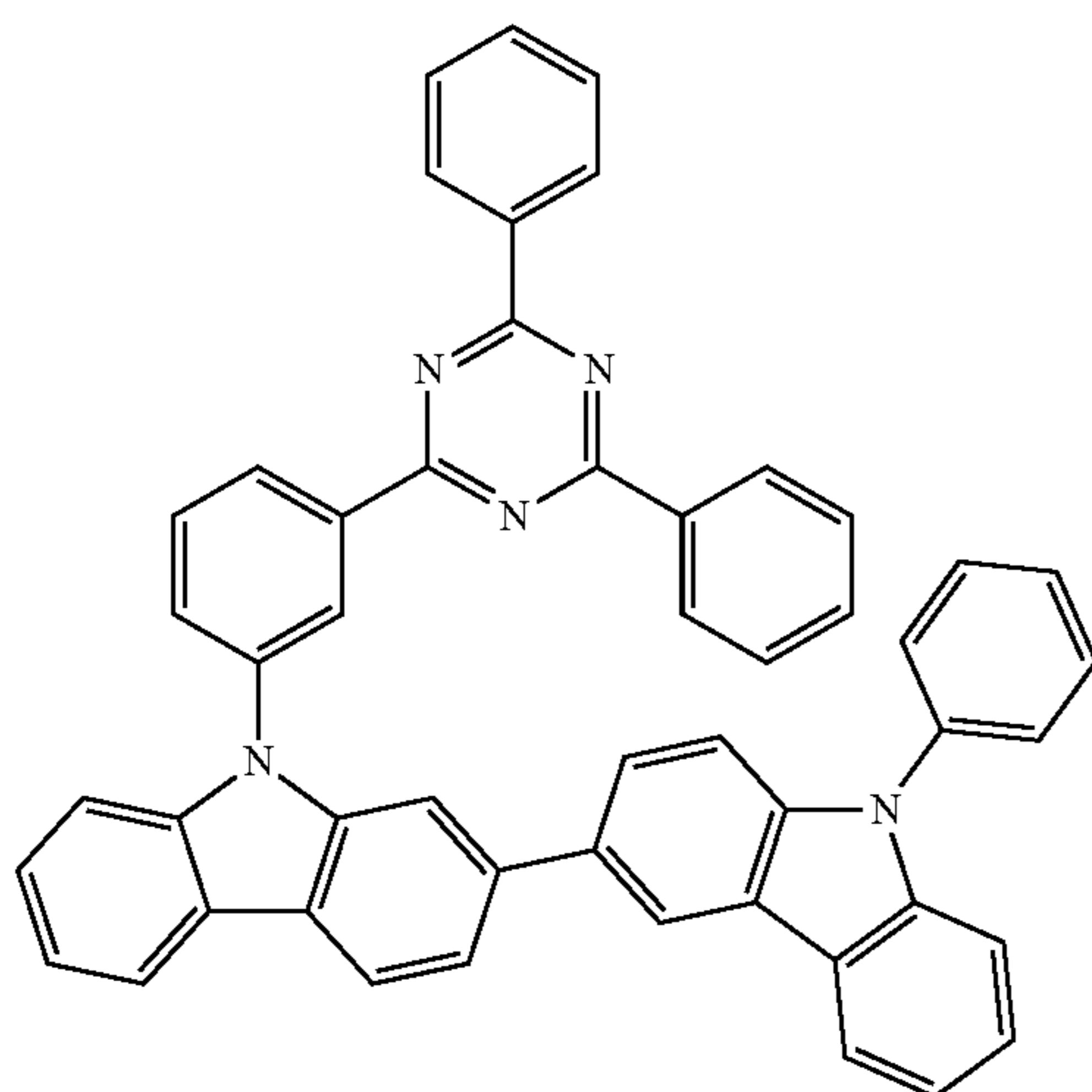
mPCCzPTzn-02
